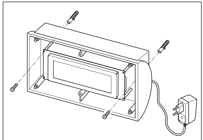
Abb. 5.2 VPI-Display montieren
