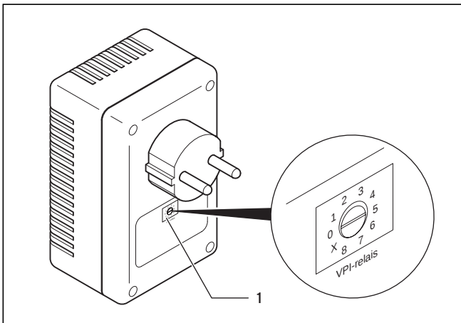
Abb. 5.4 VPI-Display Funkrelais
