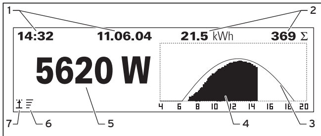
Abb. 4.4 Display 1
