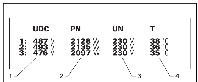
Abb. 4.8 Display 5
