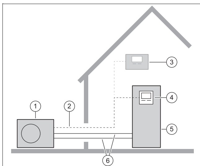
1 Außeneinheit 2 eBUS-Leitung
