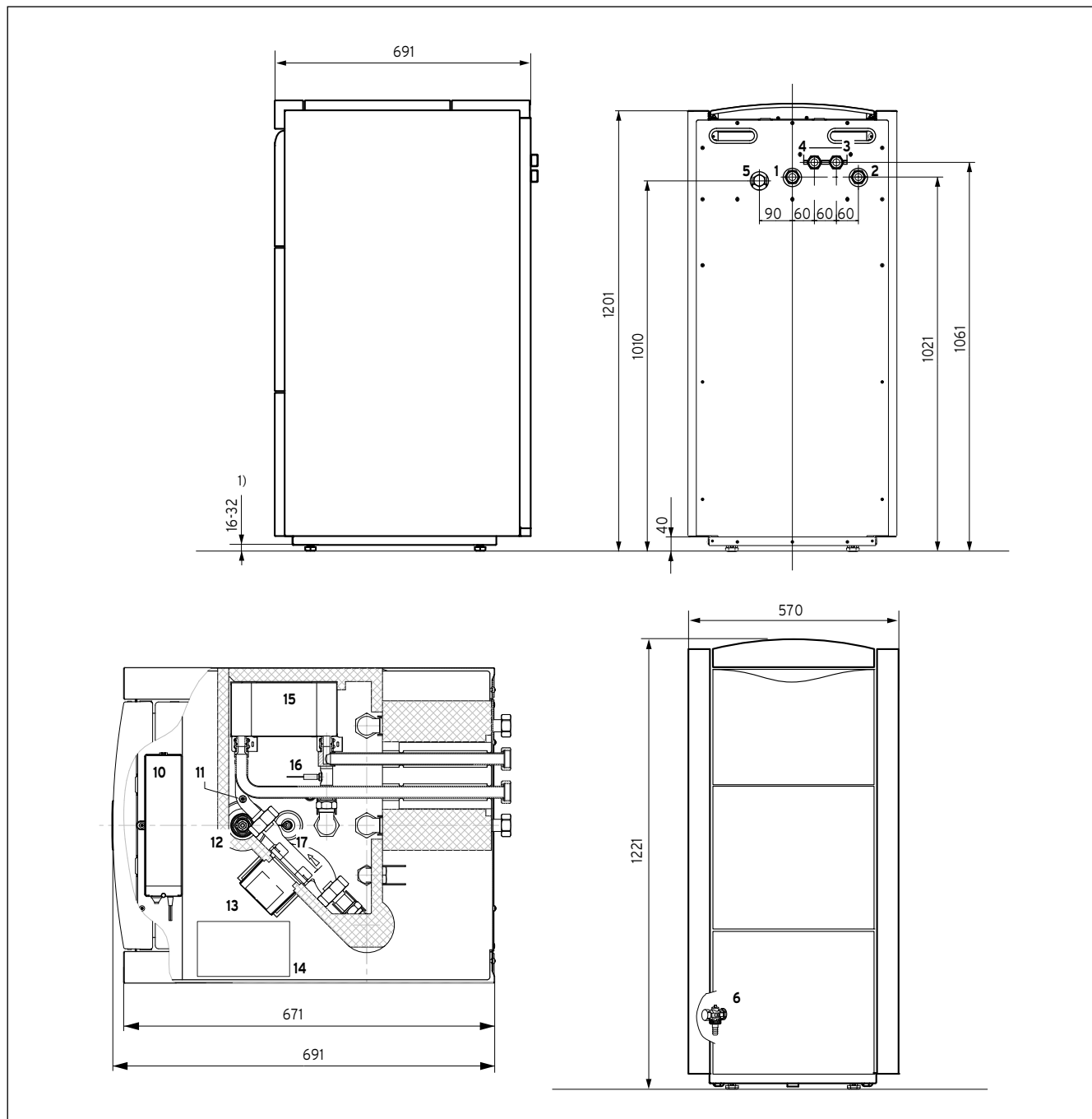
Abb. 5.2 Maßzeichnung
