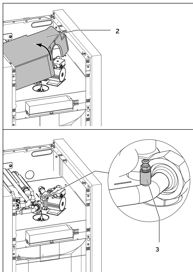
Fig. 6.2 Udluftning på brugsvandssiden
