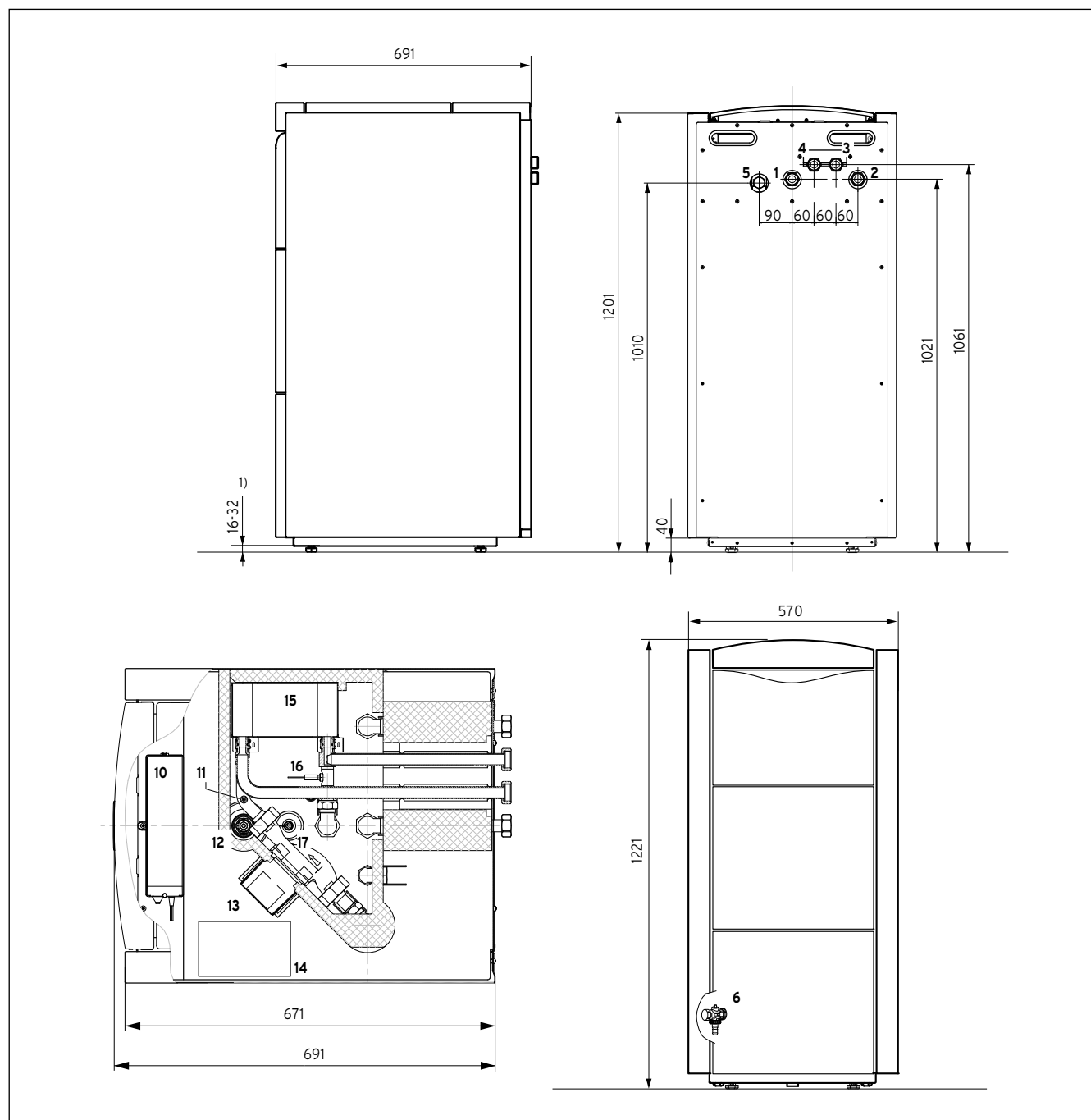
Fig. 5.2 Disegno quotato
