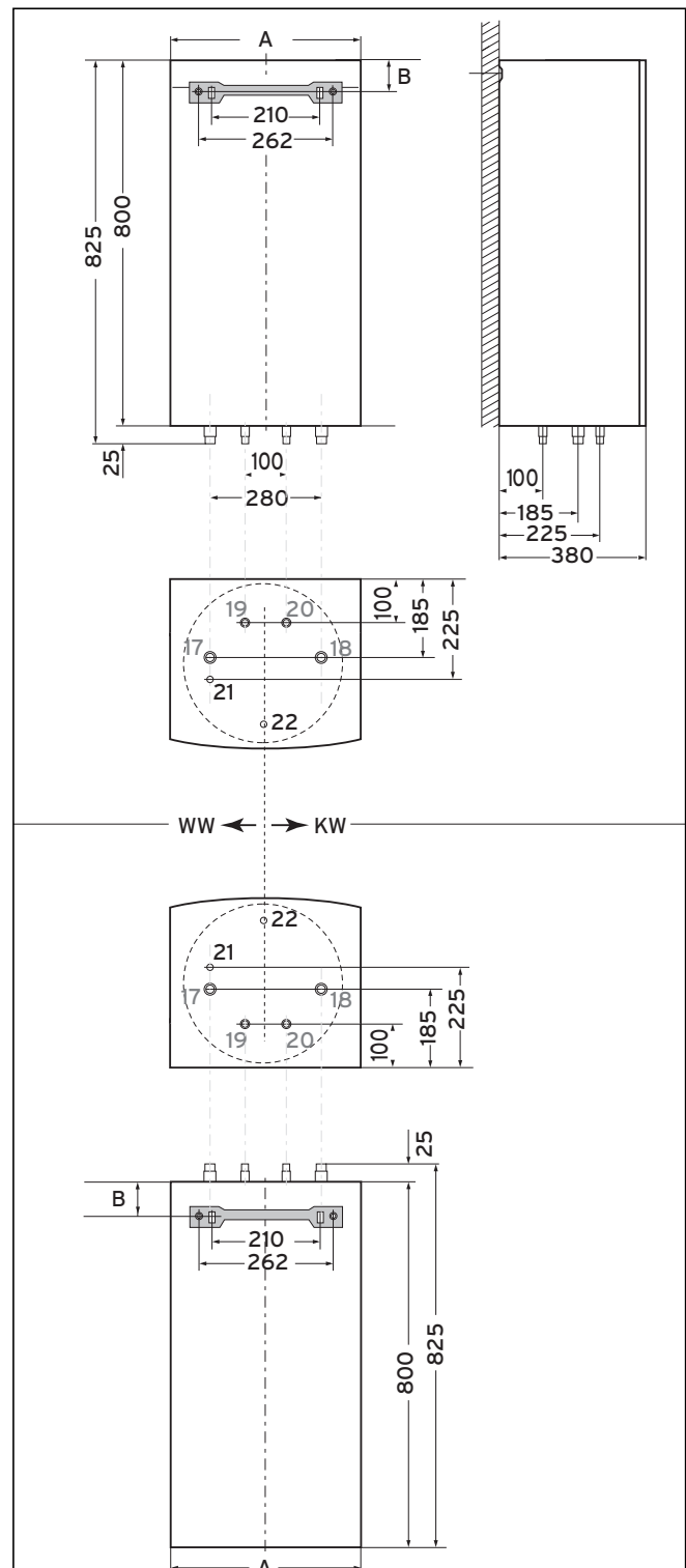
Abb. 4.1 Abmessungen bei Montage neben und unter dem Heizgerät VIH CB 70 und VIH CT 70
