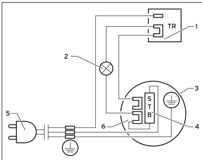
Abb. 4.8 Schaltplan
