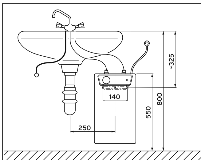
Fig. 4.3 Exemple d'installation VEN 10/5 U
