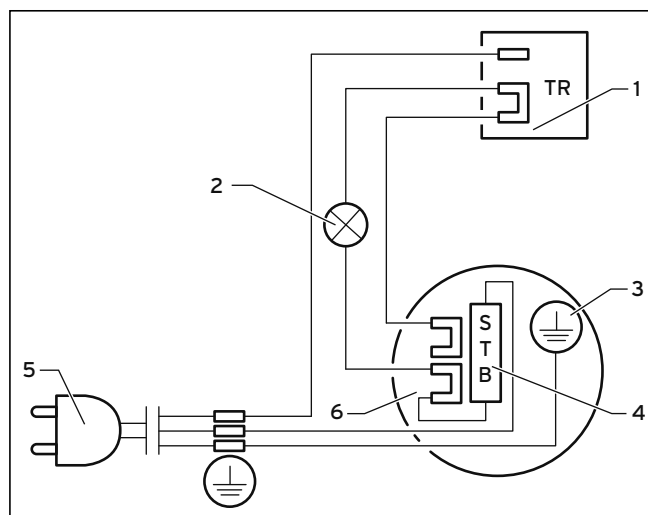
Fig. 4.8 Schéma électrique
