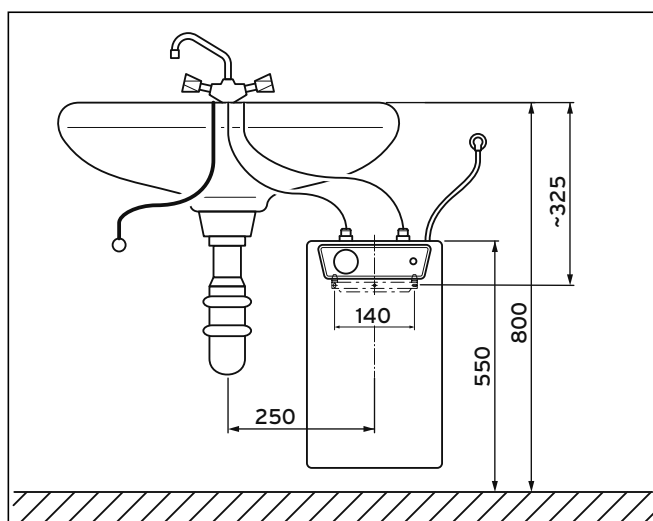
Afb. 4.3 Installatievoorbeeld VEN 10/5 U
