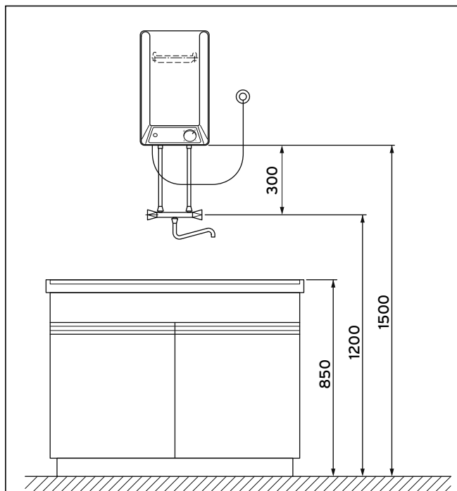
Fig. 4.5 Exemple d'installation VEN 10/5 O
