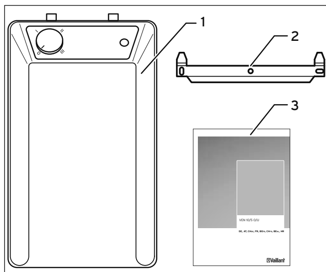
Fig. 4.1 Contenu de la livraison VEN 10/5 U, appareil sous évier
