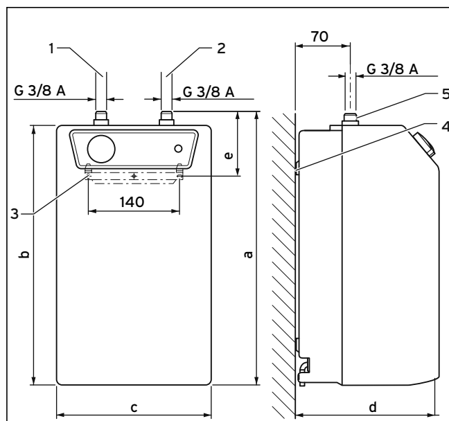
Afb. 4.4 Afmetingen VEN 10/5 U
