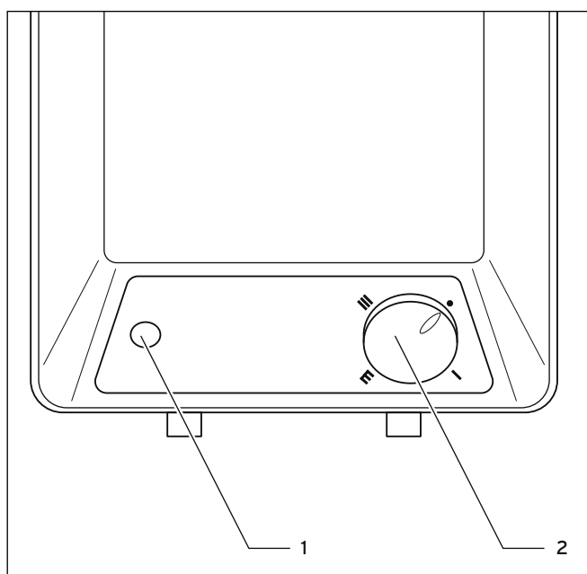
Afb. 5.2 Bedieningselementen bovenbouwtoestel
