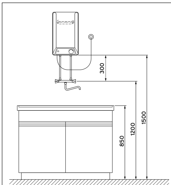
Afb. 4.5 Installatievoorbeeld VEN 10/5 O
