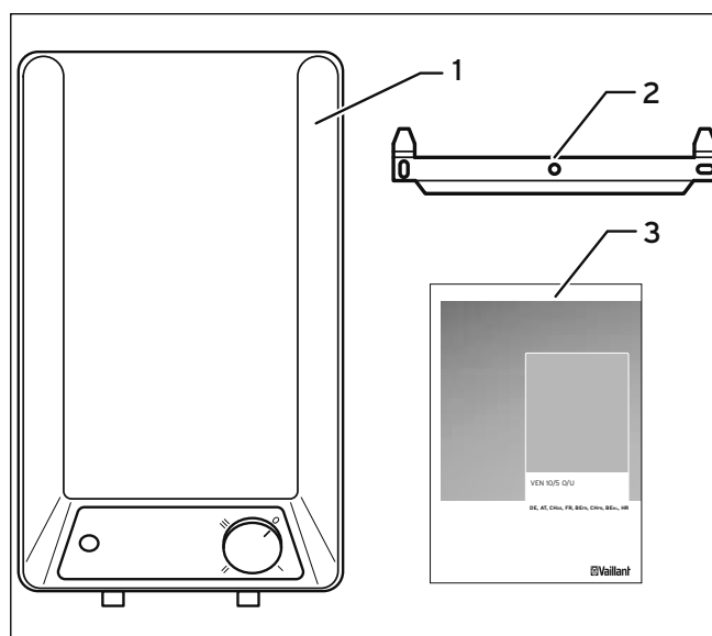
Afb. 4.2 Leveringsomvang VEN 10/5 O bovenbouwtoestel
