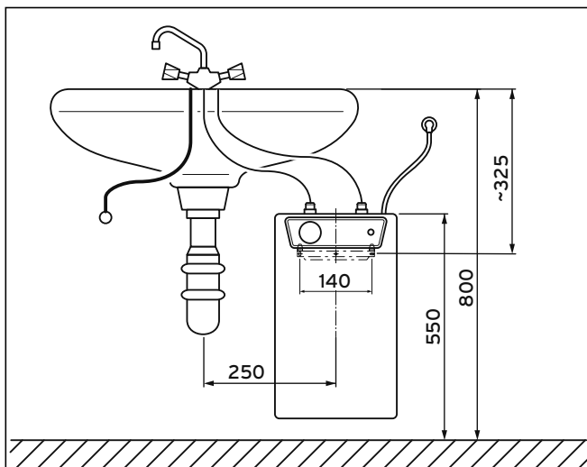
Abb. 4.3 Installationsbeispiel VEN 10/5 U
