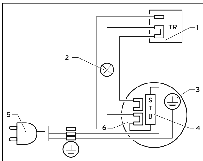
Afb. 4.8 Schakelschema
