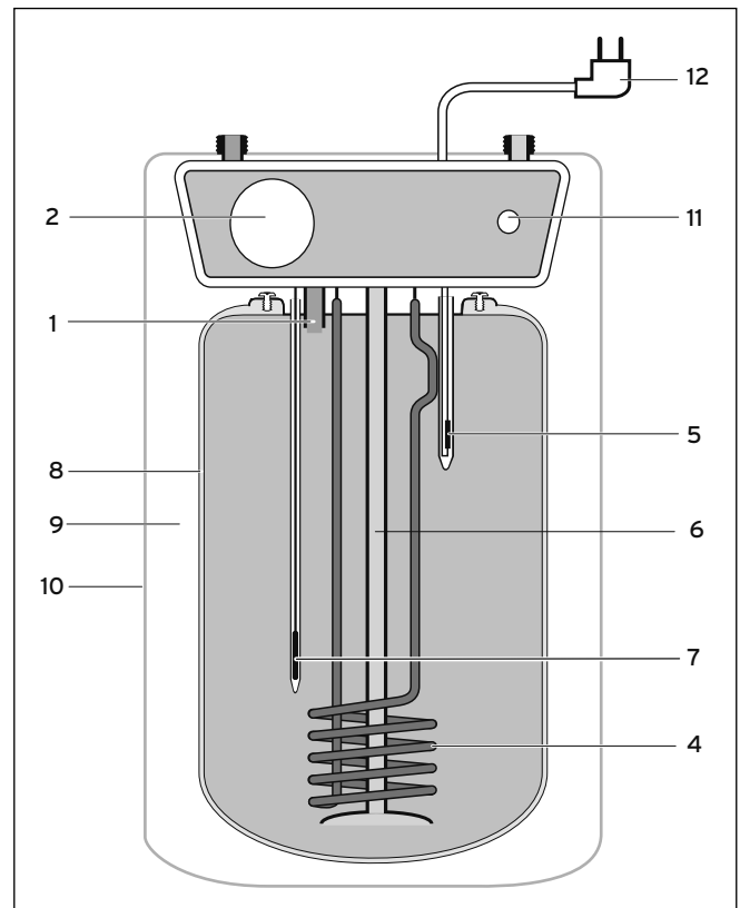
Abb 3.1 Funktionsschema VEN U
