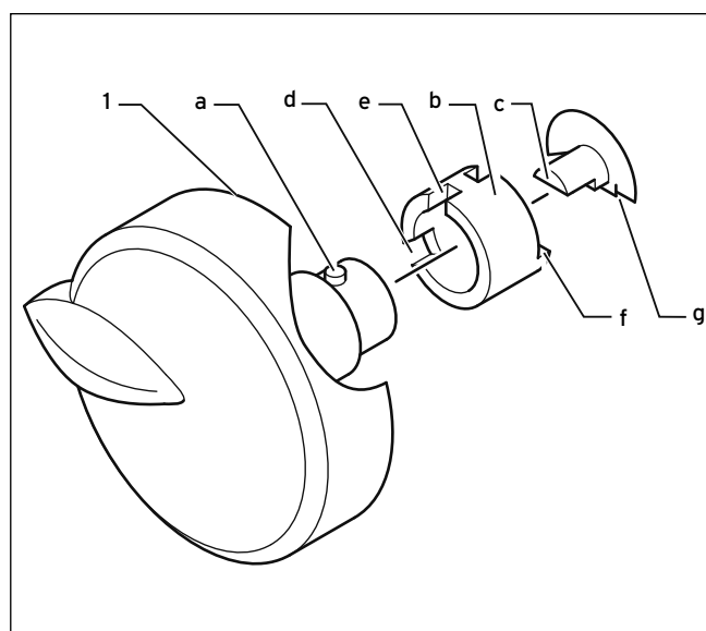
Afb. 5.3 Temperatuurkeuzeknop
