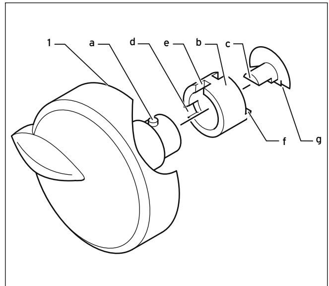
Abb. 5.3 Temperaturwähler
