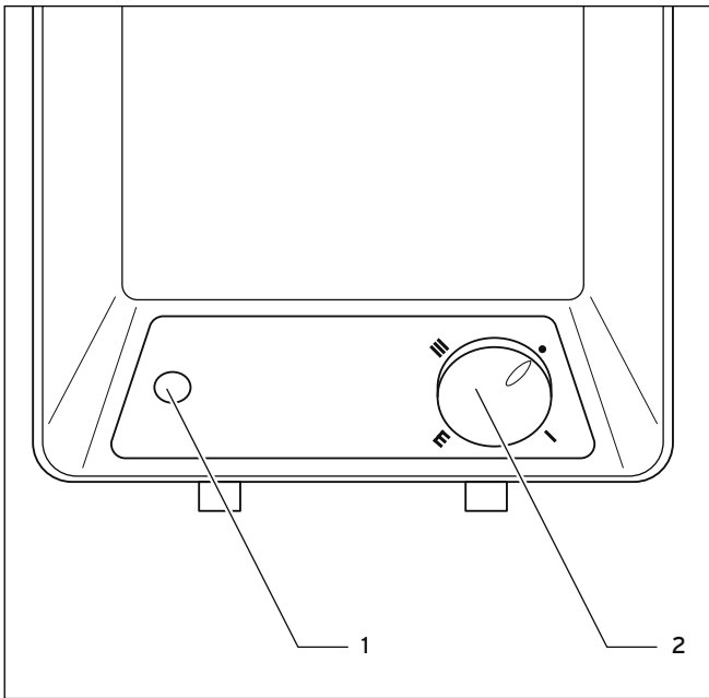
Abb. 7.2 Bedienelemente Übertischgerät
