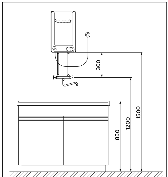
Abb. 4.5 Installationsbeispiel VEN 10/5 O
