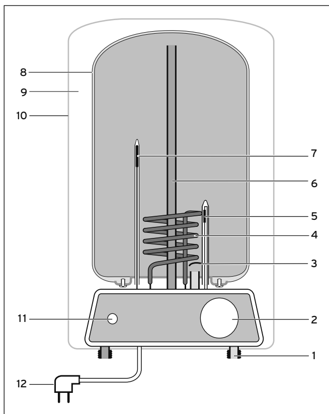
Afb 3.2 Functieschema VEN 0
