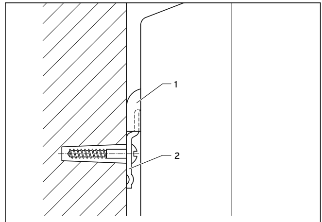
Abb. 4.7 Elektro-Warmwasserspeicher aufhängen
