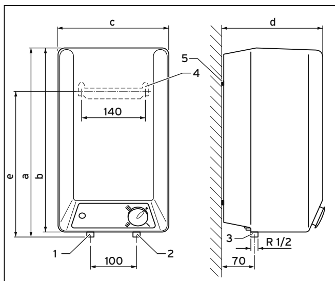
Fig. 4.6 Dimensions VEN 10/5 O
