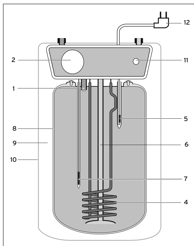
SI 3.1 Funkcionalna shema VEN U
