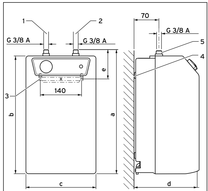
Abb. 4.4 Abmessungen VEN 10/5 U
