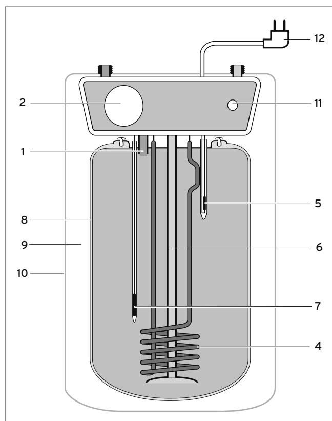
Afb 3.1 Functieschema VEN U
