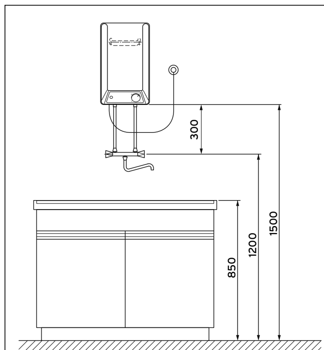
Sl. 4.5 Primjer instalacije VEN 10/5 0
