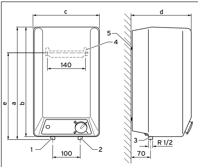
Abb. 4.6 Abmessungen VEN 10/5 O
