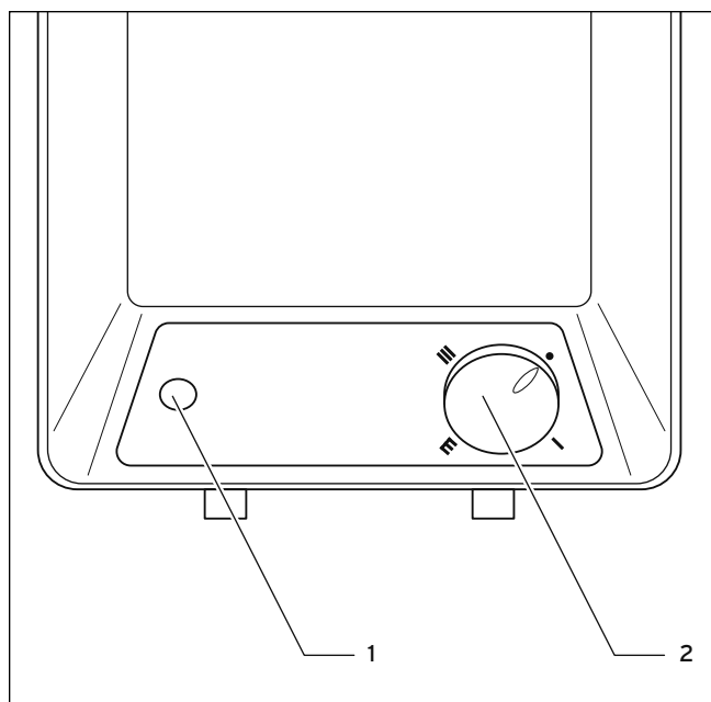
Fig. 7.2 Éléments de commande, appareil monté au-dessus du plan de travail
