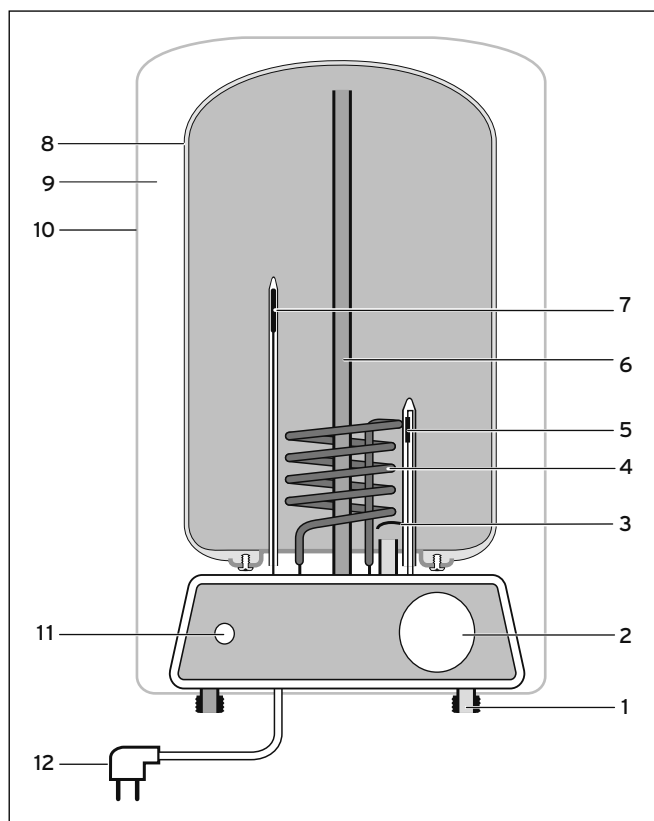
Fig. 3.2 Schéma de fonctionnement VEN O
