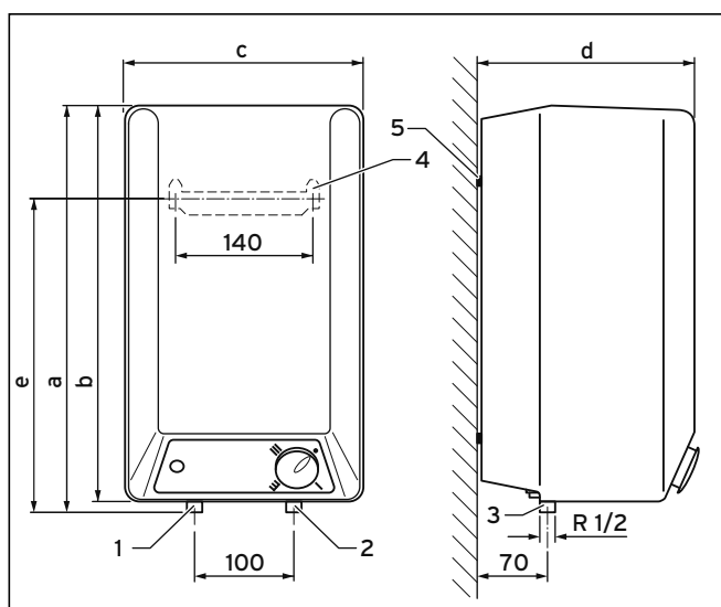
Afb. 4.6 Afmetingen VEN 10/5 O
