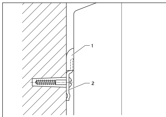
Afb. 4.7 Elektrisch boiler ophangen
