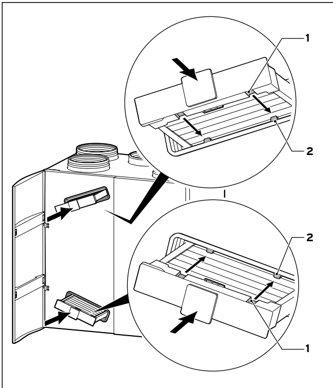
7.2 Filter zurückschieben
