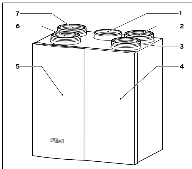
3.3 Lüftungsgerät
