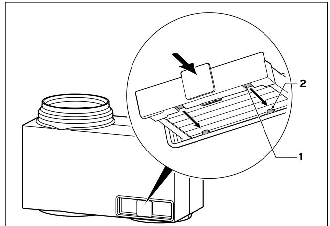
7.5 Bypass-Filter zurückschieben
