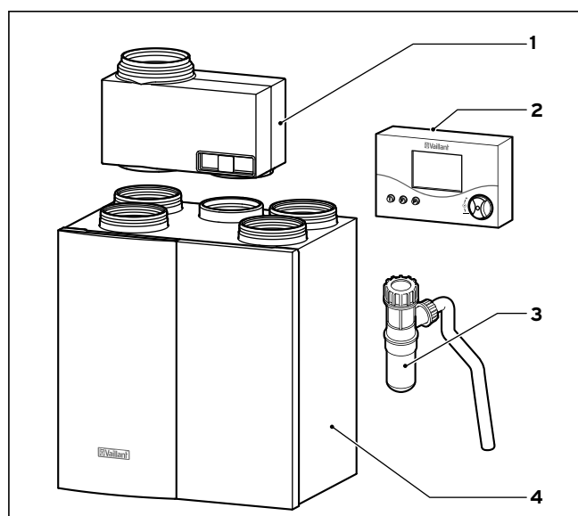
3.2 Wohnraumlüftungsgerät recoVAIR
