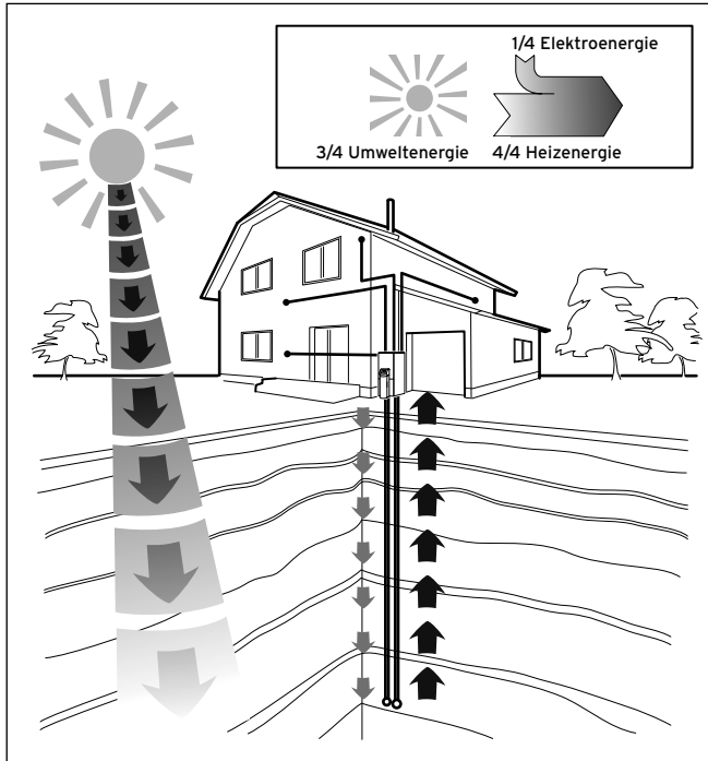
3.2 Nutzung der Wärmequelle Erdwärme
