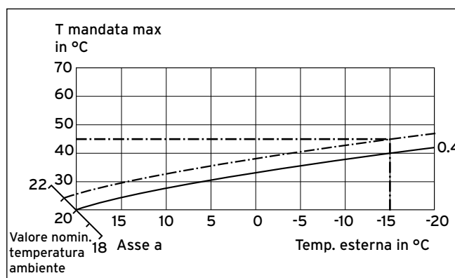
10.2 Spostamento in parallelo della curva di riscaldamento
