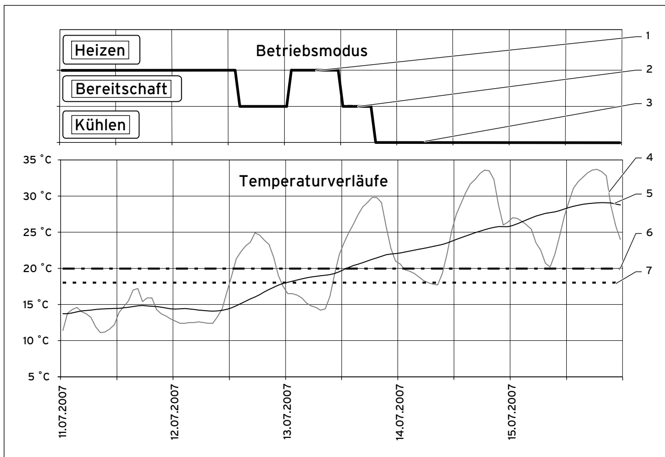
3.5 Beispiel für eine außentemperaturabhängige Umschaltung zwischen Heizen und Kühlen
