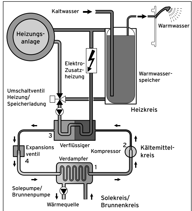
3.3 Funktionsweise der Wärmepumpe
