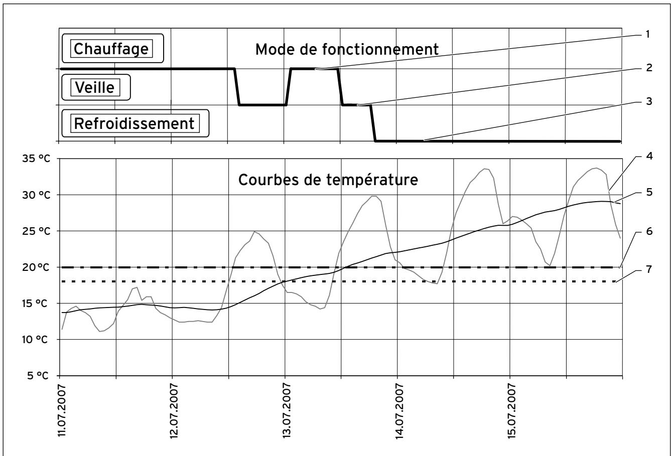
3.5 Exemple d'un passage dépendant de la température extérieure entre le mode de chauffage et celui de refroidissement
