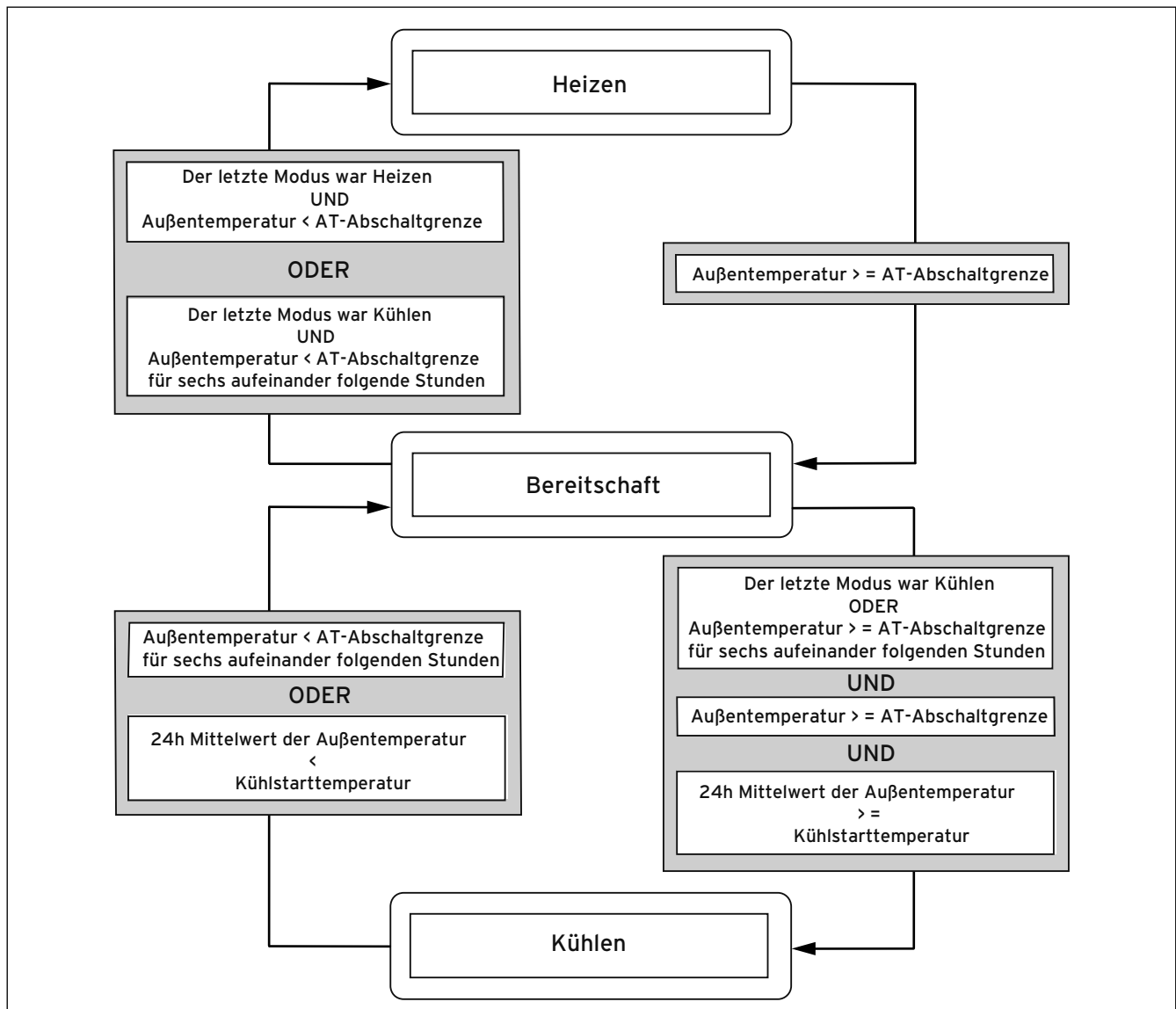
3.4 Übergangsschema
