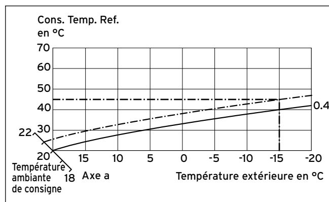
10.2 Déplacement parallèle de la courbe de chauffage
