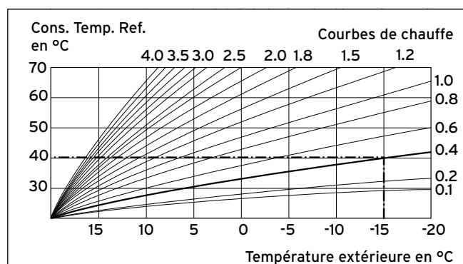
10.1 Diagramme des courbes de chauffage
