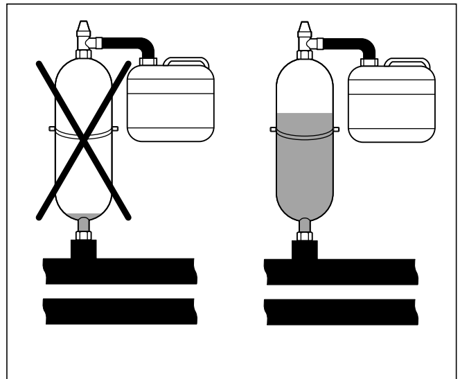
6.1 Niveau d'eau glycolée dans le réservoir de compensation
