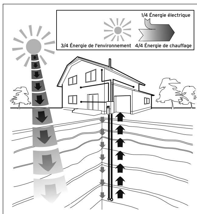
3.2 Exploitation de la source géothermique
