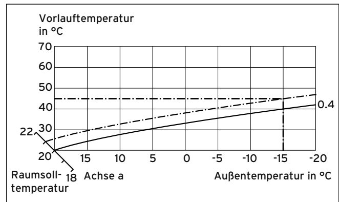
10.2 Parallelverschiebung der Heizkurve
