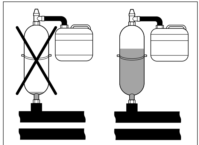
6.1 Füllstand des Sole-Ausgleichsbehälters
