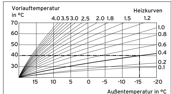
10.1 Diagramm Heizkurven
