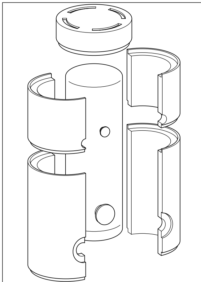
5.11 Rimozione dell'isolamento
