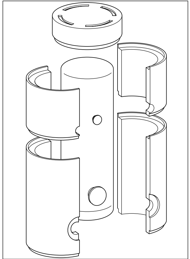
Afb. 5.11 Isolatie wegnemen
