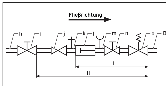
Abb. 6.1 Anschlussplan
