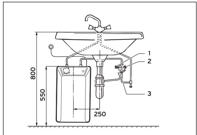
Abb. 5.3 Montagebeispiel, Maße in mm
