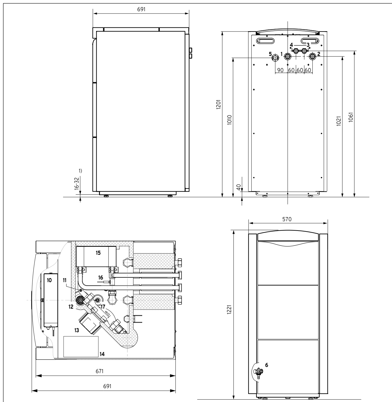
Fig. 5.2 Plan coté
