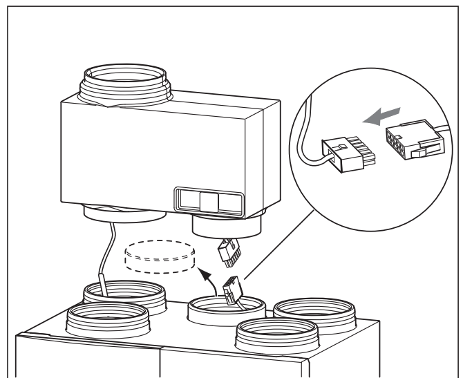
Abb. 4.10 Elektrischer Anschluss Bypass
