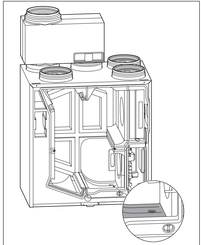
Abb. 6.2 Kondenswasserabfluss
