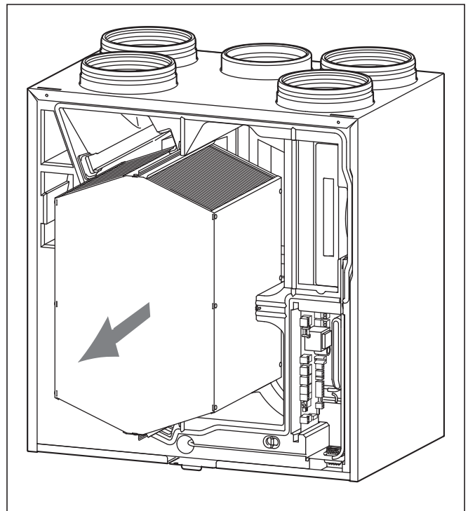
Abb. 6.1 Wärmetauscher ausbauen
