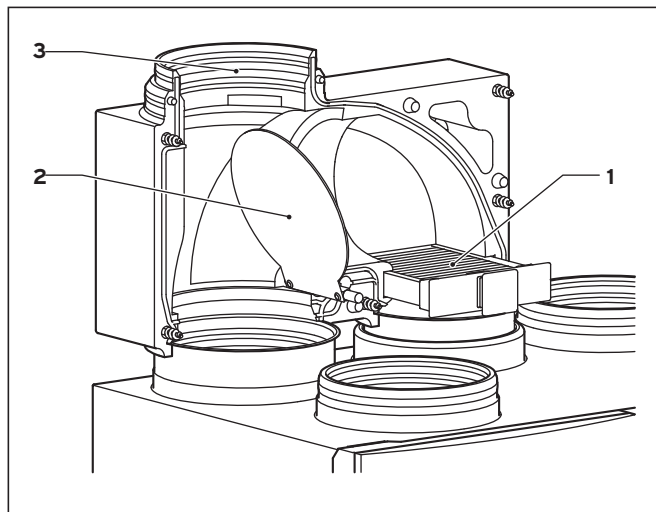
Abb. 4.3 Aufbau Bypass
