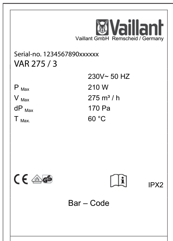
Abb. 1.1 Typenschild
