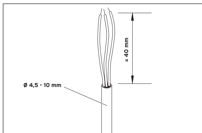
Abb. 4.16 Kabelisolation entfernen
