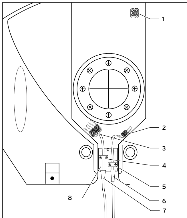
Рис. 8.1 Клеммная коробка
