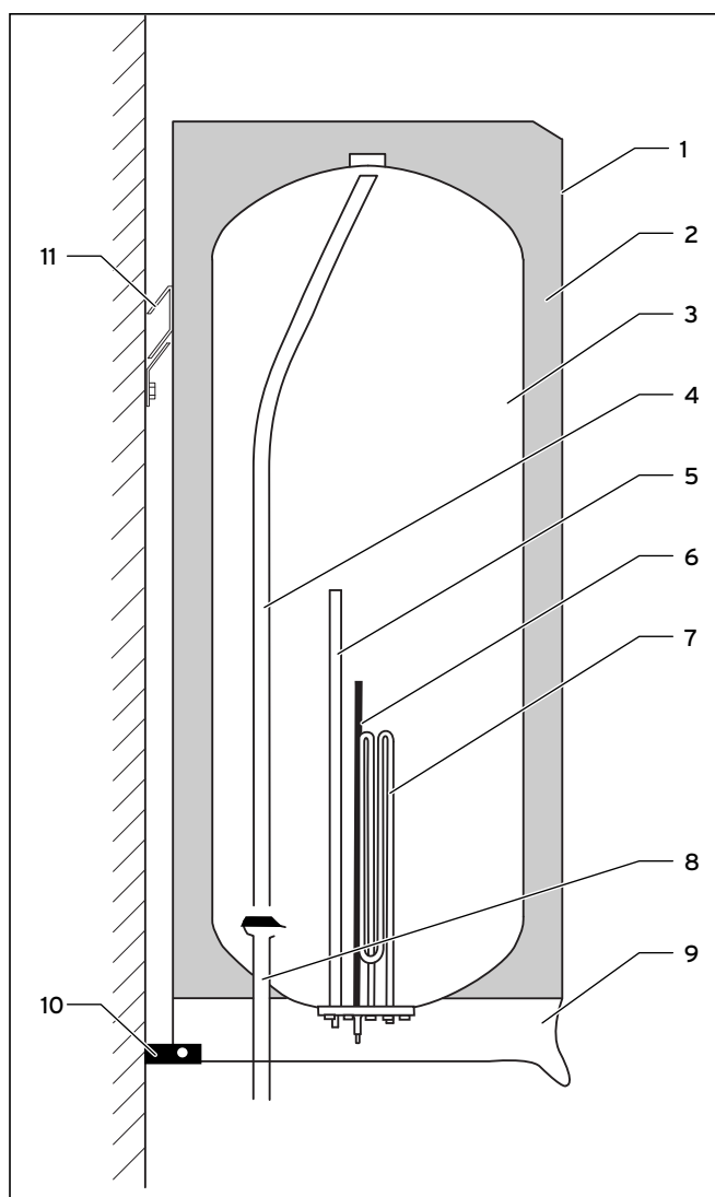
Abb. 2.2 Aufbau
