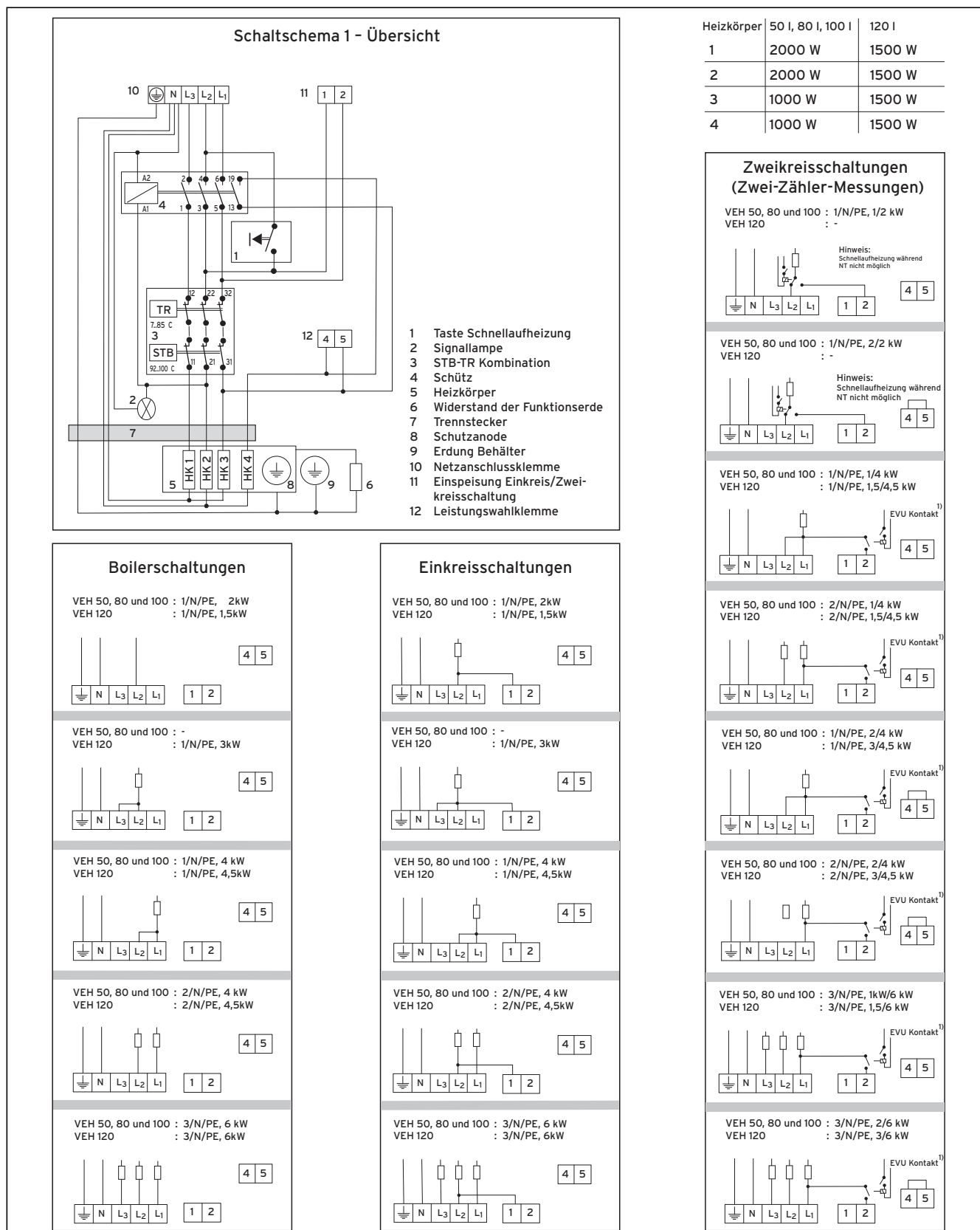
Abb. 8.2 Schaltschema (VEH exclusiv/pro)
