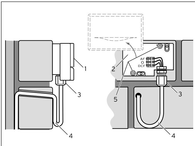
Abb. 4.3 Montage des Außenfühlers VRC 9535
