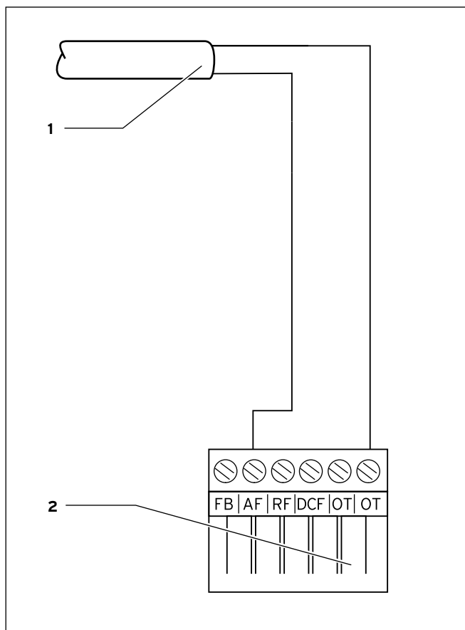
Abb. 5.2 Elektrischer Anschluss des Außenfühlers VRC 693
