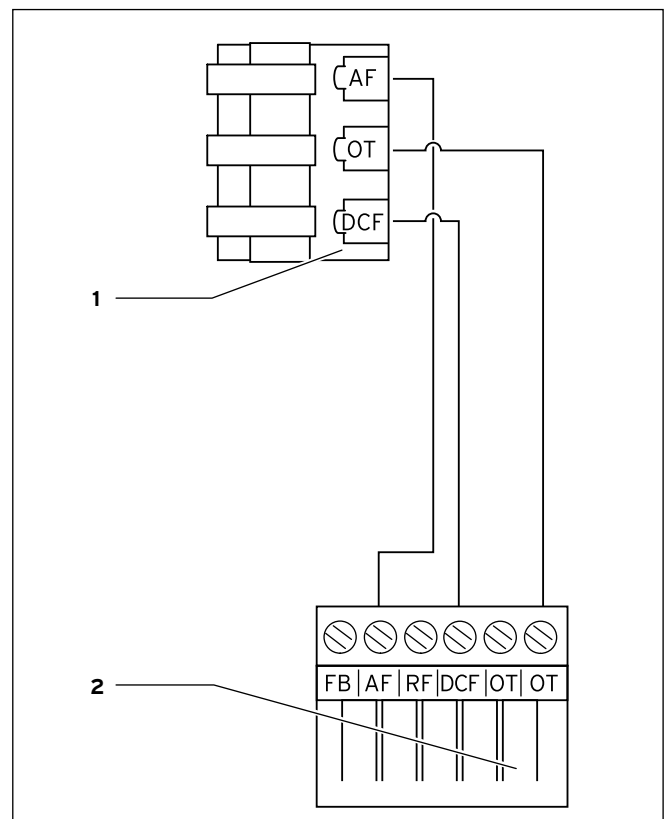
Abb. 5.3 Elektrischer Anschluss des Außenfühlers VRC 9535
