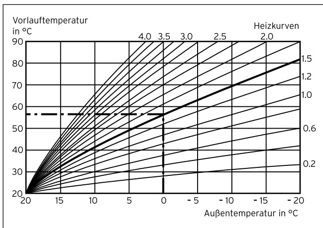
Abb. G.1 Diagramm mit Heizkurven für eine Raumsolltemperatur von 20 °C
