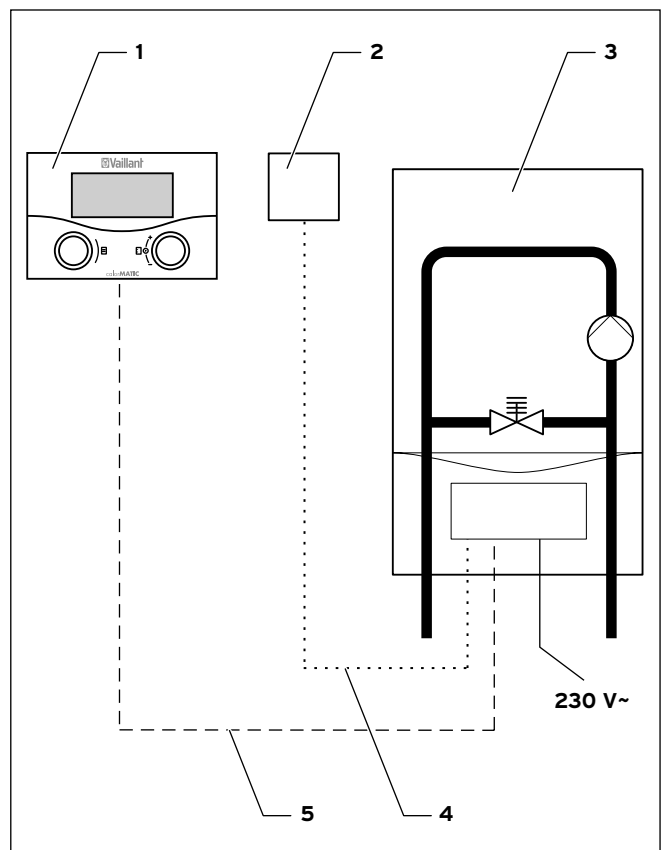
Abb. 2.1 Systemschema
