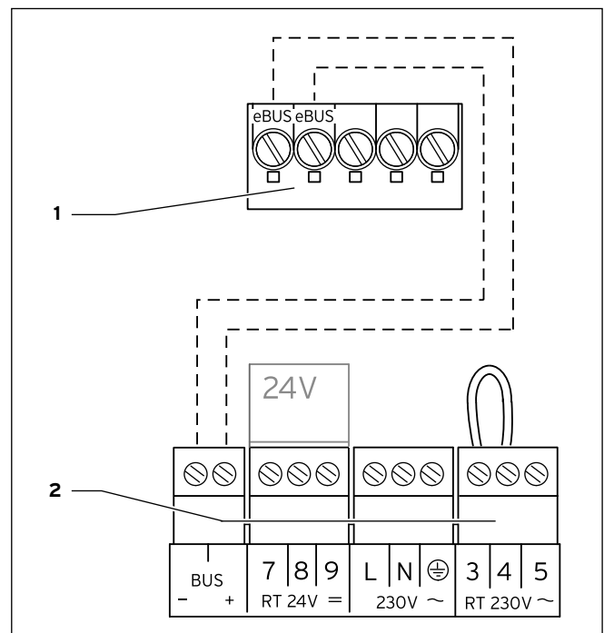
Abb. 5.1 Elektrischer Anschluss des calorMATIC 430
