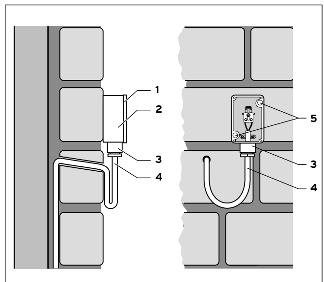
Abb. 4.2 Montage des Außenfühlers VRC 693
