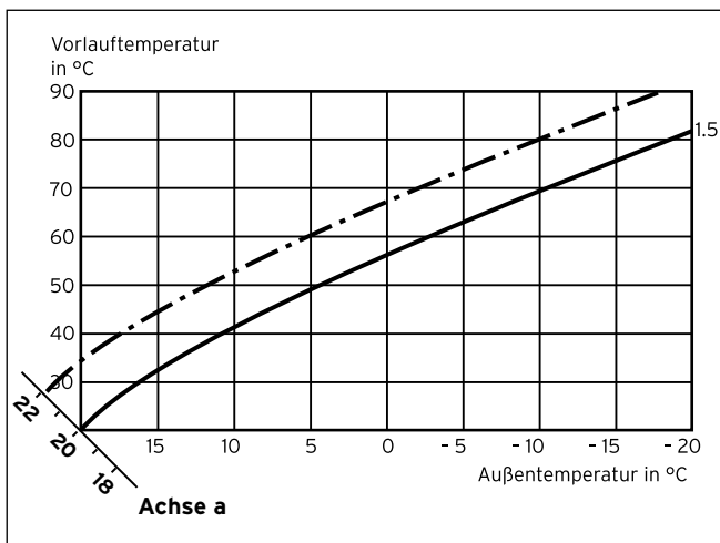
Abb. G.2 Parallelverschiebung der Heizkurve
