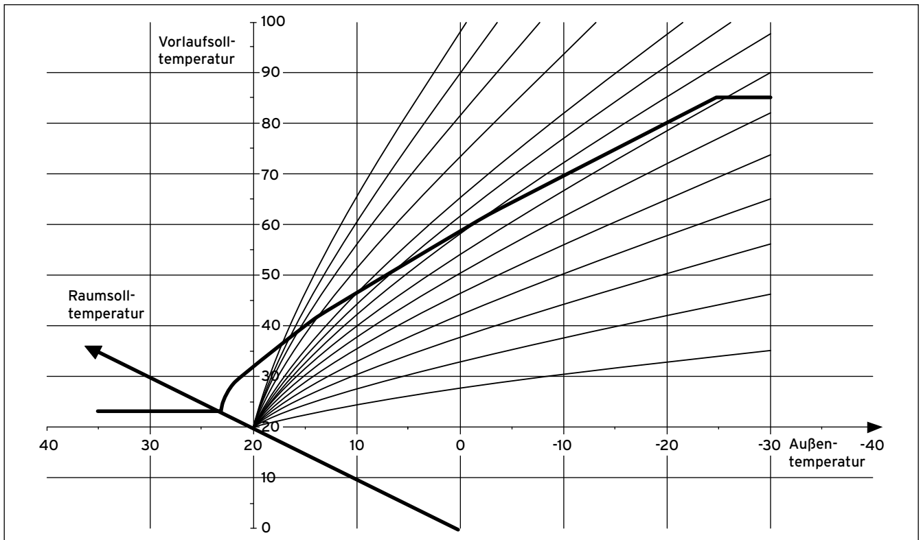
8.35 Heizkurve
