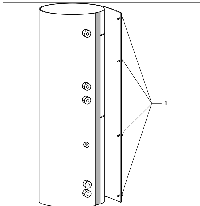
Afb. 5.8 Mantel losmaken
