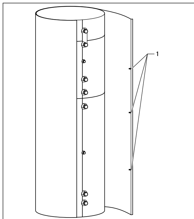
Abb. 5.9 Verkleidungsmantel lösen
