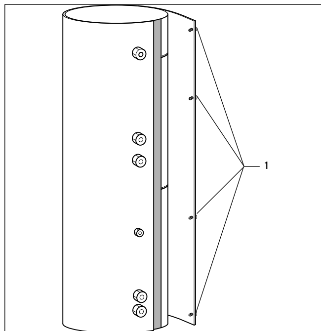
Abb. 5.8 Verkleidungsmantel lösen
