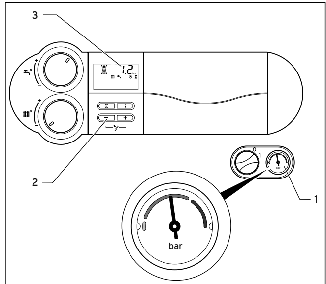
Abb. 4.14 Heizungsanlage füllen
