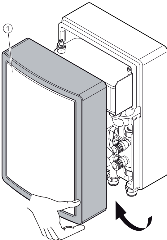
1 Frontverkleidung
