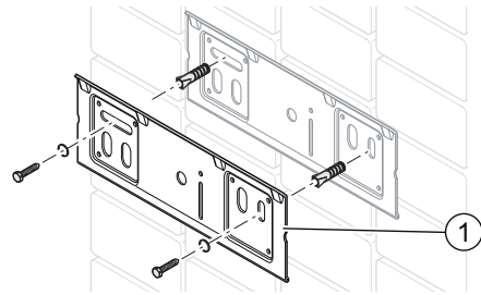
1 Aufhängeleiste
