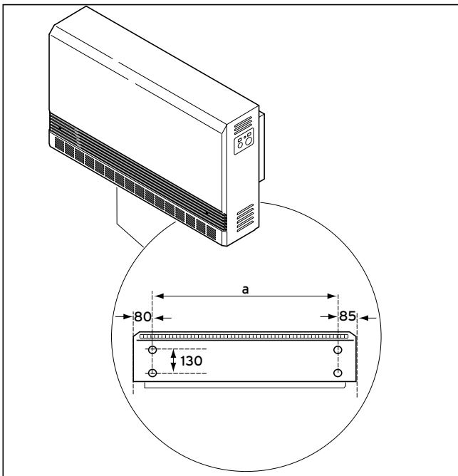
Abb. 4.7 Maße Bodenbefestigung
