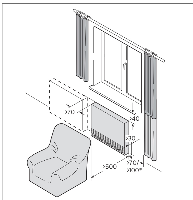
Abb. 2.2 Sicherheitsabstände
