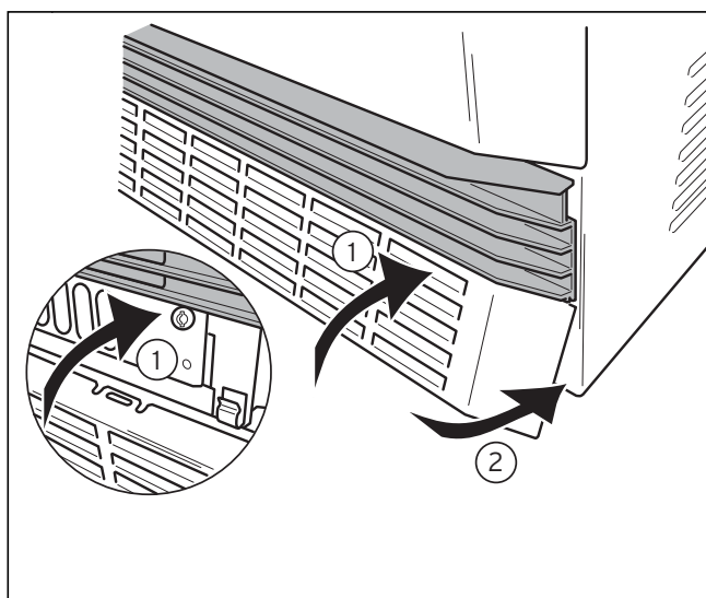
Abb. 4.5 Luftgitter einsetzen
