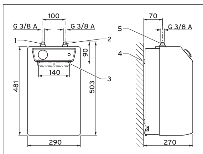
Abb. 5.2 Aufbau des VEH 10/5 U
