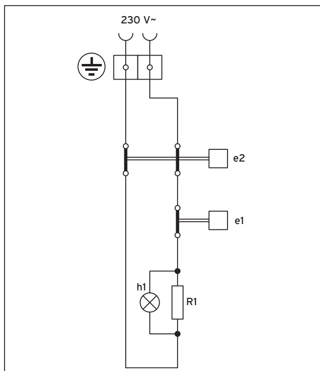
Abb. 6.2 Schaltplan
