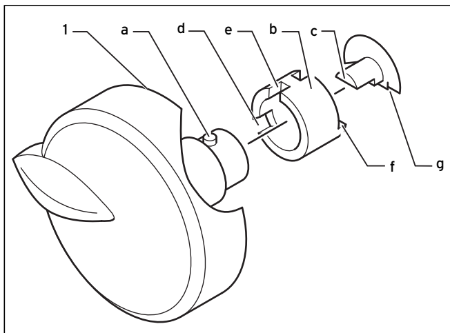
Abb. 7.1 Temperaturwähler
