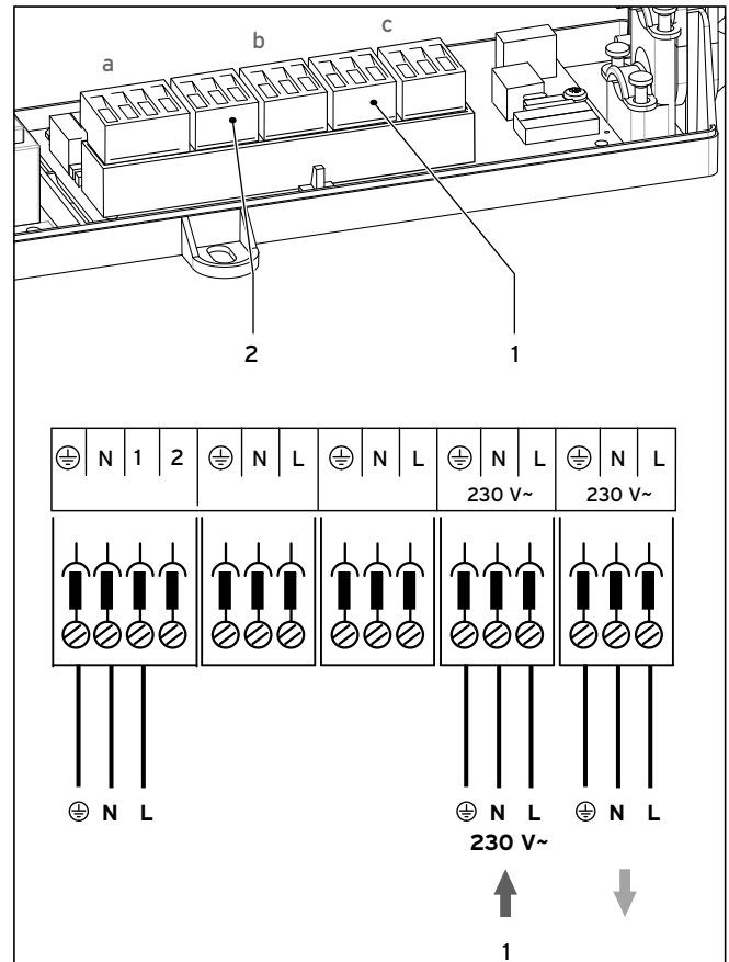
Fig. 5.3 EI-tilslutning på actoSTOR
