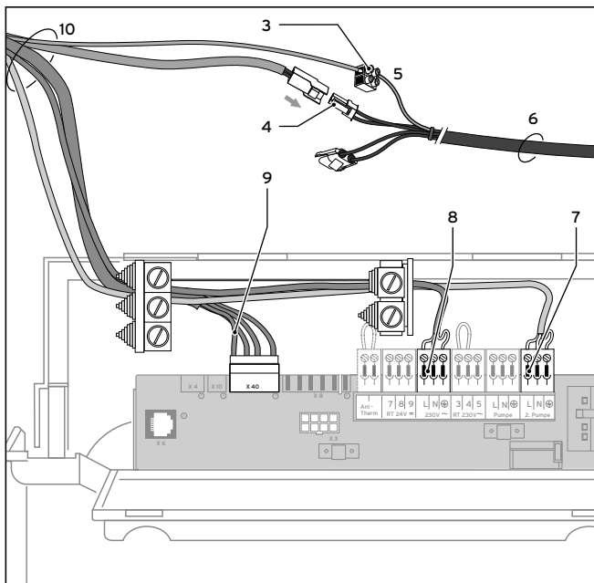
Fig. 5.4 El-tilslutning på ecoVIT/4 og icoVIT VKO 246-7
