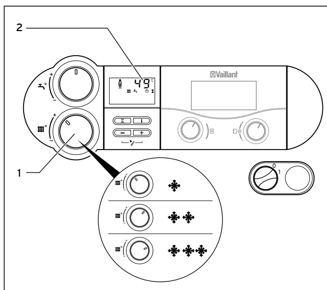
4.6 Vorlauftemperatur-Einstellung ohne Regelgerät
