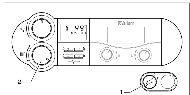
4.7 Vorlauftemperatur-Einstellung bei Einsatz eines Regelgerätes
