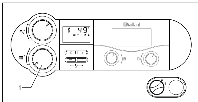
4.8 Heizbetrieb ausschalten (Sommerbetrieb)
