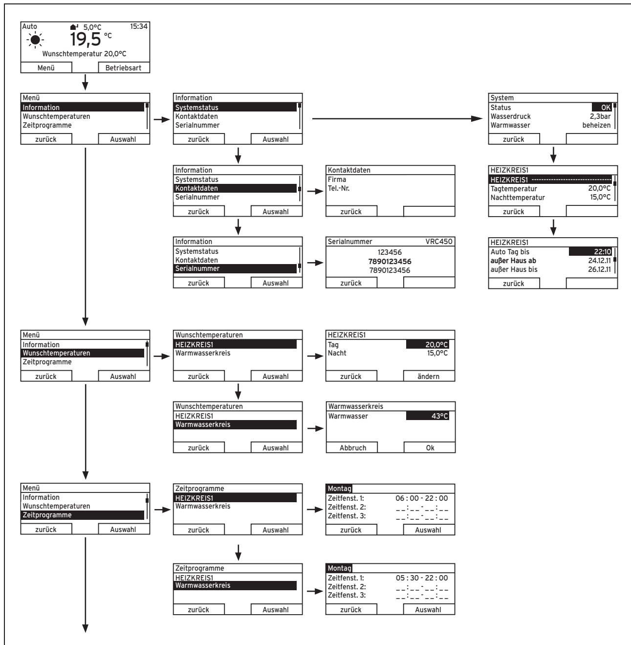
Abb. 4.14: Menüstruktur Teil 1
