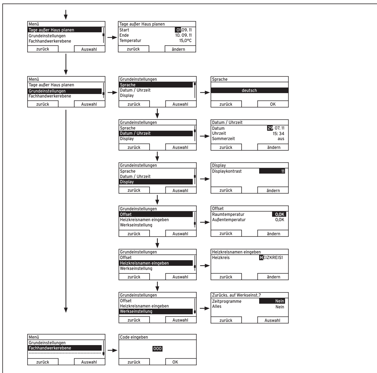
Abb. 4.15: Menüstruktur Teil 2
