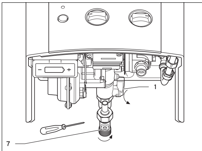
Abb. 4.6 Außerbetriebnahme
