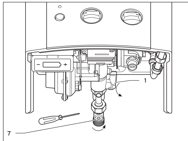
Abb. 4.2 Absperreinrichtungen
