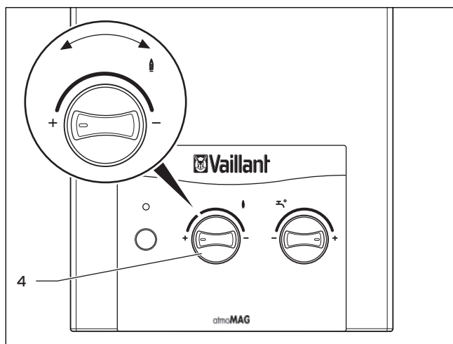
Abb. 4.5 Leistungsvorwahl
