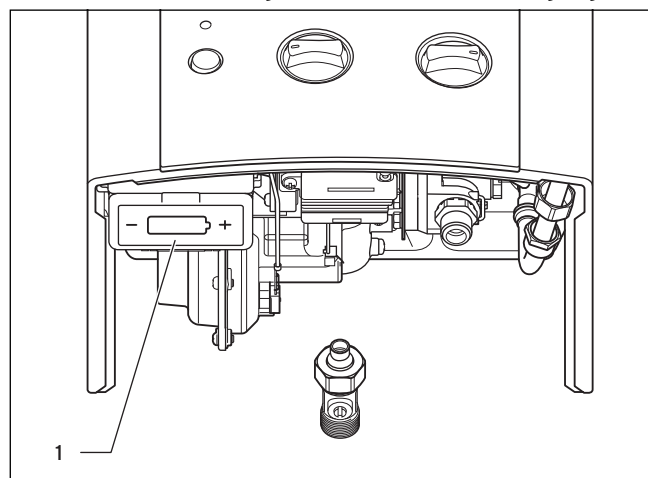
Fig. 4.8 Batteriewechsel
