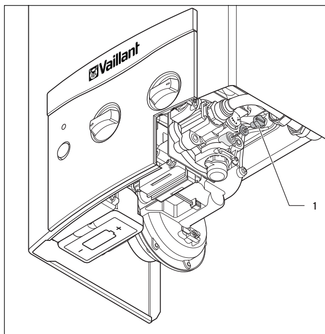
Abb. 4.7 Entleerung
