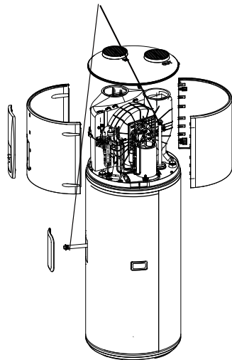
Hořčičková anoda
