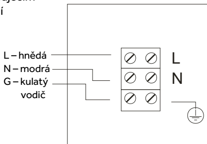
Připojení terminálů tepelného čerpadla
