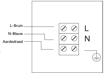
Aansluitblok van de warmtepomp
