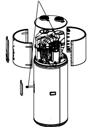
Magnesium anode
