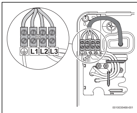
Rys. 155 Podłączenie od góry
