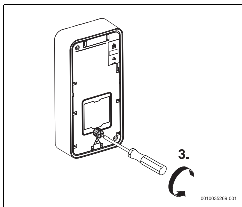
Fig. 67 Desserrer la vis
