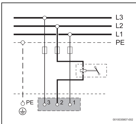
Fig. 98 Schéma de câblage
