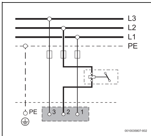
Rys. 154 Schemat elektryczny
