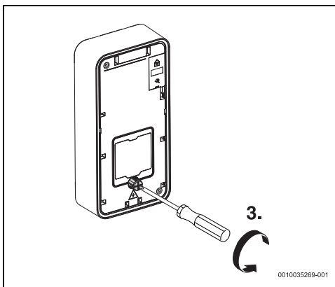
Rys. 123 Wykręcanie śruby
