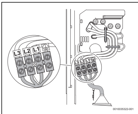
Rys. 156 Podłączenie od dołu
