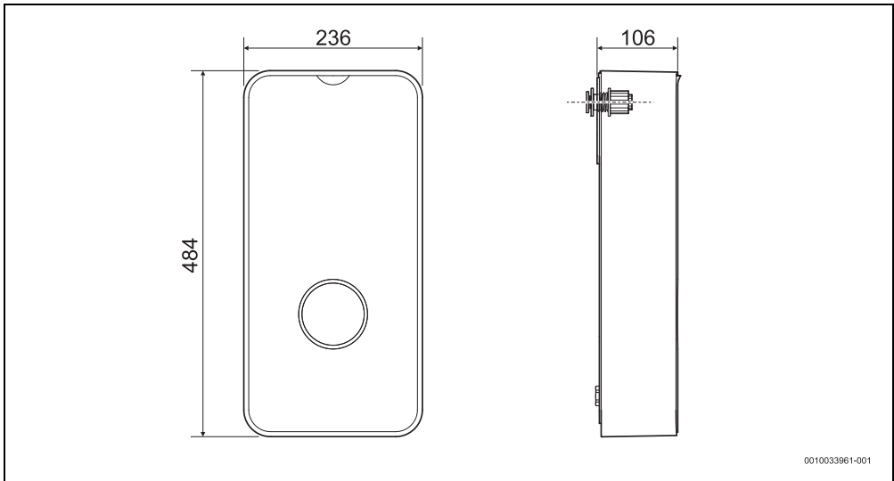
Fig. 58 Dimensions en mm
