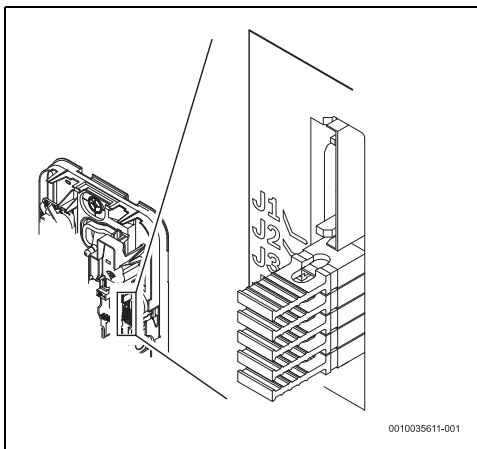
Rys. 151 Dołączone zworki elektroniczne
