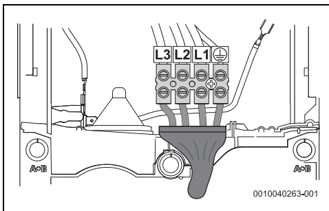
Rys. 164 Przyłącze od dołu na krótkie kable
