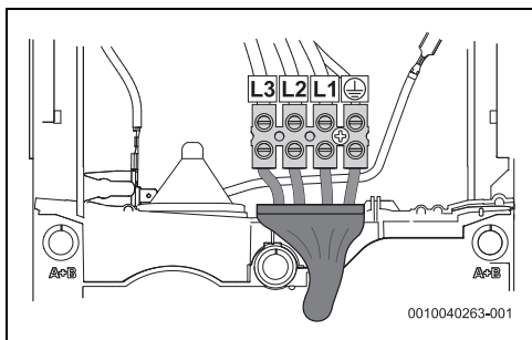
Rys. 157 Przyłącze od dołu na krótkie kable
