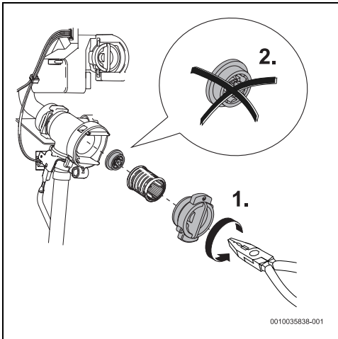
Fig. 113 retirer le limiteur de débit.
