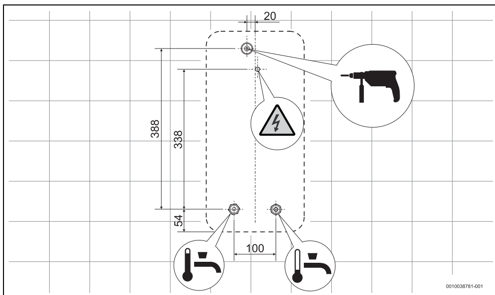
Rys. 115 Wymiary w mm
