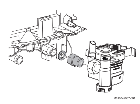
Rys. 141 Dodatkowa tuleja
