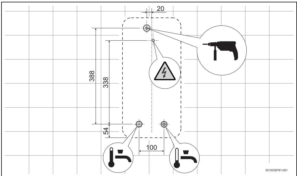
Fig. 59 Dimensions en mm
