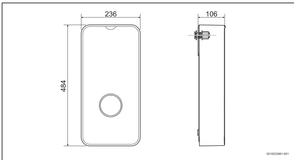
Rys. 114 Wymiary w mm
