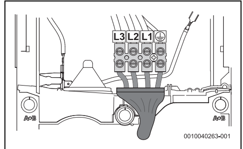
Fig. 108 Raccordement inférieur pour câble court
