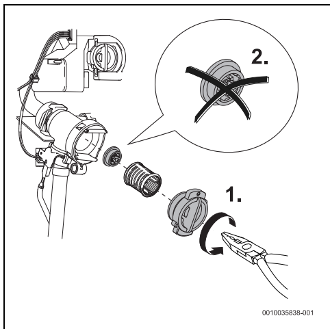
Rys. 169 Usuwanie ogranicznika przepływu.
