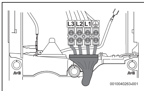
Fig. 101 Raccordement inférieur pour câble court
