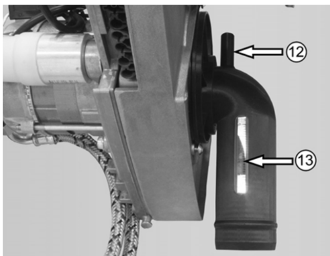
Abb. 5: Anschluss-Stück RLU
