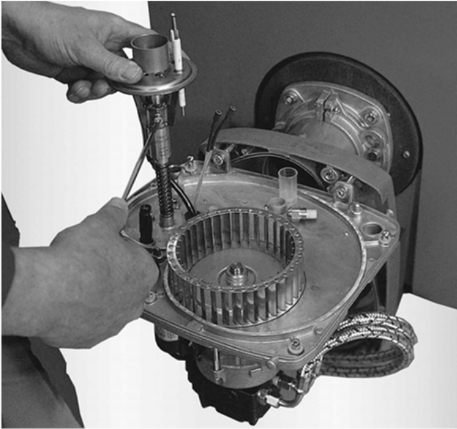
Abb. 37: Demontage Mischsystem
