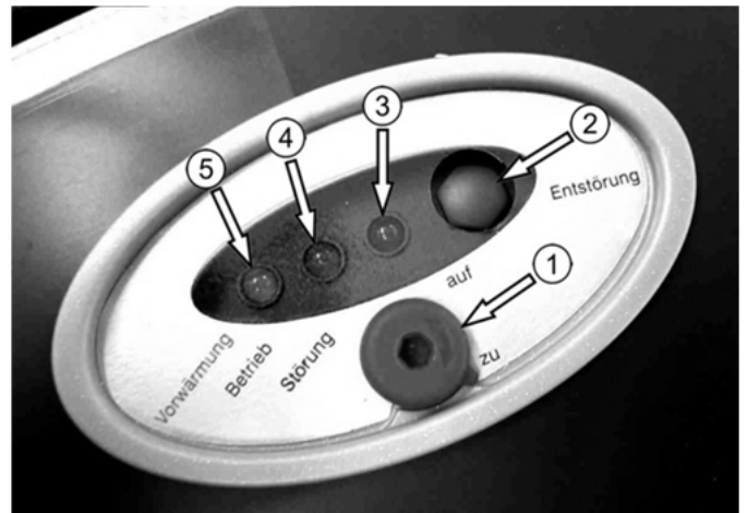
Abb. 15: Lampenfeld RE 1H / RE 1HK / RE 1 HG
