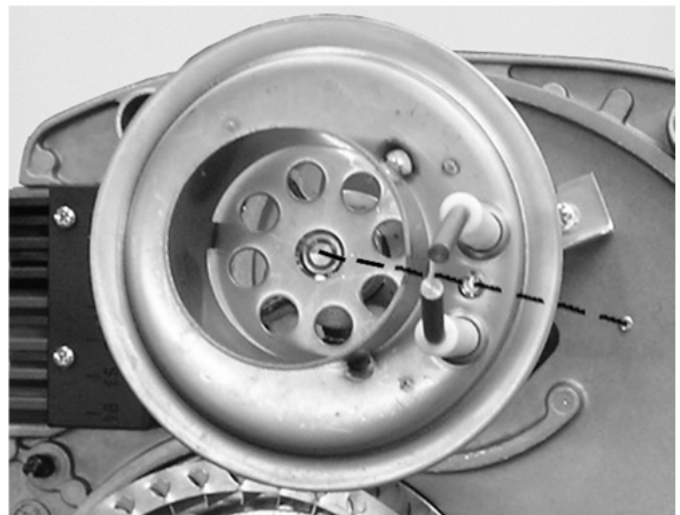
Abb. 40: Mischsystempositionierung und Ausrichtung Zündelectrode
