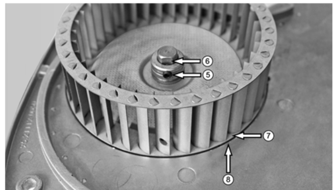
Abb. 43: Axiale Positionierung des Gebläserades
