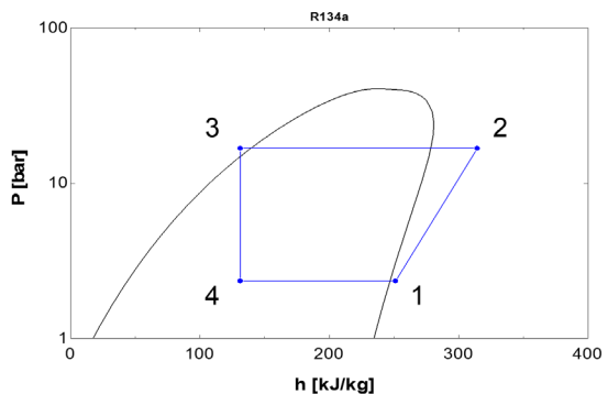
Abbildung 2 - Druck-Enthalpie-Diagramm
