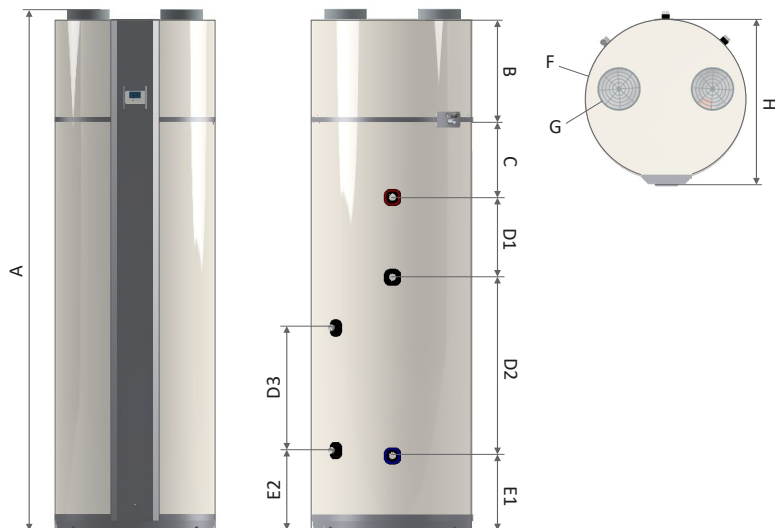
Abbildung 6 - Abmessungen
