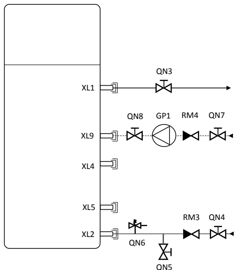
Abbildung 11 – Diagramm der vorgeschlagenen Wasserkreisverbindungen
