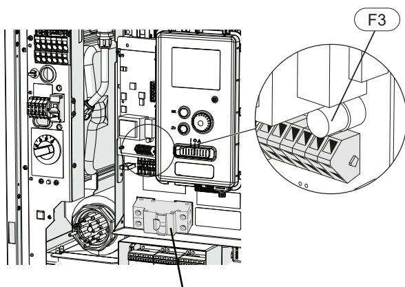
Fehlerschutzschalter RCD
