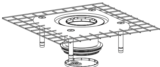
Aufstockelement CeraDrain Collar CeraDrain / Élément de rehausse CeraDrain / Opbouwelement CeraDrain / Elemento de elevación CeraDrain / Elemento de aumento CeraDrain / Przedłużka CeraDrain 563002
