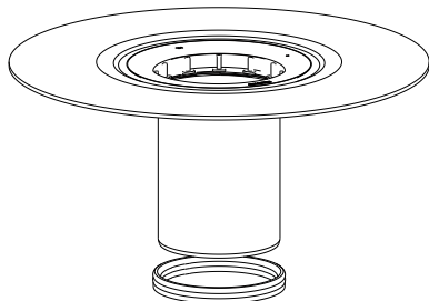
Aufstockelement 550 DallBit Raising piece / Élément de rehausse / Opbouwelement / Elemento de elevación / Elemento de aumento / Przedłużka 562005
