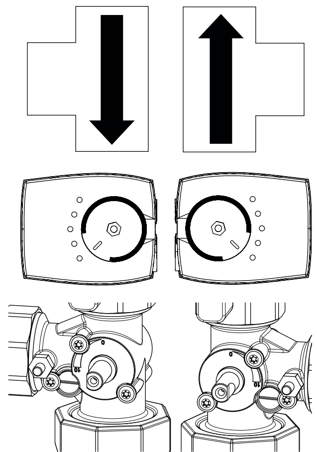
Abb. 30: Stellung Umschaltventile bei Beladung Trinkwasser
