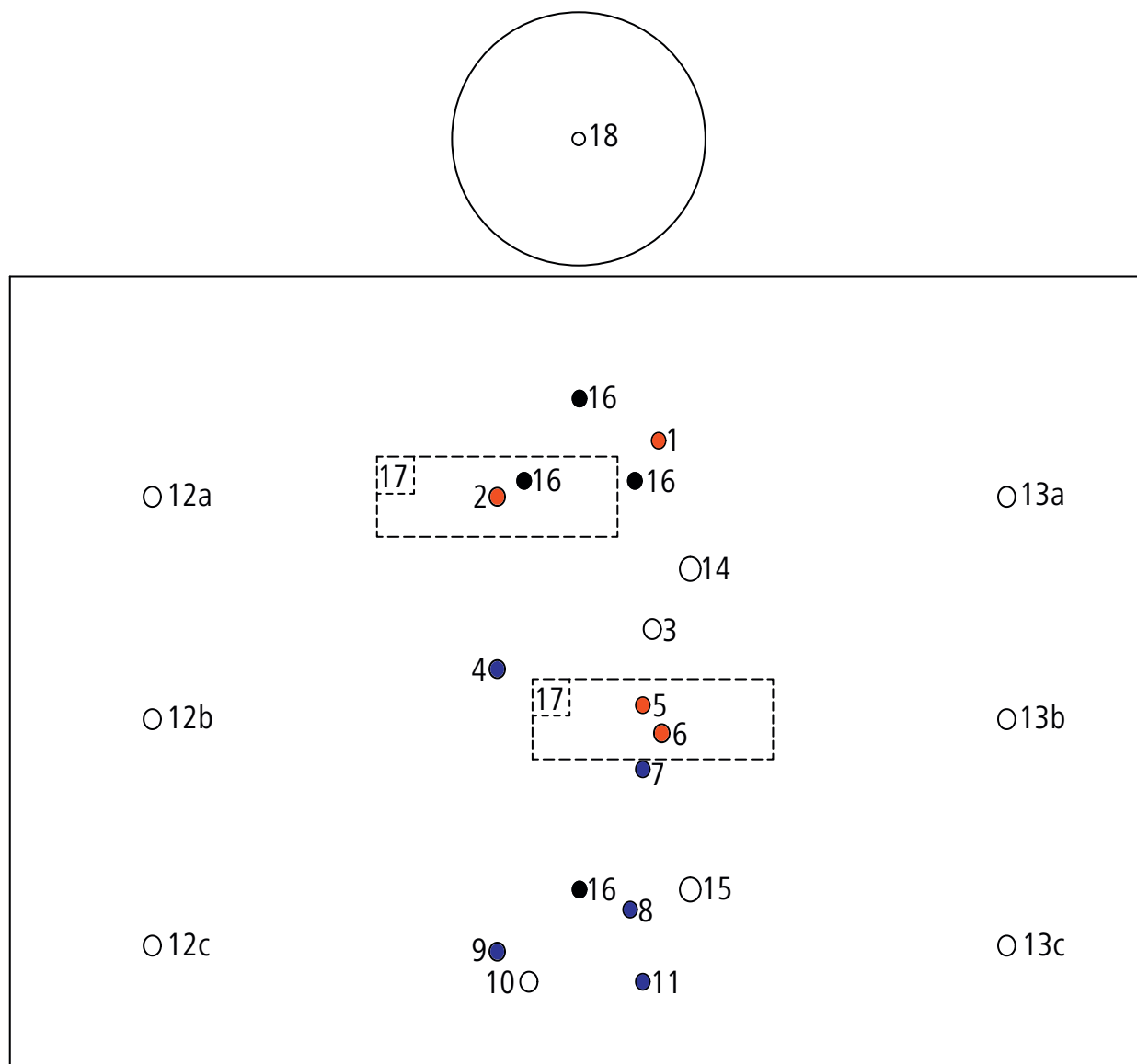
Abb. 36: Stutzenübersicht
