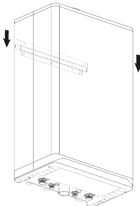
Abb. 6: Montage des Gerätes
