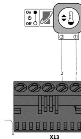
Abb. 18: Anschluss Raumthermostat oder OpenTherm Raumeinheit
