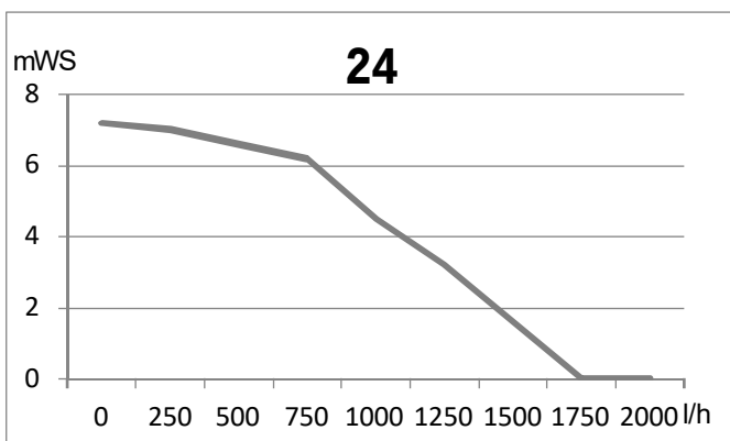
Abb. 121: Restförderhöhe ecoGAS Pro 24
