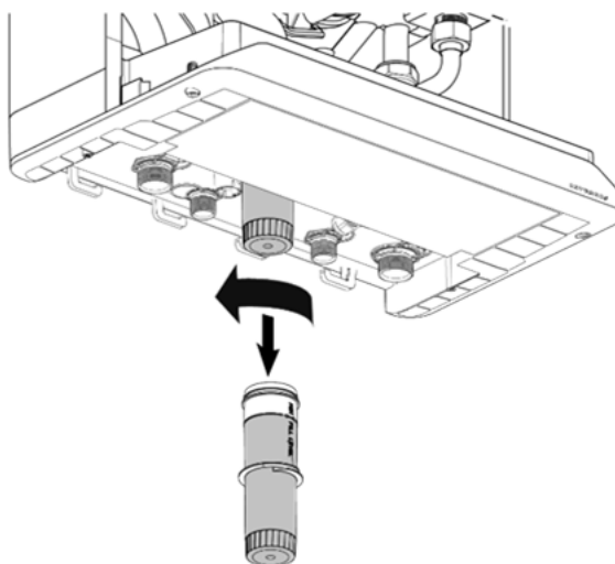
Abb. 98: Demontage der Siphontasse
