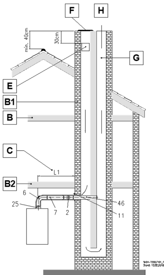
Abb. 34: C 43x Anschluss an ein Luft-Abgas-System (LAS)
