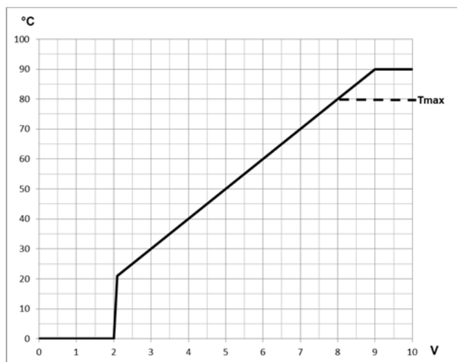
Abb. 19: Vorlauftemperatur-Sollwert in Abhängigkeit des 0-10 V Steuersignals
