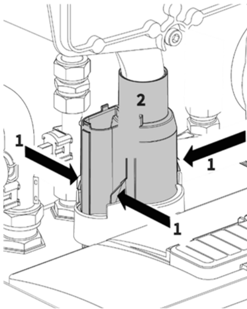
Abb. 99: Demontage des Siphons
