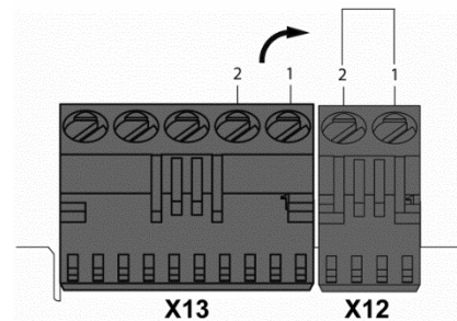
Abb. 17: Versetzte Brücke für Betrieb mit LANfunk-Box
