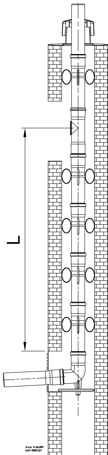
Abb. 58: Kaminsystem, starr, zur Ermittlung von Abstandsmaß L
