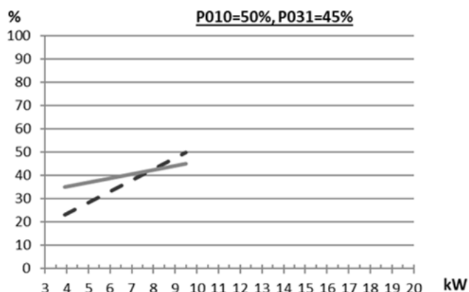
Abb. 86: Heizleistung und Pumpendrehzahl am Beispiel ecoGAS Pro 18 mit reduziertem Parameter P010 (= 50 %) und reduziertem Parameter P031 (= 45 %)
