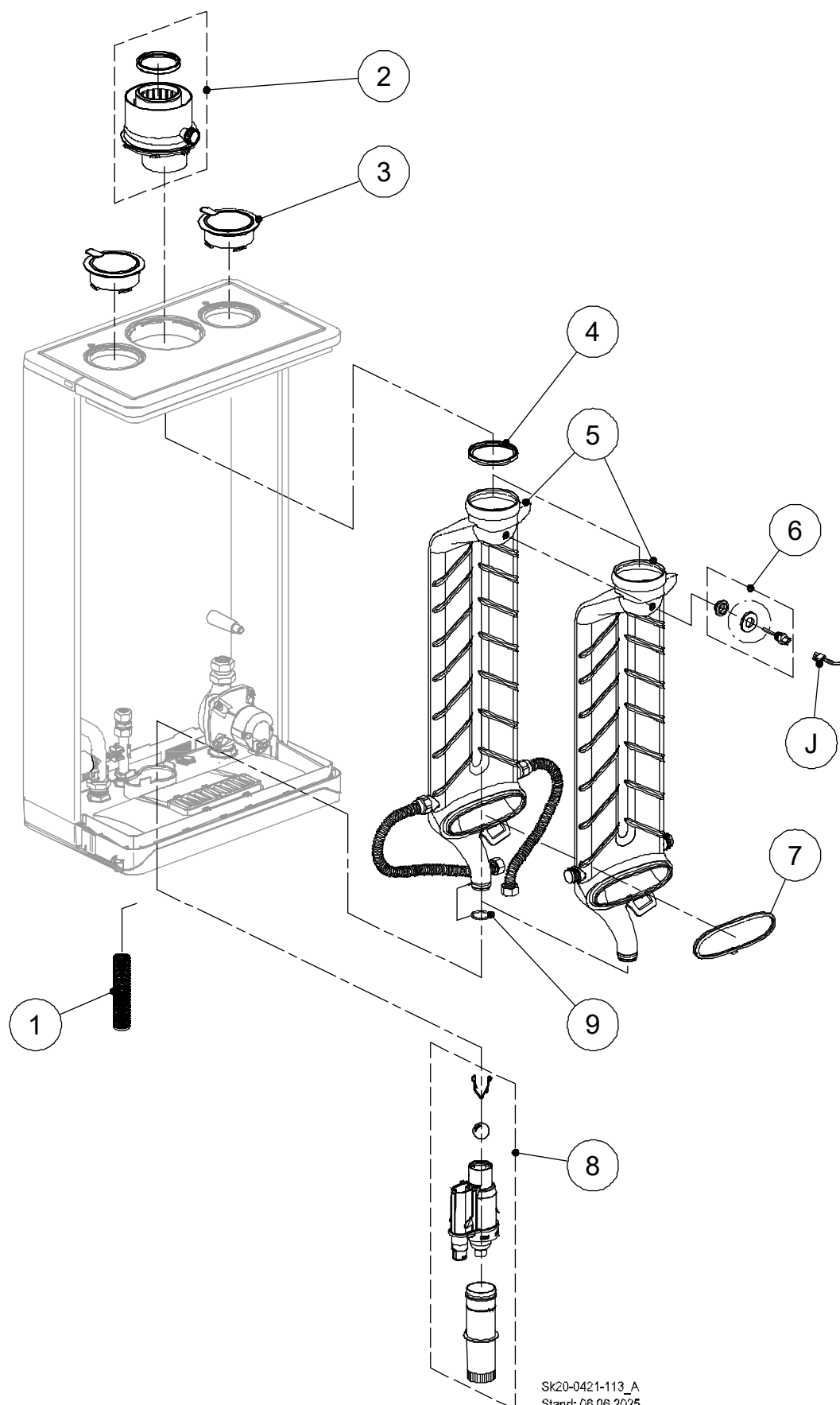
Abb. 113: Abgas und Kondensat
