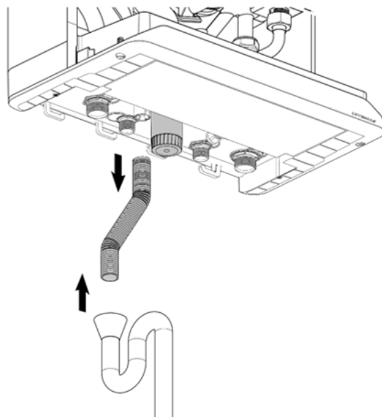
Abb. 97: Demontage des Kondensatschlauchs
