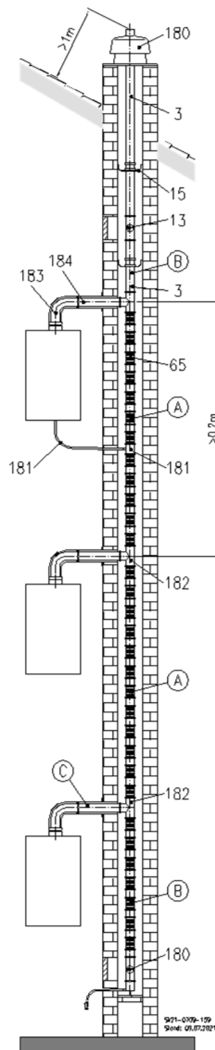
Abb. 43: C (11)3x Mehrfachbelegung im Schacht
