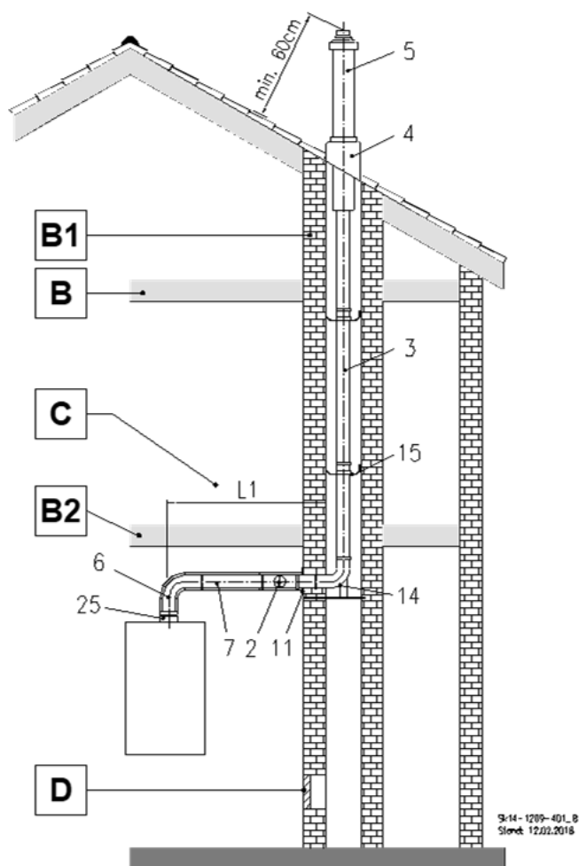
Abb. 38: C 93x Luft-Abgas-System im Schacht und Luft-Abgas-Rohrsystem mit Dachdurchführung
