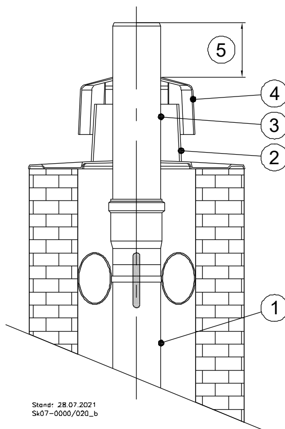
Abb. 59: Schachtabdeckung
