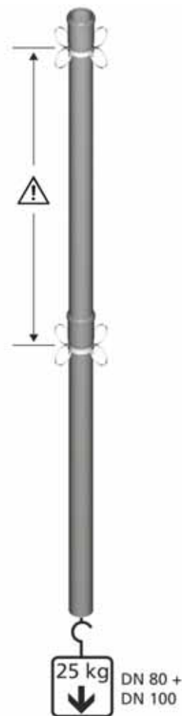
Abb. 57: Abgasrohre mit Stoppring-Technik ①
