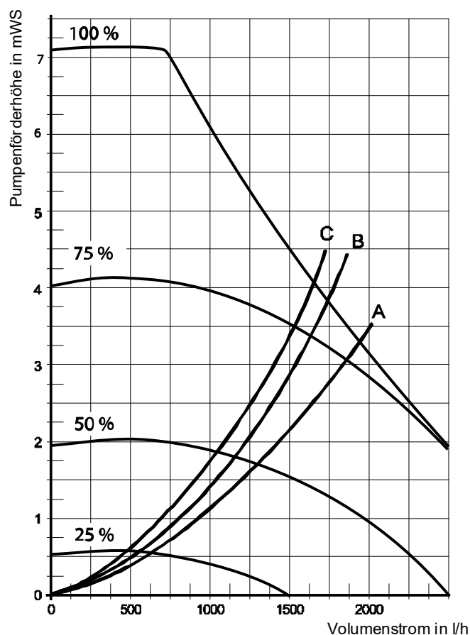
Abb. 87: Hydraulischer Druckverlust des Wärmetauschers auf der Heizungsseite
