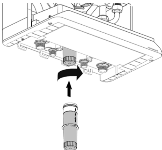
Abb. 104: Montage der Siphontasse
