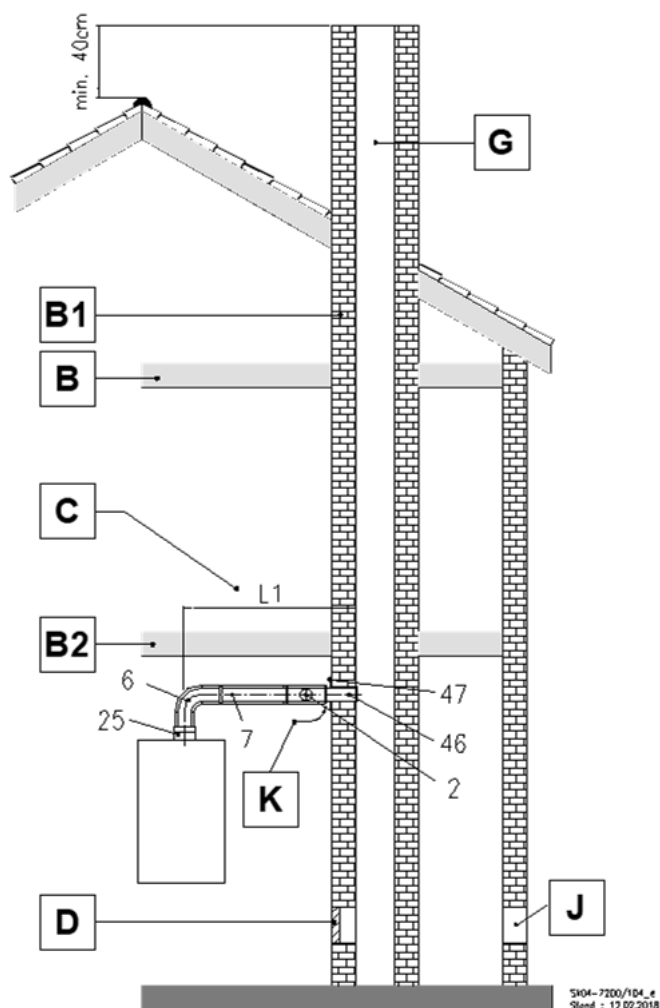
Abb. 30: B 33 Abgasrohr endet im feuchteunempfindlichen Schornstein
