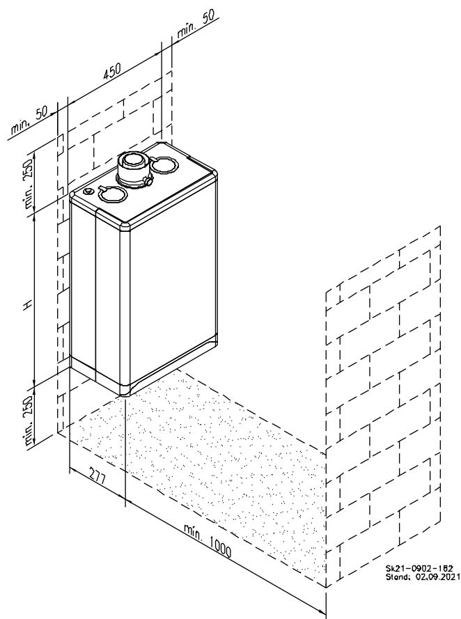
Abb. 3: Montageabstände
