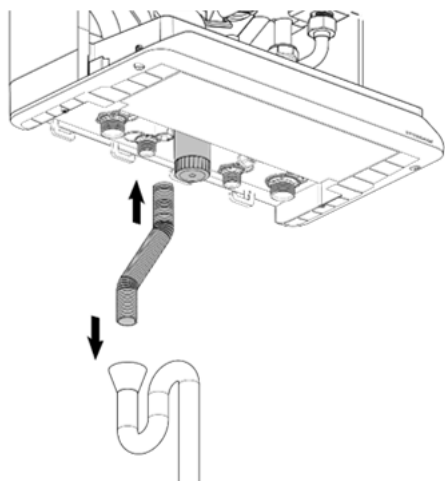
Abb. 105: Montage Kondensatschlauch
