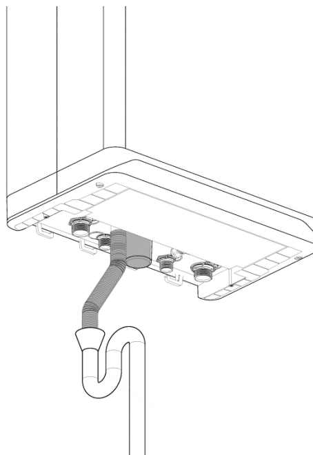
Abb. 9: Frei abtropfender Kondensatablauf
