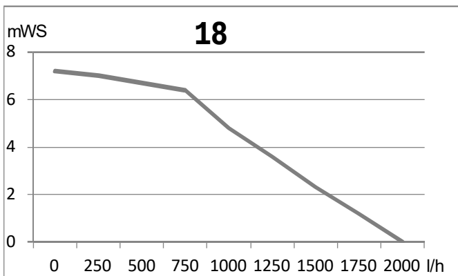
Abb. 120: Restförderhöhe ecoGAS Pro 18, ProX 18/24
