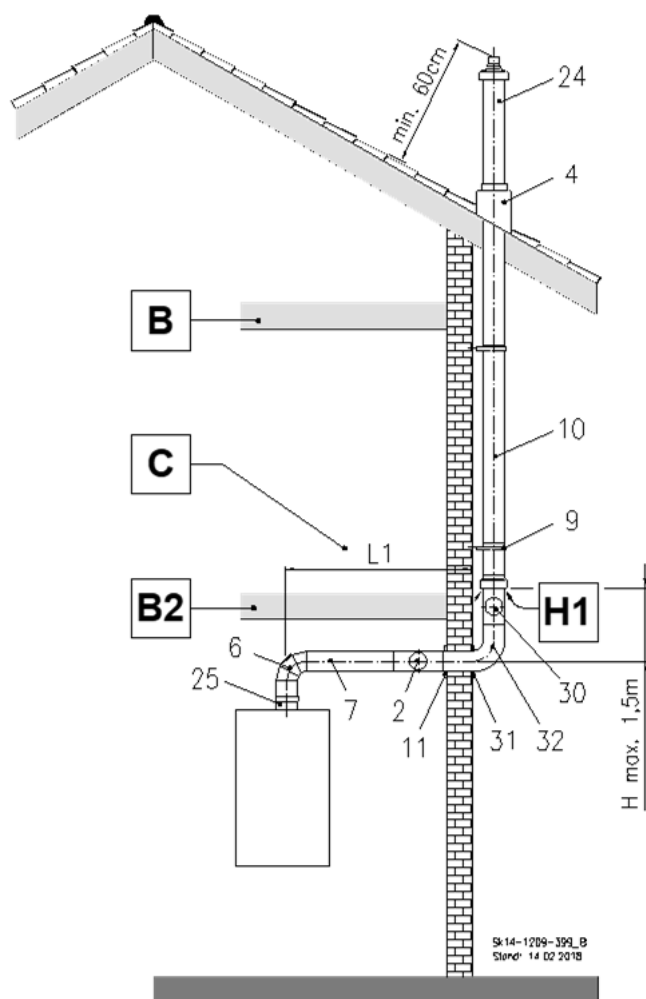
Abb. 35: C 53x Außenwandführung LAS
