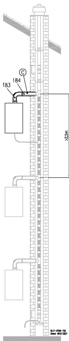
Abb. 41: C (10)3x Mehrfachbelegung im Schacht
