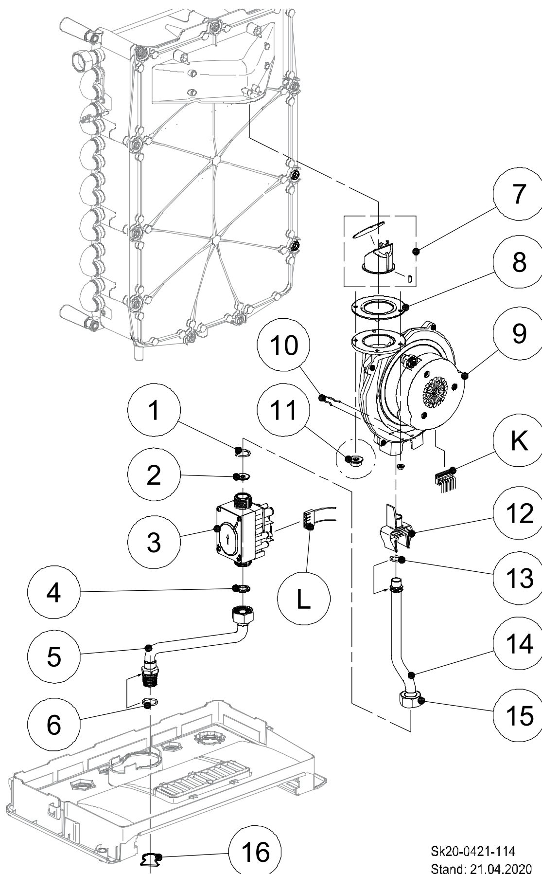
Abb. 114: Gasarmatur und Gebläse
