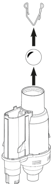
Abb. 100: Sicherungsklammer und Kunststoffkugel des Siphons
