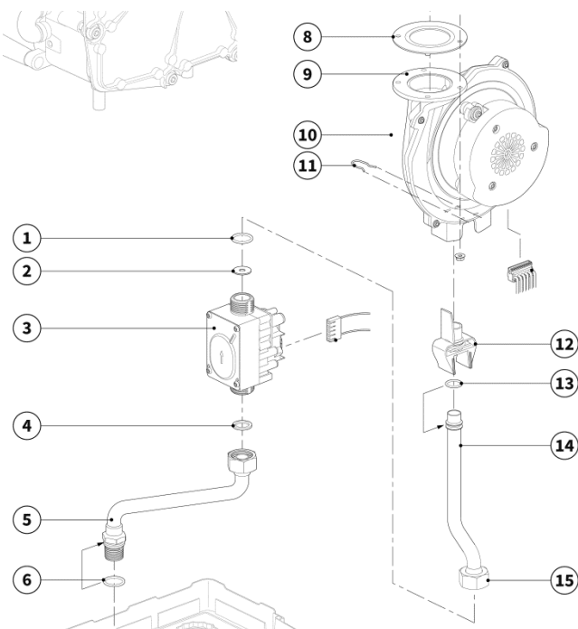
Abb. 95: Komponenten des Gas-Luft-Verbundes
