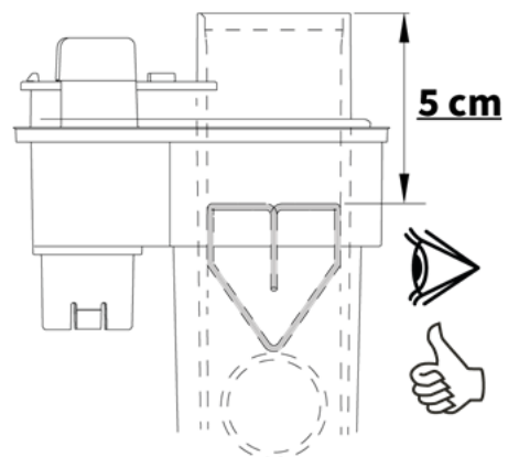
Abb. 101: Korrekte Position von Sicherungsklammer und Kunststoffkugel
