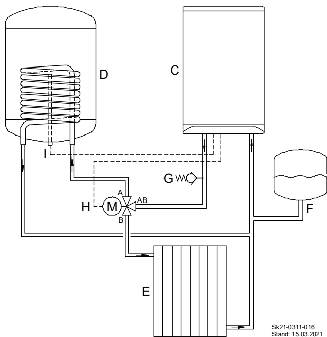
Abb. 23: Trinkwarmwasserbereitung mit externem Speicher über 3-Wege-Umschaltventil
