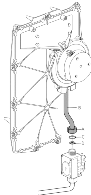
Abb. 92: Umbau Gasdüse
