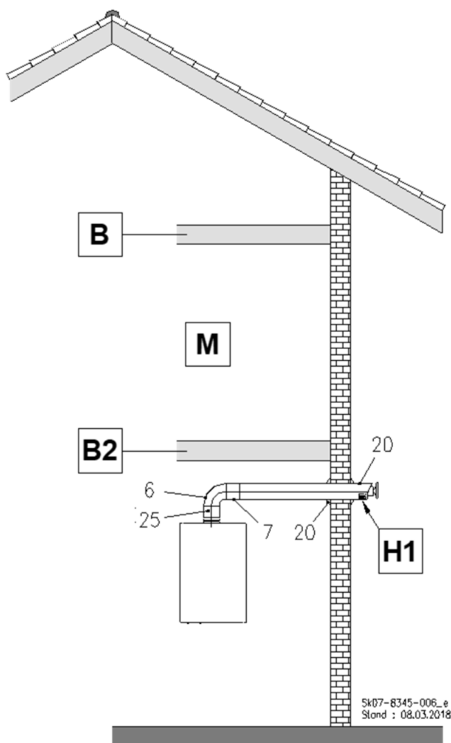
Abb. 31: C 13x Luft-Abgas-Rohrsystem horizontal durch die Außenwand
