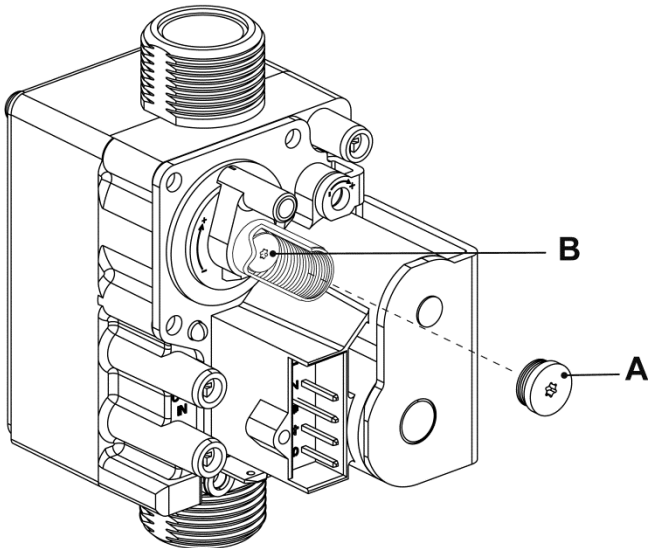
Abb. 96: Gasventil
