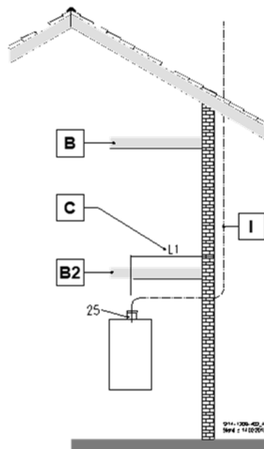
Abb. 36: C 63x Für Anschluss an eine nicht mit der Gasfeuerstätte geprüfte Verbrennungsluftzuführung und Abgasabführung
