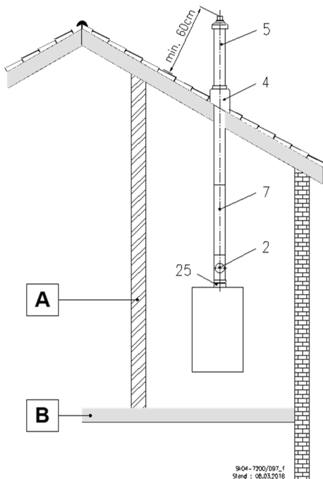
Abb. 33: C 33x Dachheizzentrale mit der Durchführung senkrecht durch ein Schrägdach
