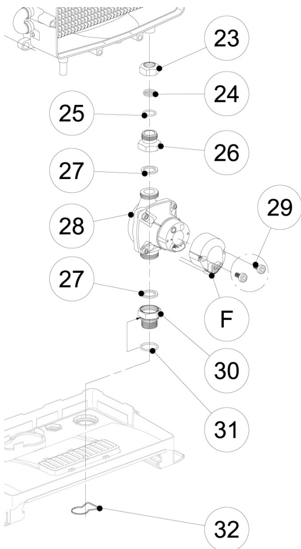
Abb. 107: Umwälzpumpe mit Verschraubungen
