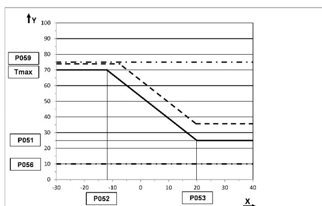
Abb. 91: Heizkennlinie mit Parallelverschiebung (T RaumSoll = 24 °C, P054 = 3) und Begrenzung durch Parameter P059
