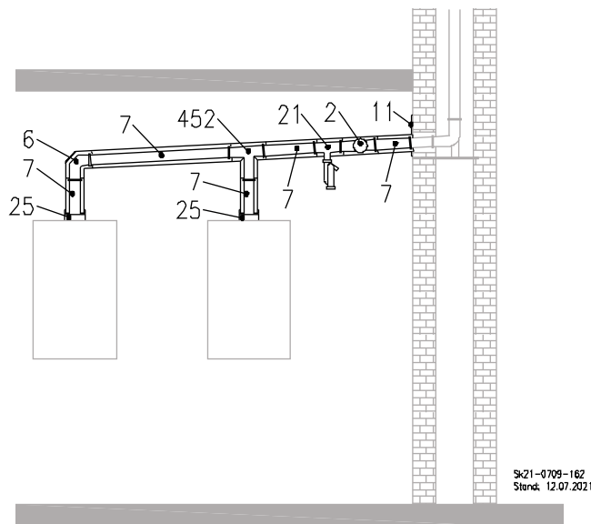
Abb. 54: RLU Kaskade
