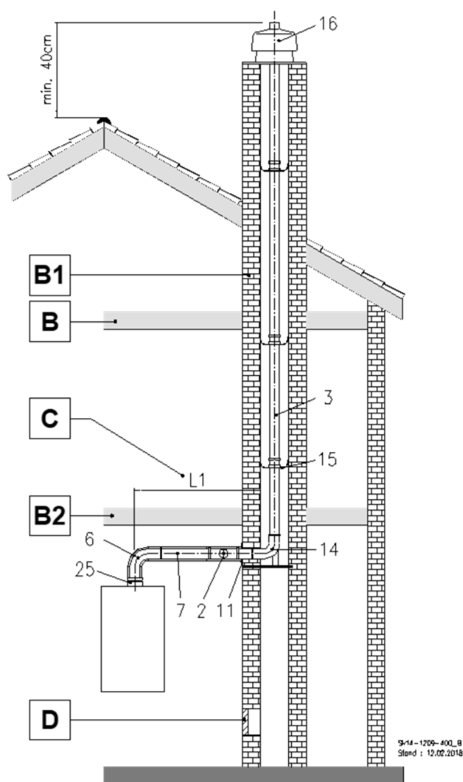
Abb. 39: C 93x Abgasrohr im Schacht
