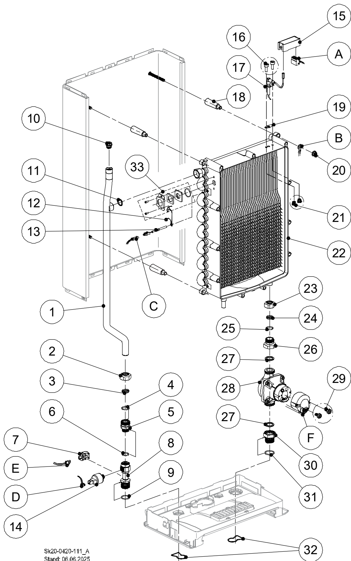
Abb. 111: Wärmetauscher mit Hydraulik Heizkreis
