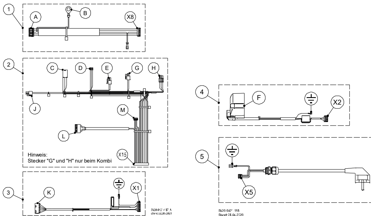
Abb. 117: Verdrahtung
