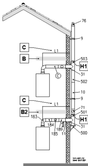
Abb. 48: C (13)3x Mehrfachbelegung an der Außenwand
