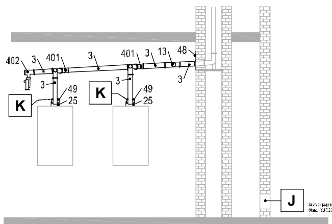
Abb. 55: RLA Kaskade
