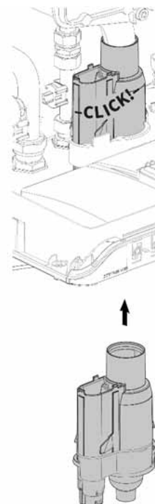
Abb. 102: Montage des Siphons
