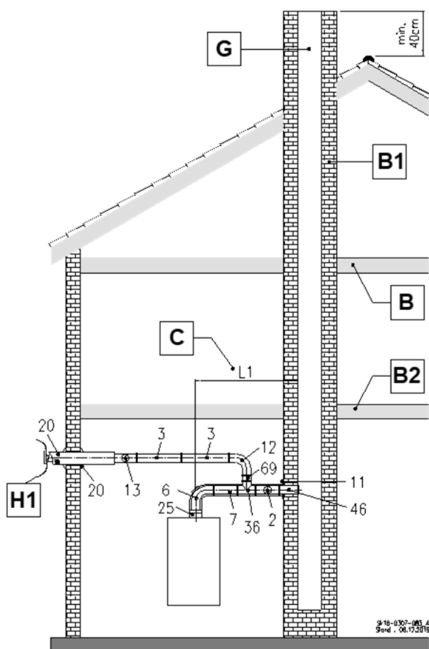
Abb. 37: C 83x Anschluss an einen feuchte-unempfindlichen Abgasschornstein und Zuluft durch die Außenwand
