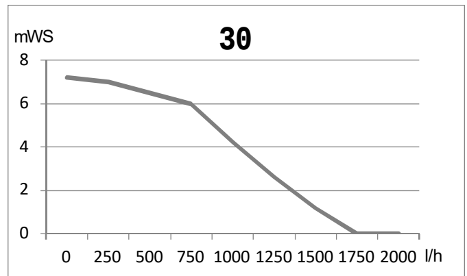
Abb. 122: Restförderhöhe ecoGAS Pro 30, ProX 30/38
