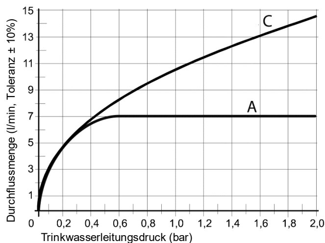
Abb. 13: Widerstandsdiagramm Trinkwasser-Tauscherschlange
