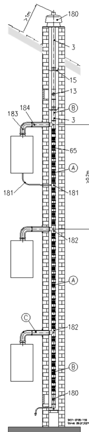
Abb. 51: C (14)3x Mehrfachbelegung im Schacht
