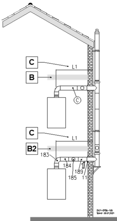
Abb. 46: C (12)3x Mehrfachbelegung an der Außenwand
