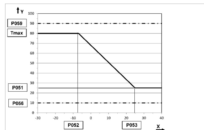
Abb. 88: Heizkennlinie gemäß Werkseinstellungen
