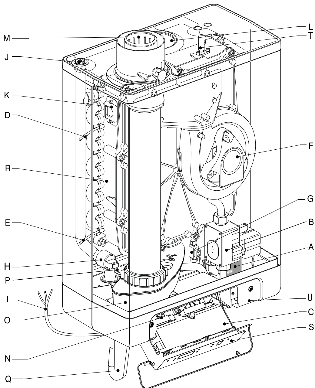
Abb. 2: Hauptkomponenten
