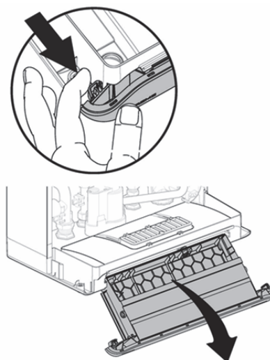
Abb. 3: Öffnen der Regelung
