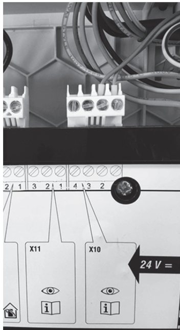
Abb. 5: Anschlussklemme X10
