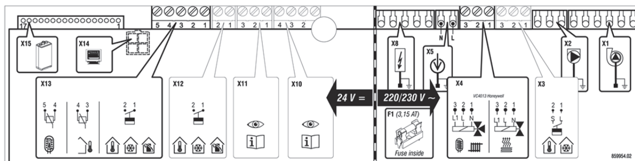
Abb. 2: Aufkleber Elektrische Anschlüsse
