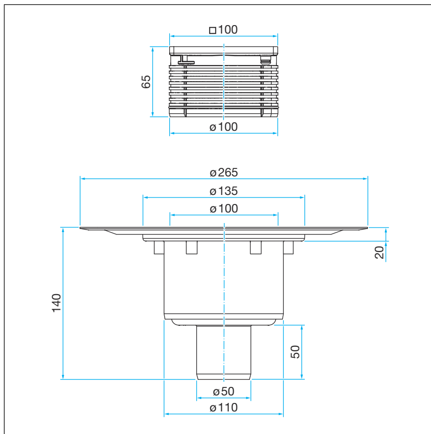
Abb. 5: Maßzeichnung Modell 4926
