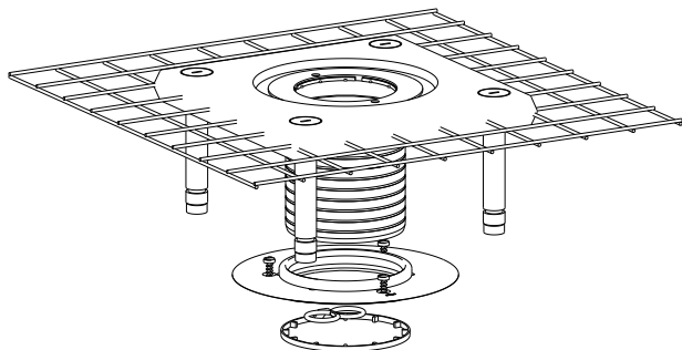
Aufstockelement CeraDrain S 10 Collar CeraDrain / Élément de rehausse CeraDrain / Opbouwelement CeraDrain / Elemento de elevación CeraDrain / Elemento de aumento CeraDrain / Przedłużka CeraDrain 563069
