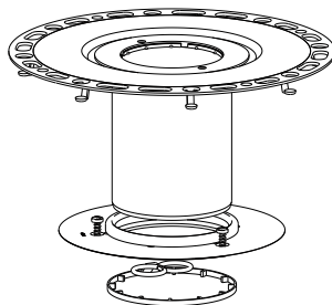
Aufstockelement TistoDrain S 10 Collar TistoDrain / Élément de rehausse TistoDrain / Opbouwelement TistoDrain / Elemento de elevación TistoDrain / Elemento de aumento TistoDrain / Przedłużka TistoDrain 513168
