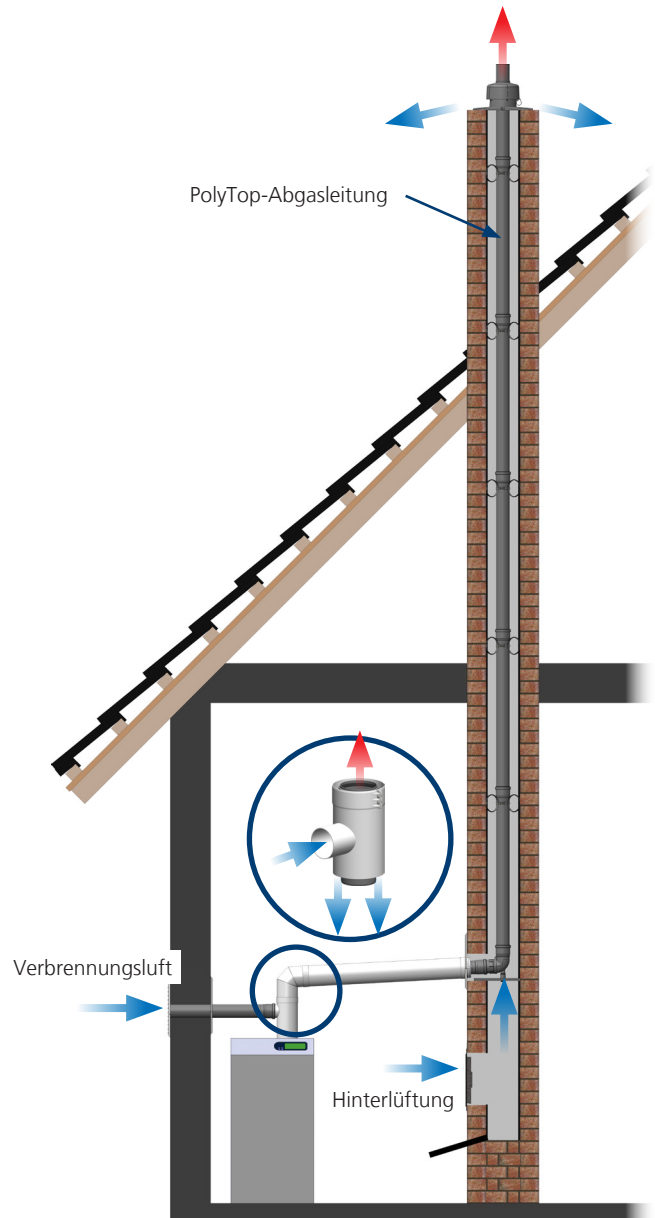
Abb. 3: Zuluft nach Art C 5 , Abgasleitung im Schacht mit Hinterlüftung im Gleichstrom
