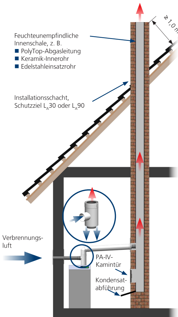
Abb. 5: Zuluft nach Art C 8 (C 12 ), Schacht mit feuchteunempfindlicher Innenschale
