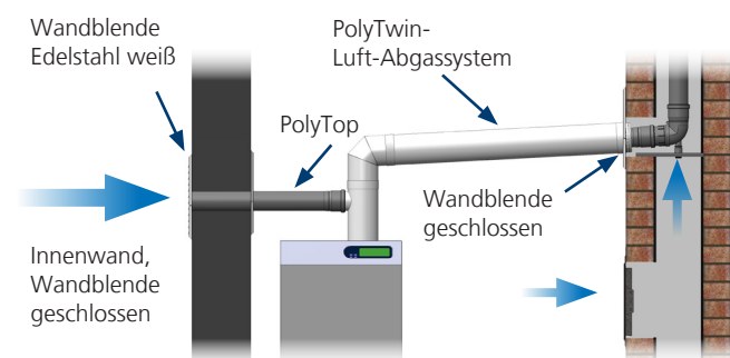
Abb. 4: Detail, Zuluft nach Art C 5
