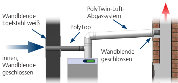
Abb. 6: Detail, Zuluft nach Art C 8 (C 12 )
