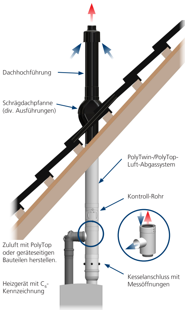
Abb. 7: Zuluft nach Art C 3 , für Heizgeräte mit Parallelanschluss
