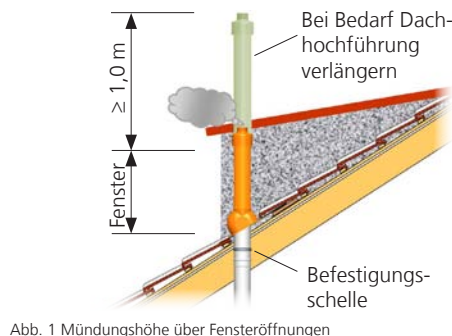
Abb. 1 Mündungshöhe über Fensteröffnungen
