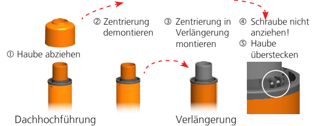
Abb. 4 Umbau der Dachhochführung und der Verlängerung
