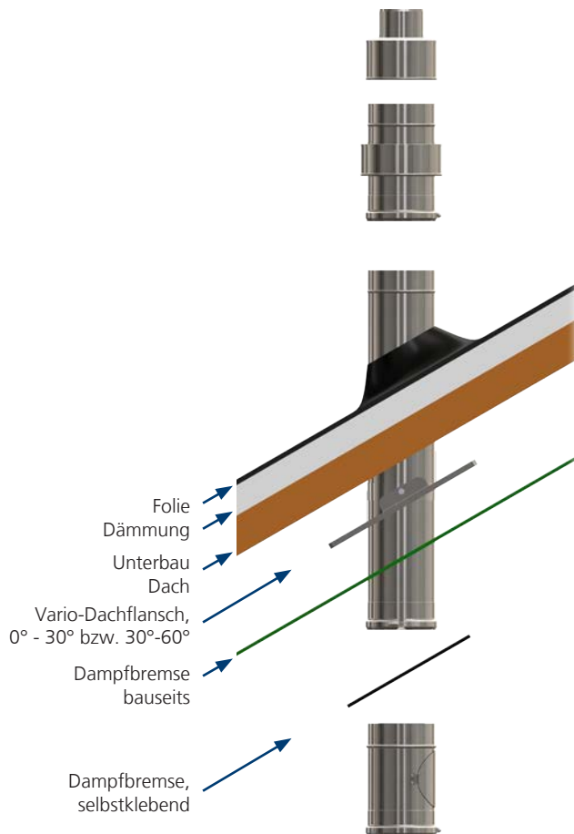
Abb. 3: Ansicht Foliendach im Schnitt
