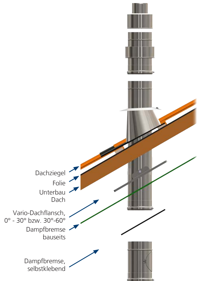
Abb. 4: Ansicht Ziegeldach im Schnitt
