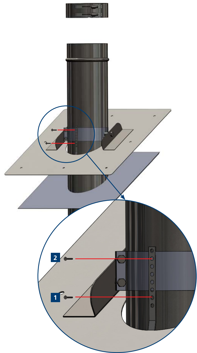
Abb. 2: Beispiel für 30° bis 60°
