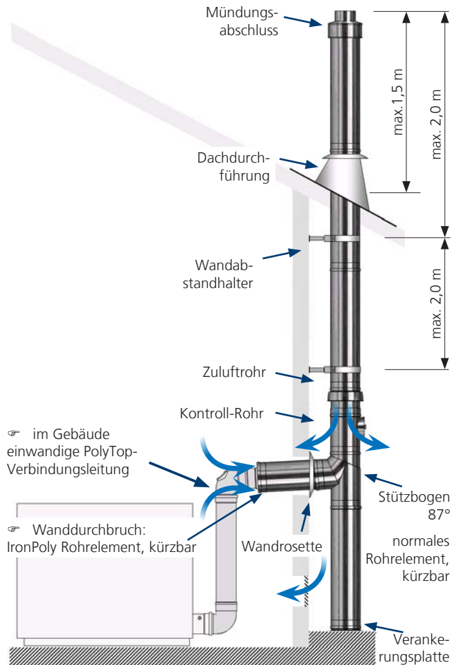
Abb. 11: bodengestützte Abgasanlage, raumluftabhängiger Betrieb
