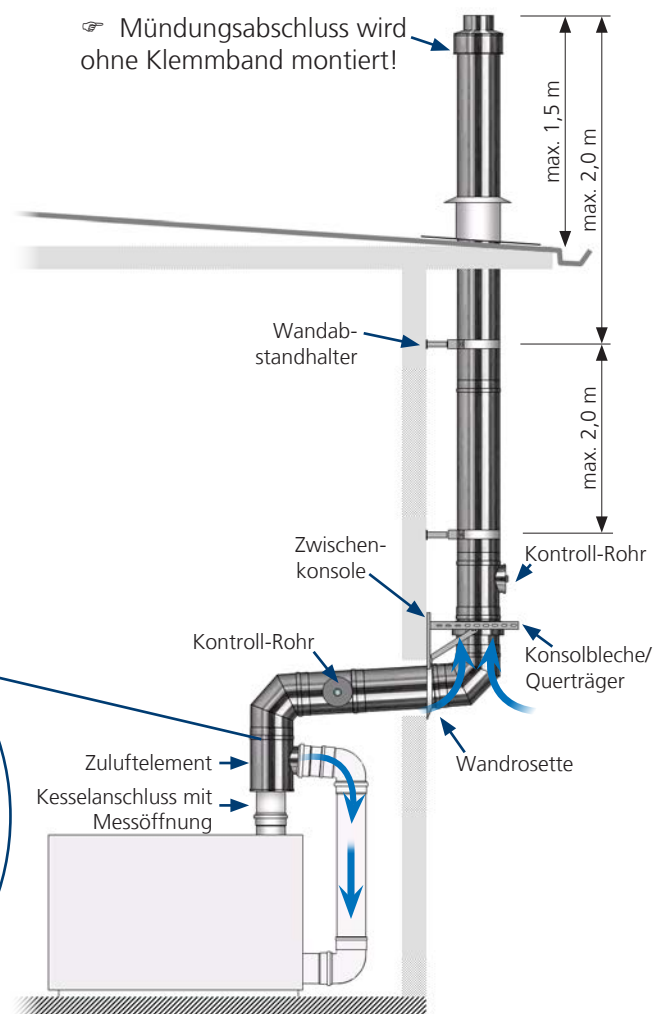
Abb. 9: querträgergestützte Abgasanlage, bedingt raumluf-tunabhängige Betriebsweise
