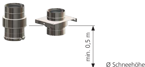
Abb. 8: Zuluftöffnungen freilassen!
