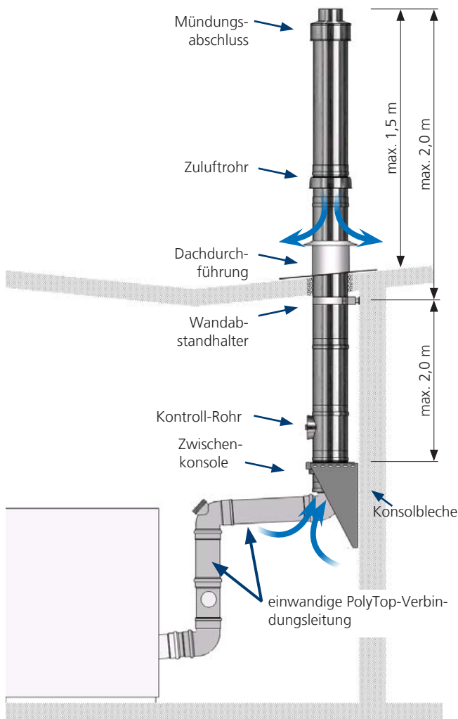
Abb. 10: konsolgestützte Abgasanlage, raumluftabhängiger Betrieb
