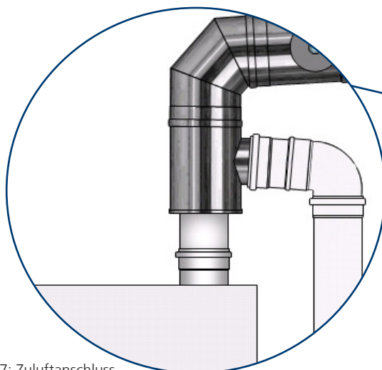
Abb. 7: Zuluftanschluss
