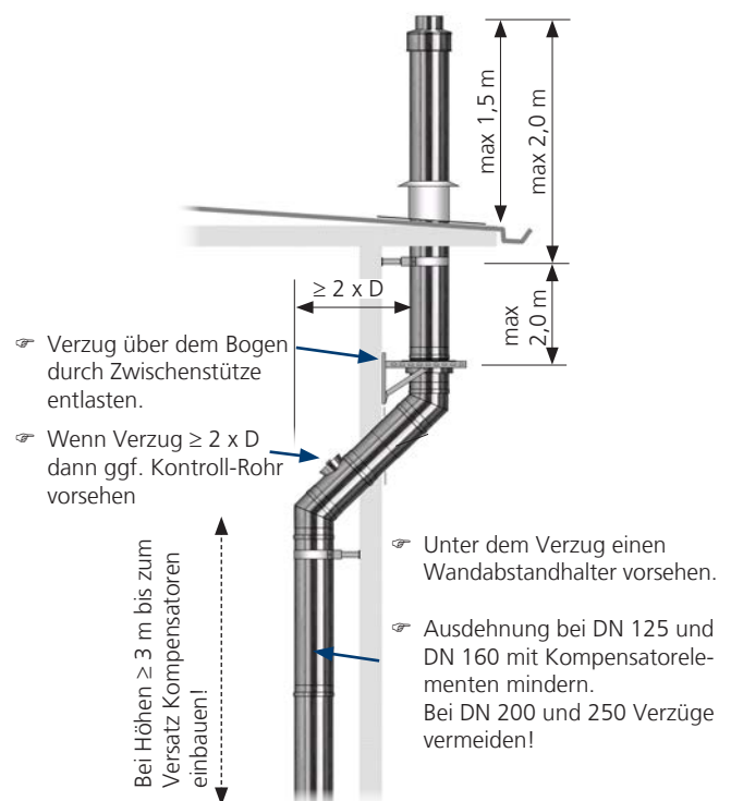
Abb. 12: typischer Versatz einer Abgasanlage
