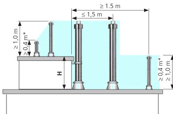
Abb. 29: Mindesthöhen für Flachdächer und Aufbauten
