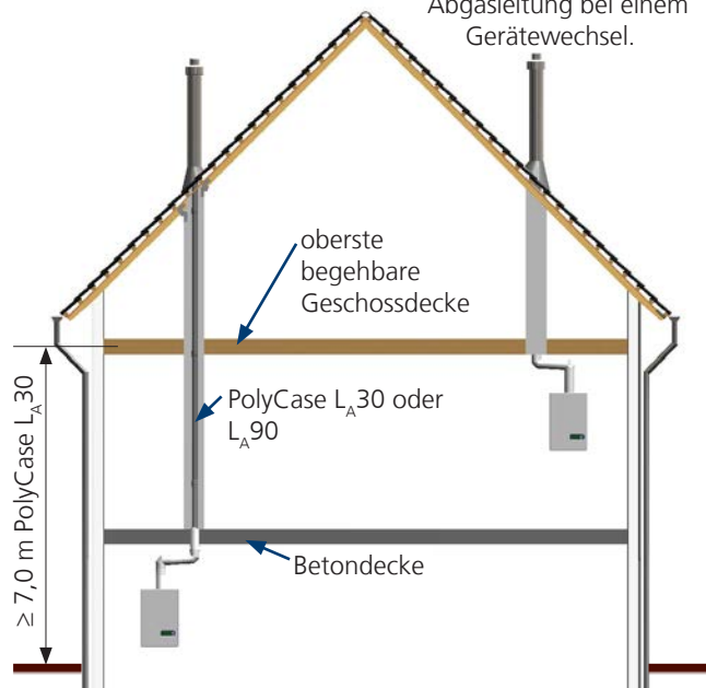
Abb. 2: deckengestützte Polycase-Abgasanlage für Beton- und Holzdecken
