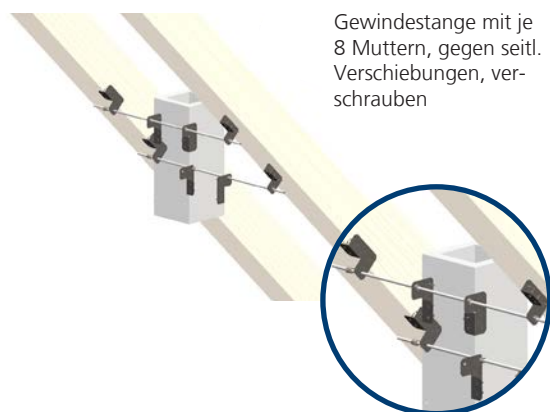
Abb. 30: typische Montage eines Sparrenhalters
