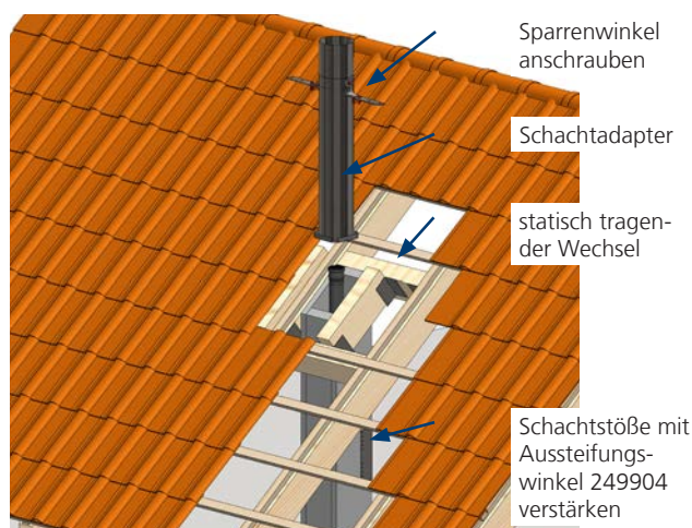
Abb. 34: typische Lastableitung mit Mündungsset PolyCase für L_A 90 -Abgasanlagen
