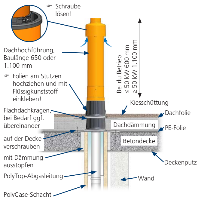
Abb. 43: Dachdurchführung DN 60/100 - 110/160
