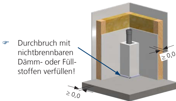
Abb. 11: Brandsicherheitsabstand zu brennbaren Baustoffen
