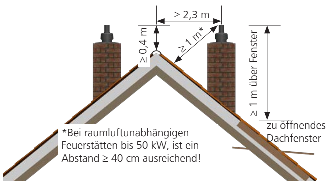
Abb. 28: Mindesthöhen über Dach bei Dachneigungen \geq 20^\circ
