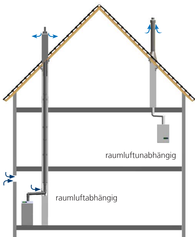
Abb. 5: mögliche Betriebsarten
