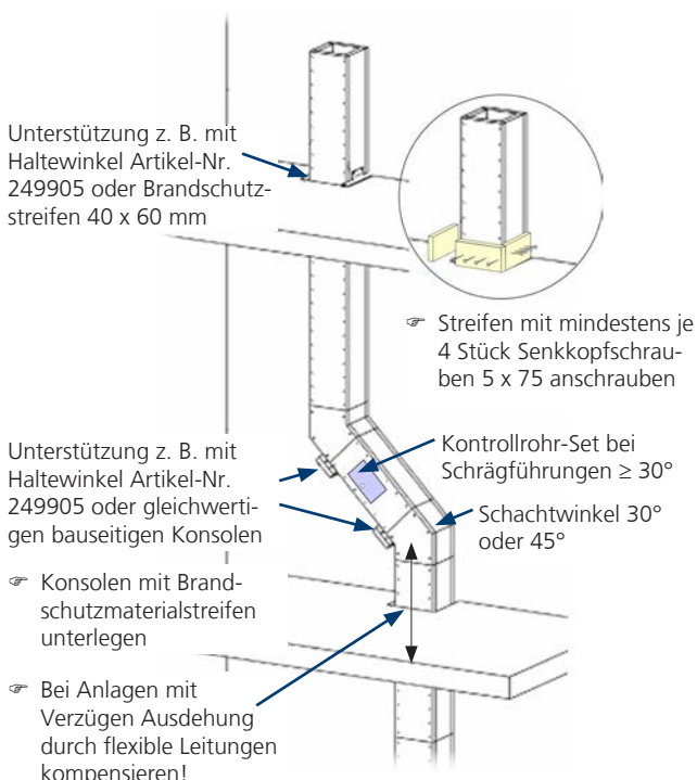
Abb. 27: typischer PolyCase-Verzug
