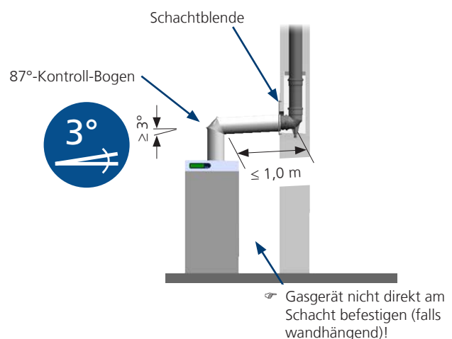
Abb. 47: typisches Verbindungsstück
