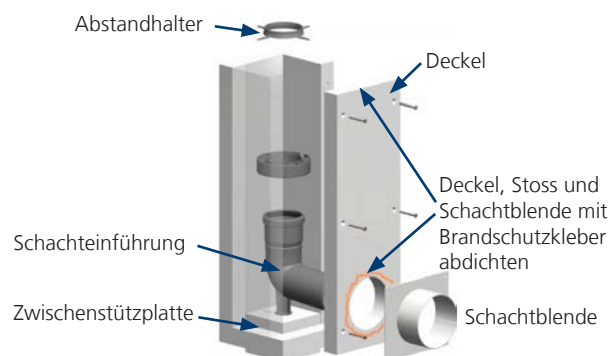
Abb. 25: Einbaudetail Schachtanschluss
