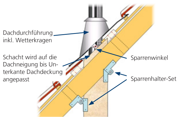
Abb. 31: Seitenansicht Dachdurchdringung mit Sparrenhalter
