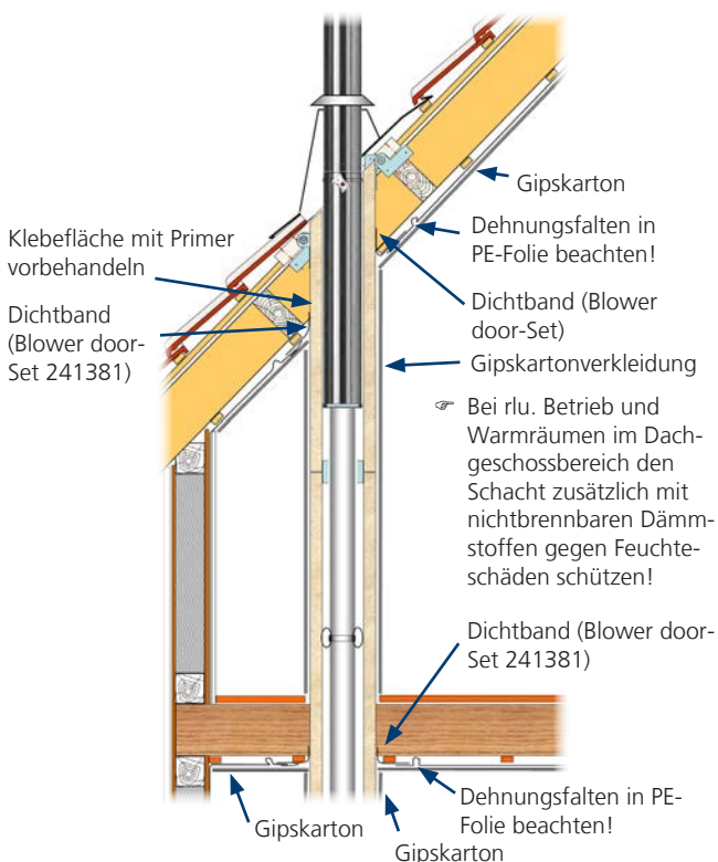
Abb. 45: typische Winddichtheits-Dichtebebenen, z. B. im Holz-Fertigbau
