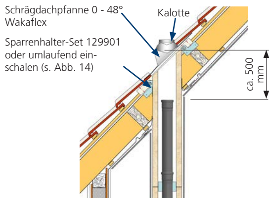
Abb. 36: Dachdurchführung bei PolyCase DN 60 bis 100
