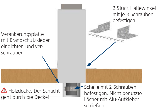
Abb. 20: Detail Holzdeckengestützter Anschluss in DN 60/100 oder DN 80/125
