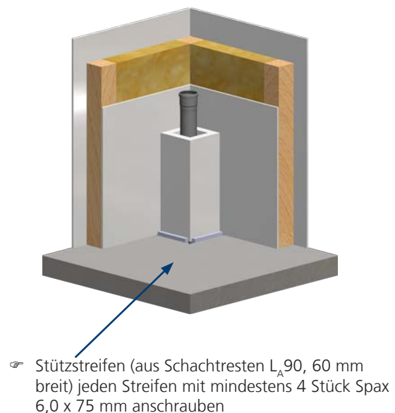
Abb. 13: Abstützung mit Streifenmaterial L_{A90} .
