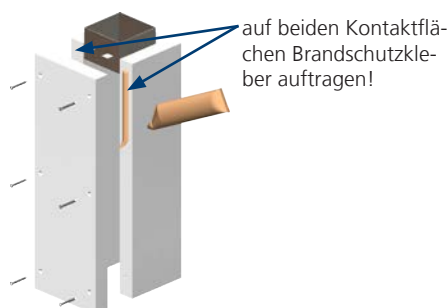
Abb. 24: Deckel eindichten
