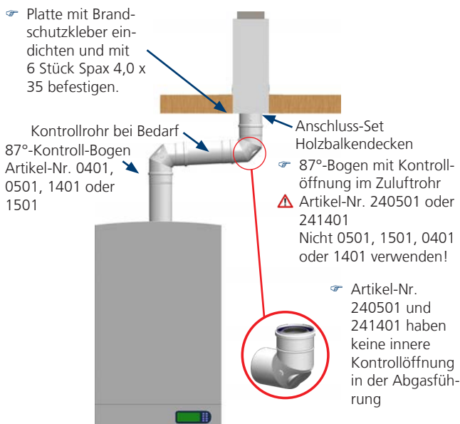
Abb. 22: Beispiel seitlicher Holzdeckenanschluss
