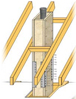
Abb. 14: Stöße unter Dach austeifen
