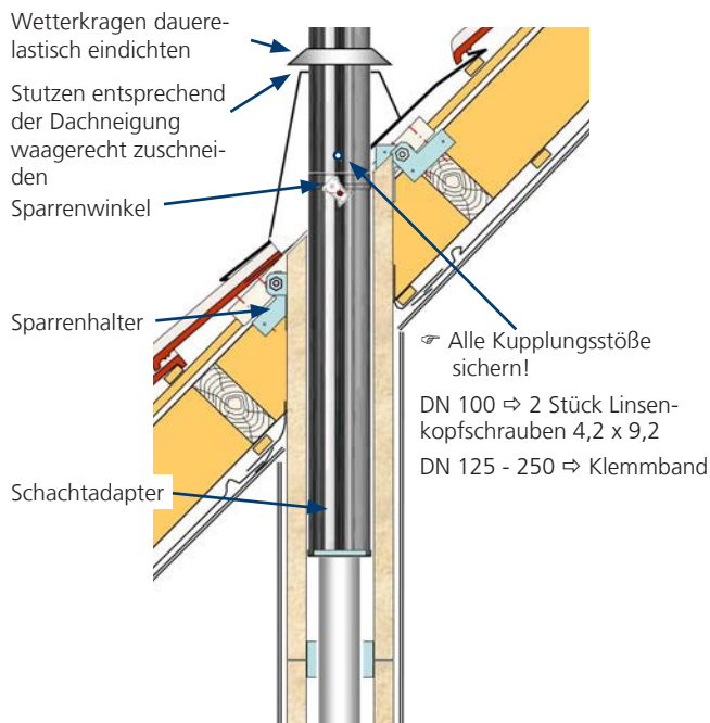
Abb. 40: Schnitt Dachdurchführung DN 100 bis 250
