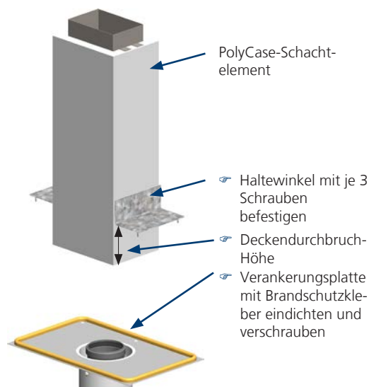
Abb. 21: Holzbalkenabstützung vorbereiten
