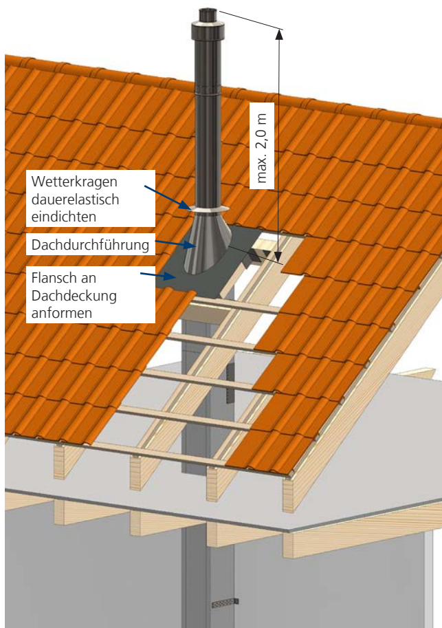
Abb. 41: fertige Mündungsausführung für PolyCase DN 100 bis 250
