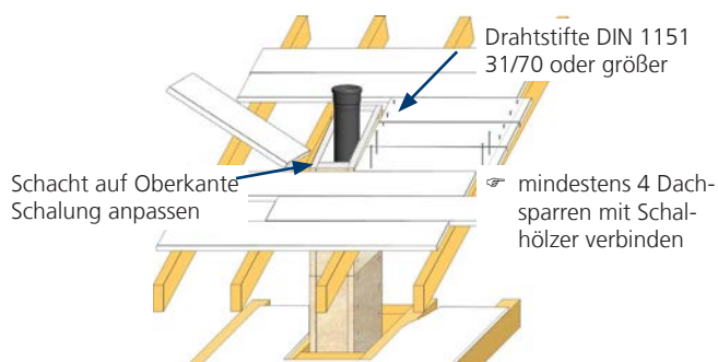
Abb. 32: Dachsparren mit Schalholz verstärken
