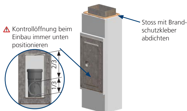
Abb. 26: Einbaudetails Kontroll-Rohr-Set und Kontroll-Rohr
