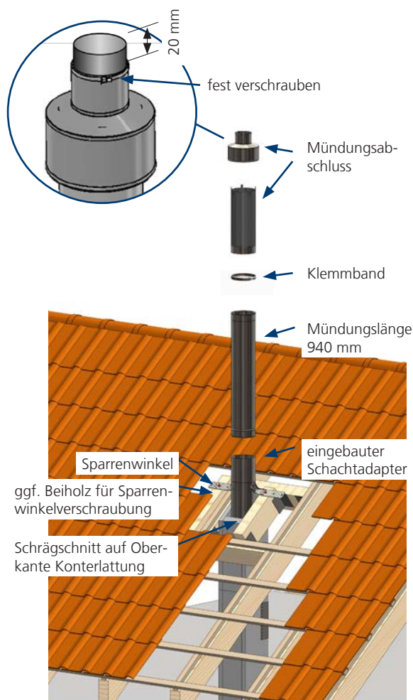
Abb. 37: Dachhochführung bei PolyCase DN 60 bis 100
