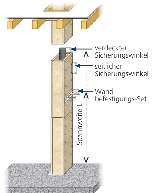
Abb. 15: Spannweiten seittl. Führungen
