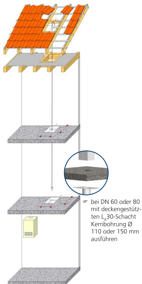
Abb. 18: Decken- und Dachdurchbrüche ausloten
