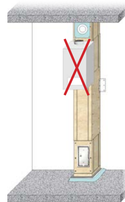
Abb. 46: Heizgeräte nicht direkt an den Schacht anbauen
