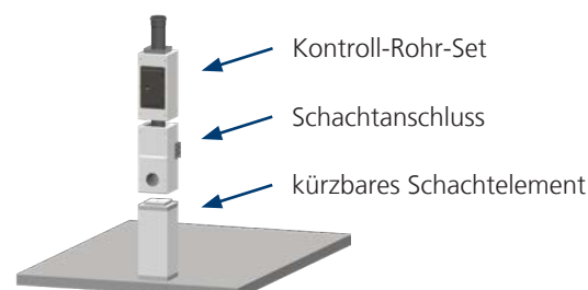
Abb. 4: bodengestützte PolyCase-Abgasanlage mit Schutzziel L A 90
