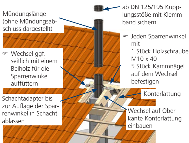
Abb. 35: Schachtheadapter auf der Sparrenkonstruktion verschrauben
