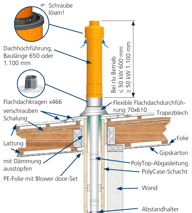
Abb. 42: Schnitt Dachdurchführung DN 60/100 - 100/150
