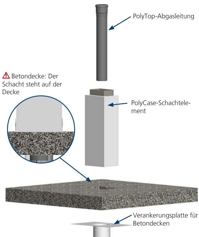
Abb. 19: Deckengestützter Anschluss in DN 60/100, 80/125, 100/150 oder 110/160
