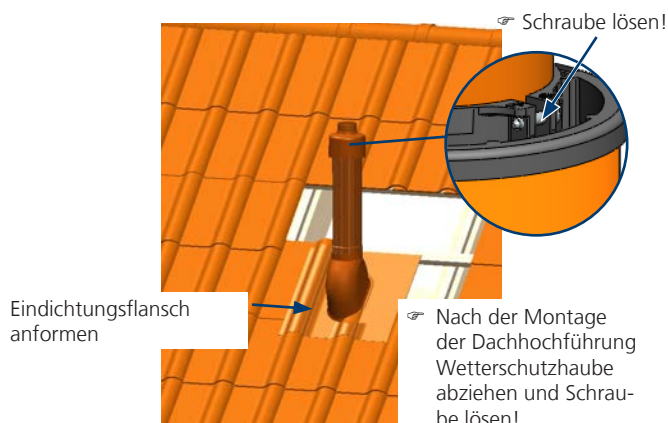
Abb. 38: Fertige Abgasanlagen-Mündung bei PolyCase DN 60 bis 100
