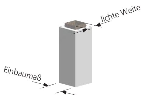
Abb. 1: Hauptabmessungen
