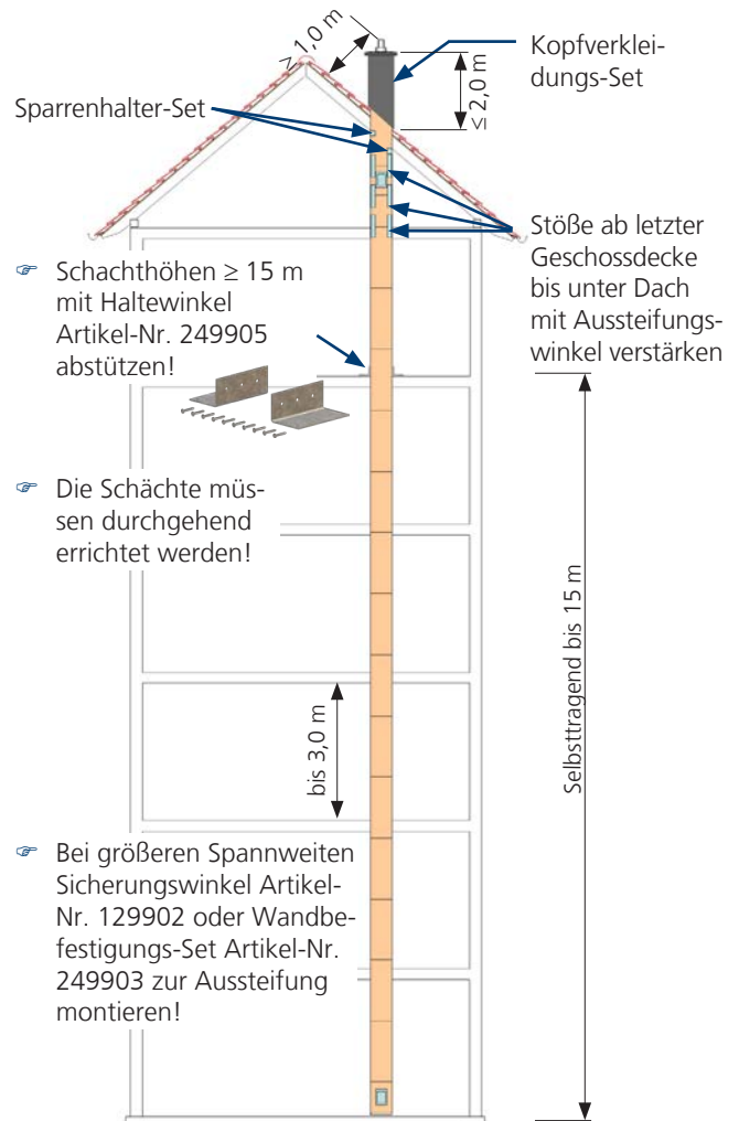
Abb. 12: Statik
