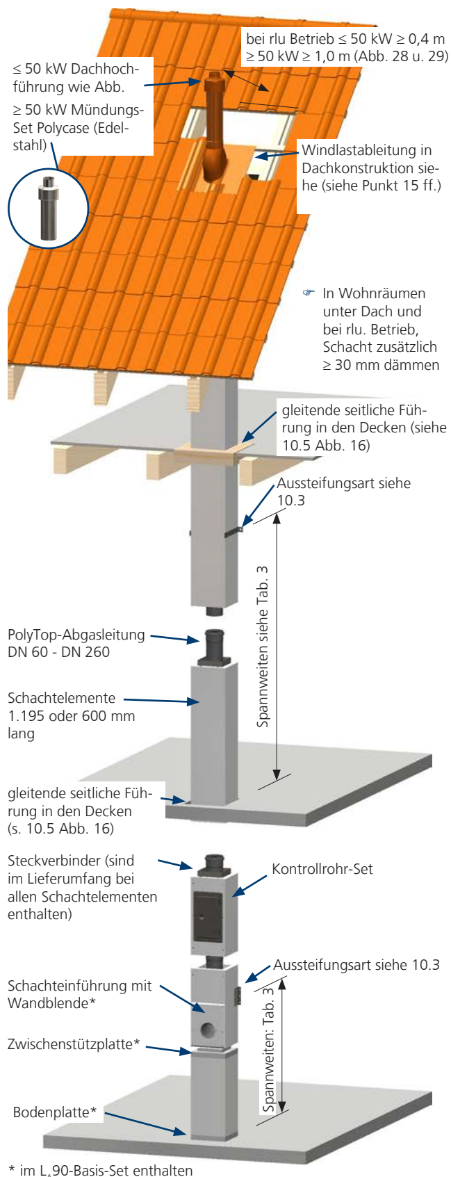
Abb. 17: typische einfachbelegte Abgasanlage
