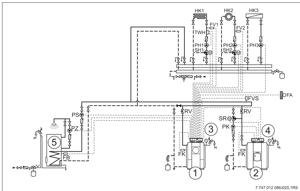
Bild 17 Hydraulik 4
