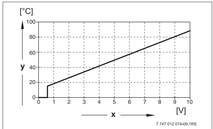
Bild 25 Eingang 0 – 10 V
