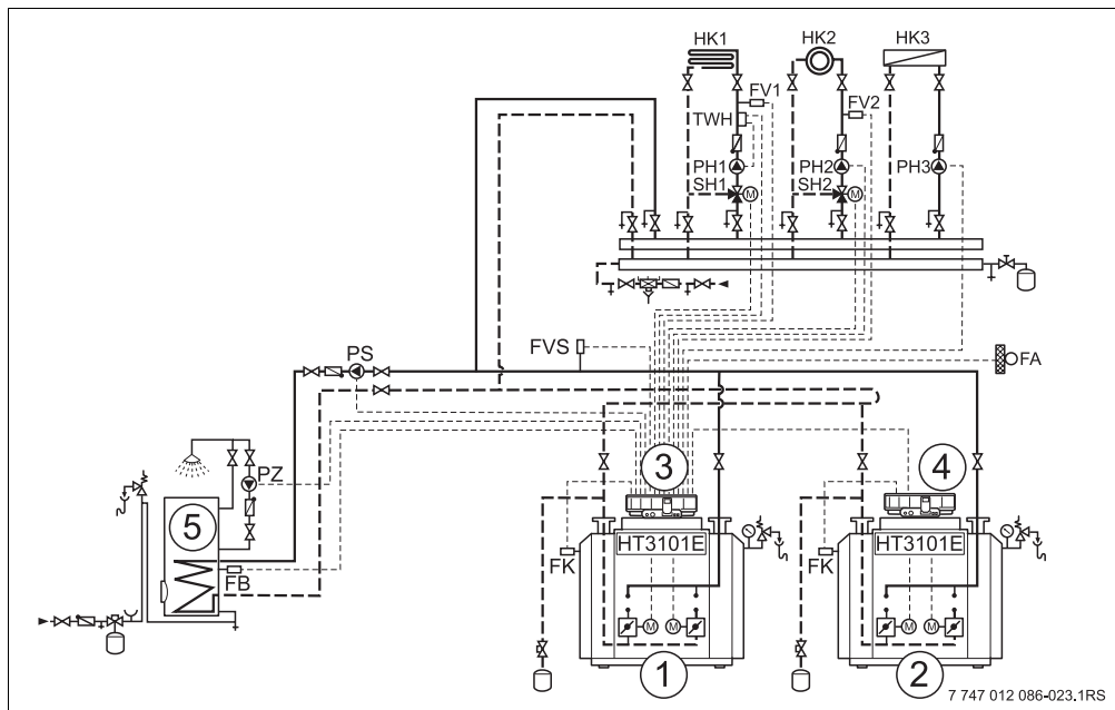
Bild 20 Hydraulik 7
