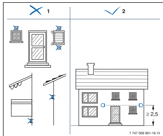
Bild 17 Anordnung des Außentemperaturfühlers, Beispiele (Maße in m)
