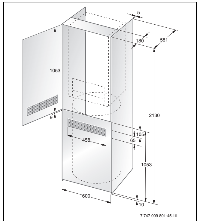
Bild 45 Buderus-Umbauschrank V 60 zur Installation einer Gas-Wärmezentrale mit Logamax U152/ U154 und Warmwasserspeicher Logalux HC70 W, HC110 W oder S120 W untereinander (Maße in mm)
