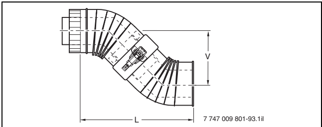
Bild 93 Versatzmaße konzentrischer Bogen (→ Tabelle 42)
