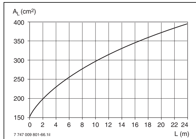
Bild 66 Querschnitt einer Verbrennungsluftleitung bzw. eines Verbrennungsluftschachts in Abhängigkeit von der Leitungs- bzw. Schachtlänge (Variante bei Rauminhalt > 1 \text{ m}^3 je 1 kW Gesamt-Nennwärmeleistung)
