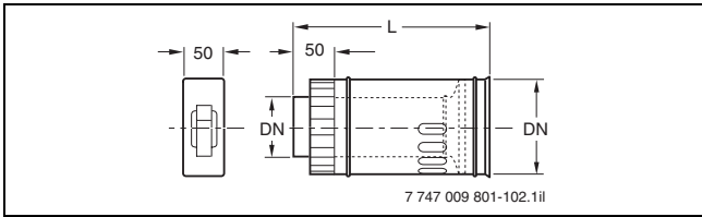
Bild 102 Zuluftgitter für Bausatz GA-X (Maße in mm, → Tabelle 45)
