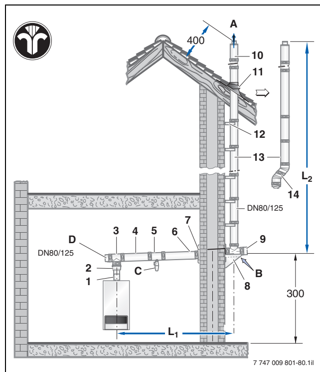
Bild 80 Montagevariante mit dem Bausatz GAF-K für U152 (Maße in mm); maximal zulässige gestreckte Baulänge L der Abgasleitung → Tabelle 30, Bauteile → Seite 88
