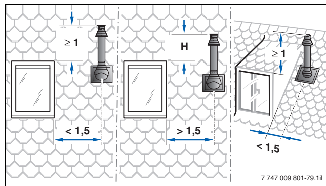
Bild 79 Beispiele für Mindestabstände zu Fenstern beim Bausatz DO nach Muster-Feuerungsverordnung; zusätzlich jeweilige Landesbauordnung beachten (Maße in m)
