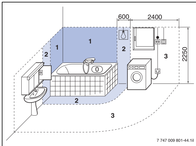
Bild 44 Elektrische Schutzbereiche nach VDE 0100 (Maße in mm)
