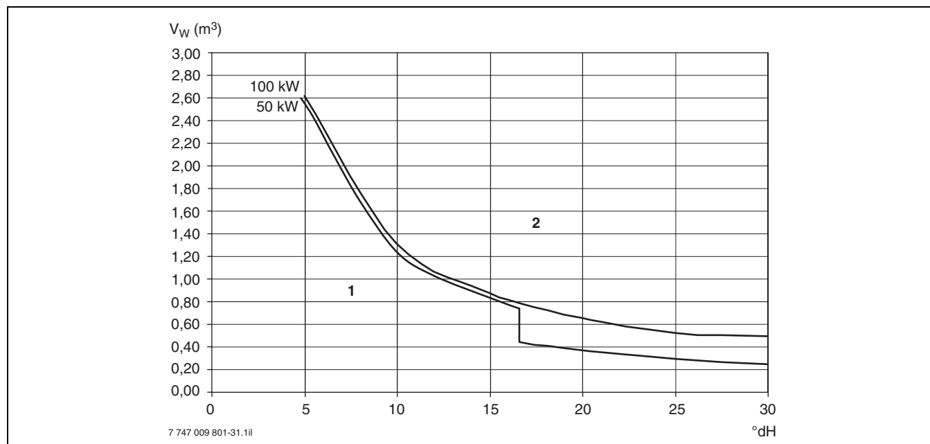
Bild 31 Grenzen zur Wasserbehandlung bei 1-Kessel-Anlagen
