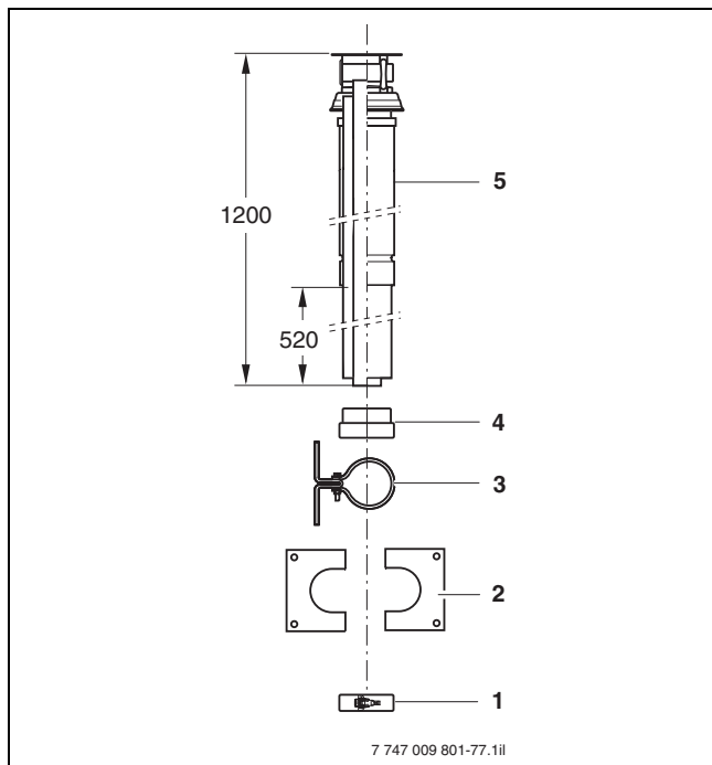
Bild 77 Bauteile des Grundbausatzes DO für U152 (Maße in mm)
