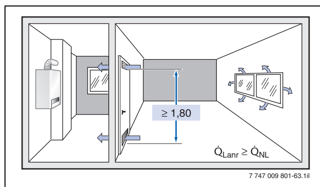
Bild 63 Unmittelbarer Verbrennungsluftverbund (Maße in m)
