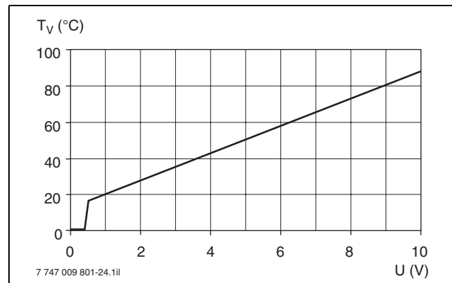
Bild 25 Kennlinie Störmeldemodul EM10 (Sollwerte)
