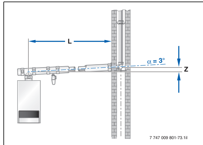
Bild 73 Gefälle ( \alpha = 3^\circ ) zum problemlosen Ableiten von Kondenswasser aus der Abgasleitung (Maße \rightarrow Tabelle 26)
