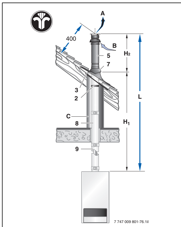
Bild 76 Montagevarianten mit dem Bausatz DO für U152 (Maße in mm, → Tabelle 28; maximal zulässige gestreckte Baulänge L der Abgasleitung → Tabelle 27, Bauteile → Seite 85 f.
