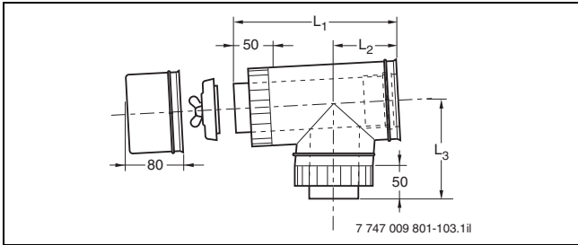
Bild 103 Konzentrisches Inspektions-T-Stück (Maße in mm, → Tabelle 46)
