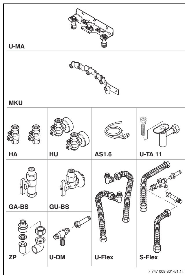
Bild 51 Anschlusszubehör für Logamax U152/U154 mit unten- oder nebenstehendem Warmwasserspeicher
