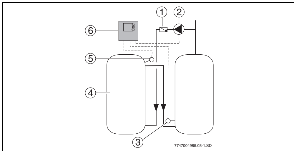
Bild 4 Umschichtfunktion
