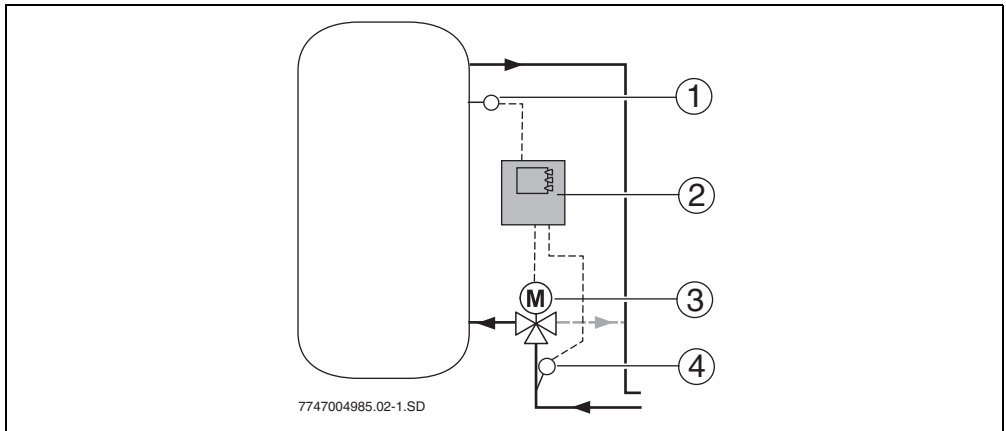
Bild 3 Rücklaufanhebung
