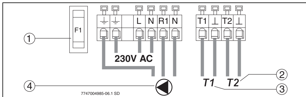
Bild 9 Anschlussplan
