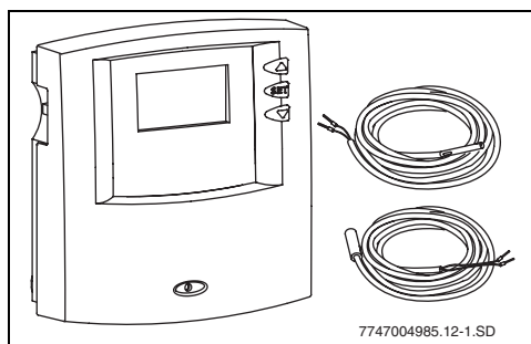
Bild 1 Regler SC10 mit Temperaturfühlern
