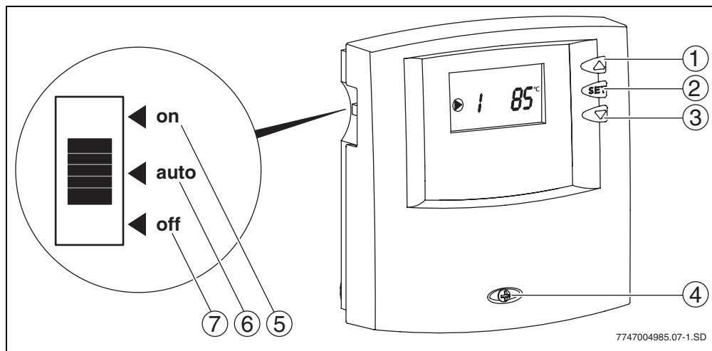
Bild 11 Regler und Handschalter
