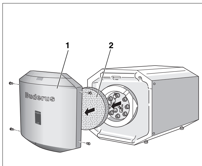
Abb. 8 Vorderwand und Wärmeschutz abnehmen
