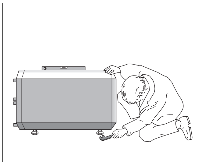
Abb. 6 Warmwasserspeicher ausrichten (Prinzipabbildung) mit Hilfe einer Wasserwaage
