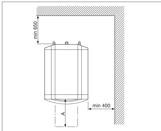
Abb. 5 Warmwasserspeicher aufstellen (Prinzipabbildung)
