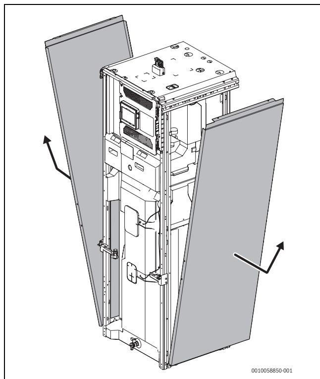
Bild 17 Seitenwand
