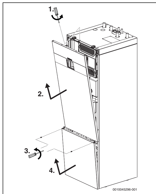
Bild 20 Demontage der Frontseite
