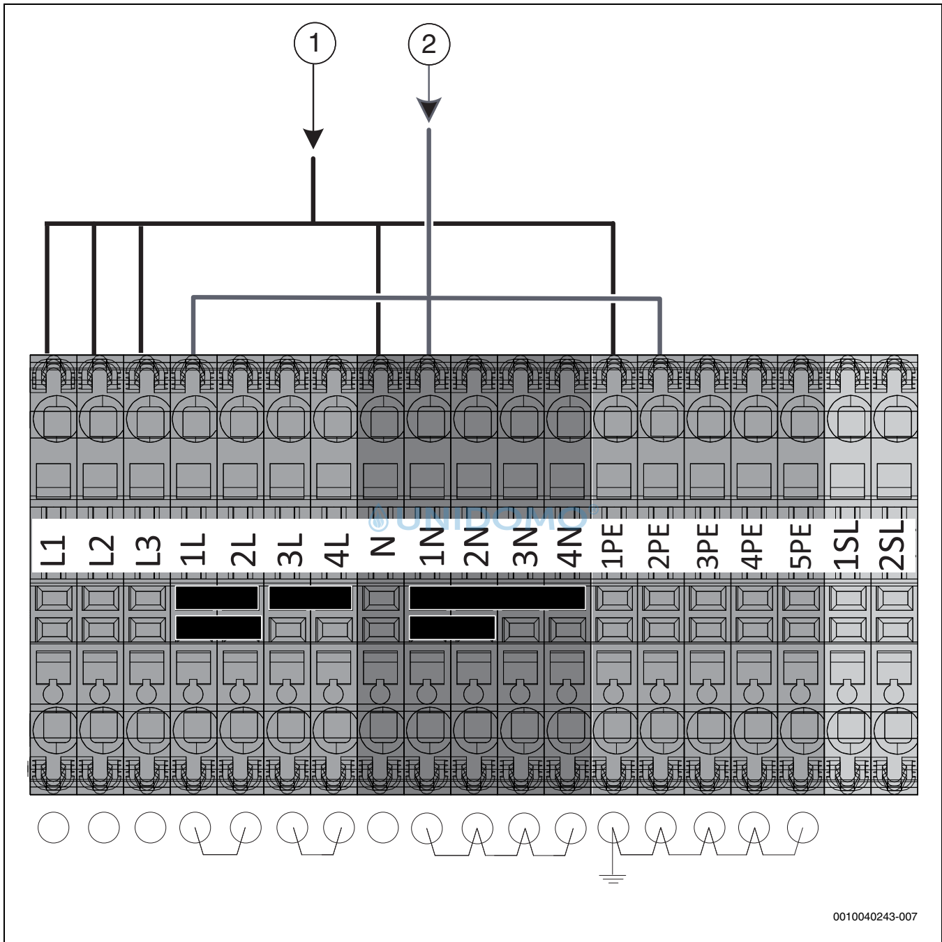
Bild 43 Elektrische Anschlüsse mit EVU-Sperre
