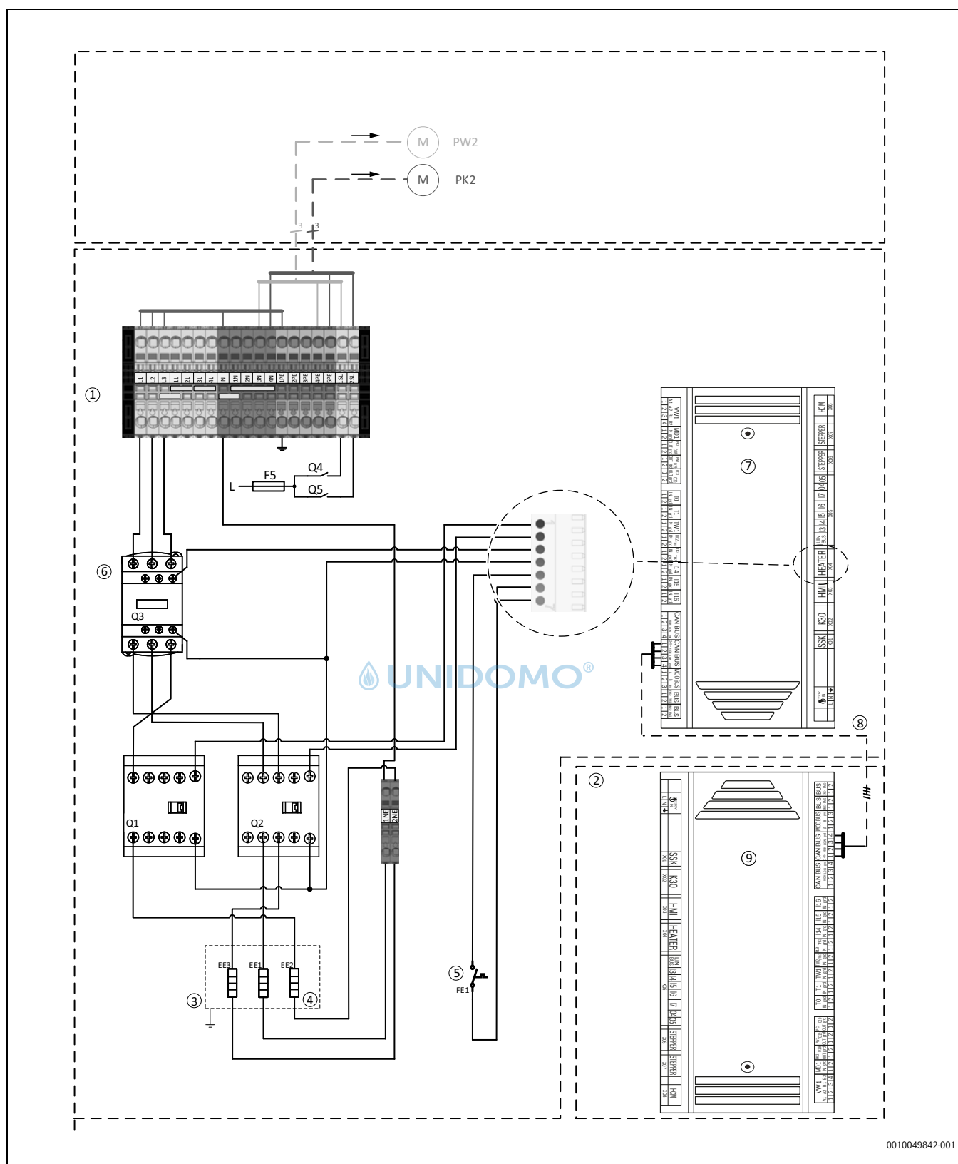
Bild 59 Spannungsversorgung Inneneinheit
