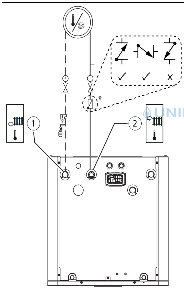
Bild 27 Heizungsanlagenanschlüsse der Inneneinheit
