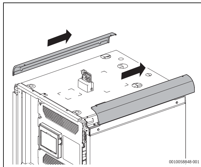
Bild 15 Abdeckleisten
