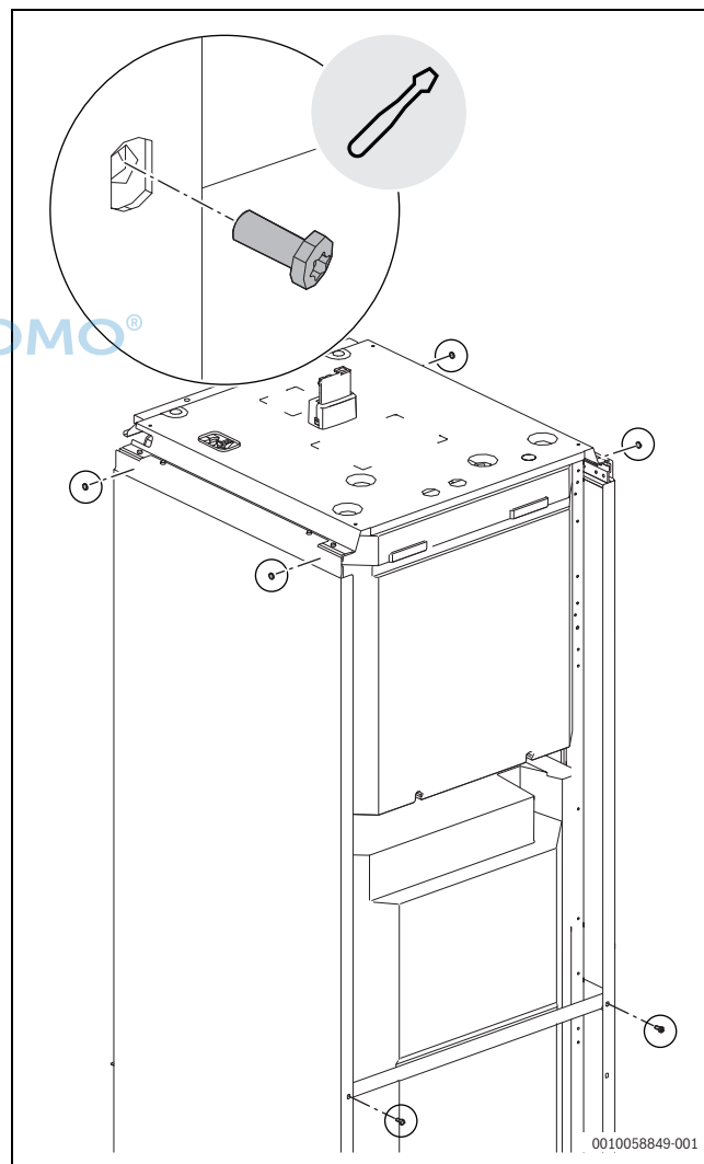
Bild 16 Schrauben für die Seitenwände
