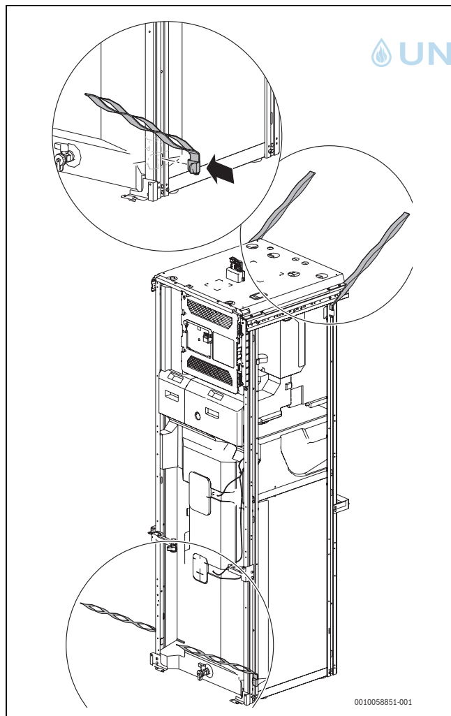
Bild 18 Transportgurte
