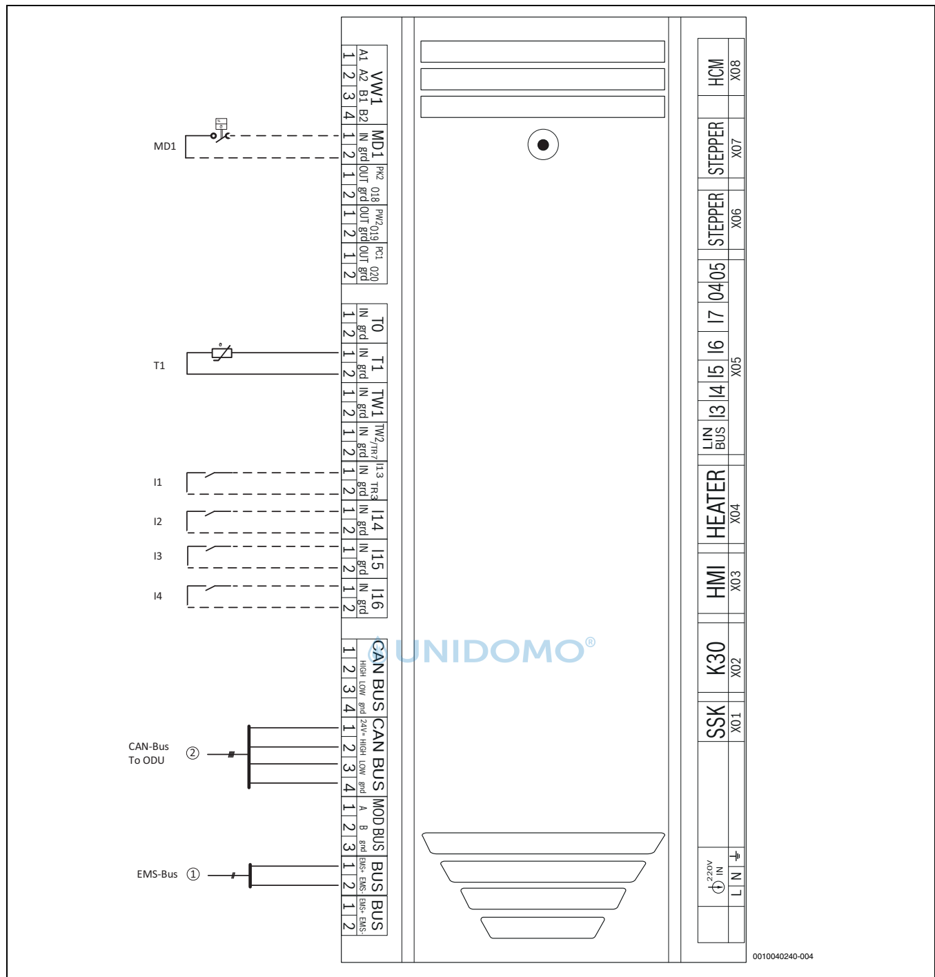
Bild 45 Anschlüsse XCU-THH (XCU HY)
