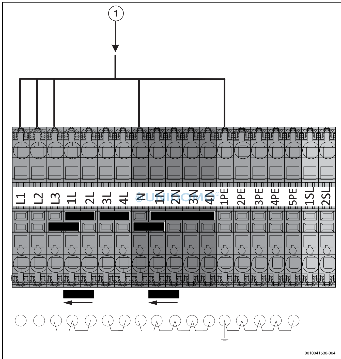
Bild 41 Elektrische Anschlüsse ohne EVU-Sperre
