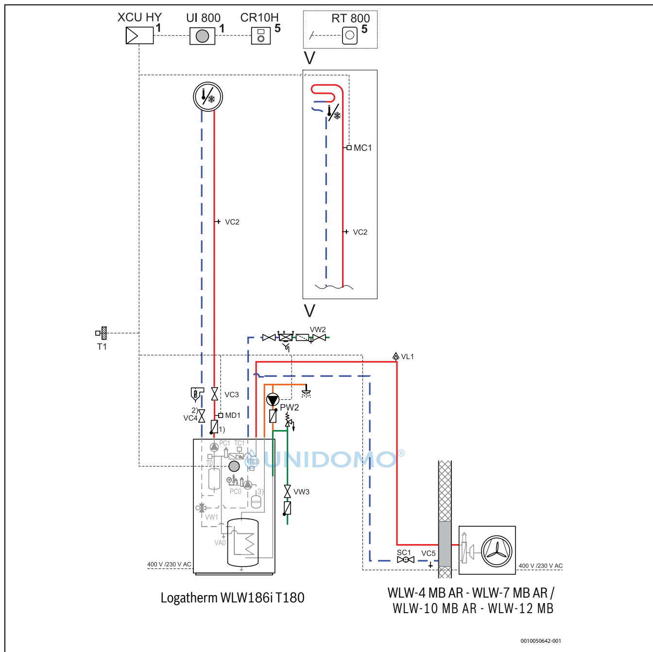
Bild 54 Tower Inneneinheit, Wärmepumpe (ODU), ein ungemischter Heizkreis (nur für Polen)
