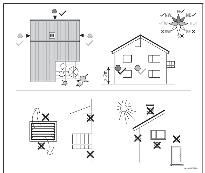
Bild 36 Position des Außentemperaturfühlers
