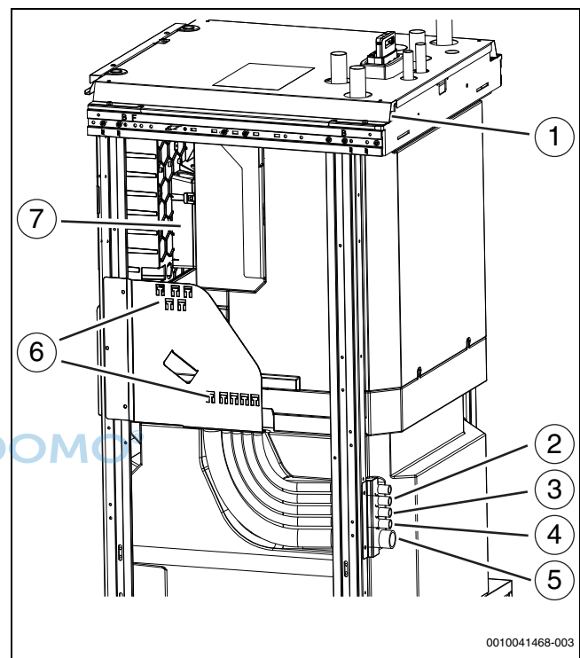
Bild 38 Kabeleinführungen der Inneneinheit
