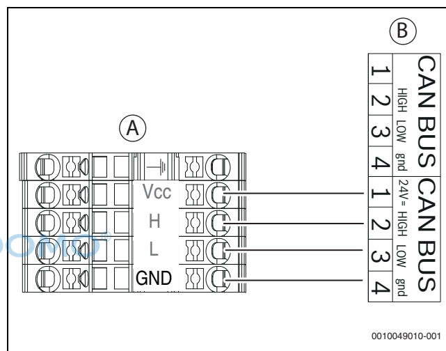
Bild 33 CAN-BUS Wärmepumpe - Inneneinheit
