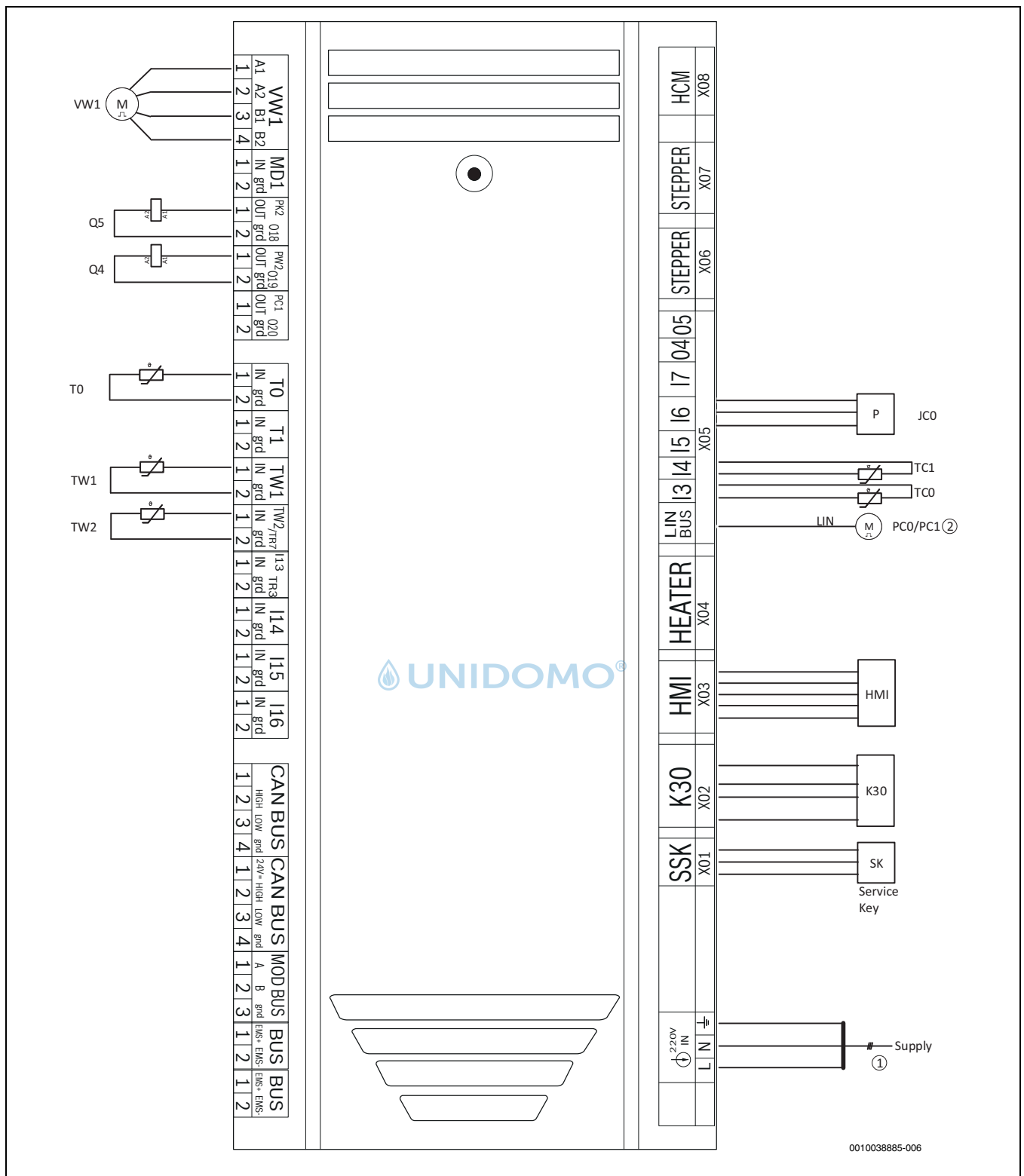
Bild 57 Schaltplan XCU-THH (XCU HY)-Modul
