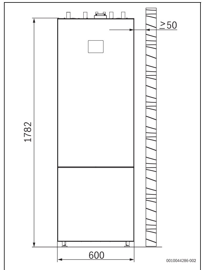
Bild 3 Abmessungen (mm)
