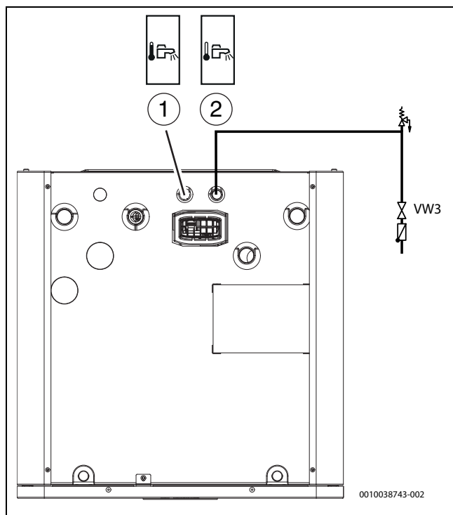
Bild 29 Wärmepumpenanschlüsse Trinkwasser
