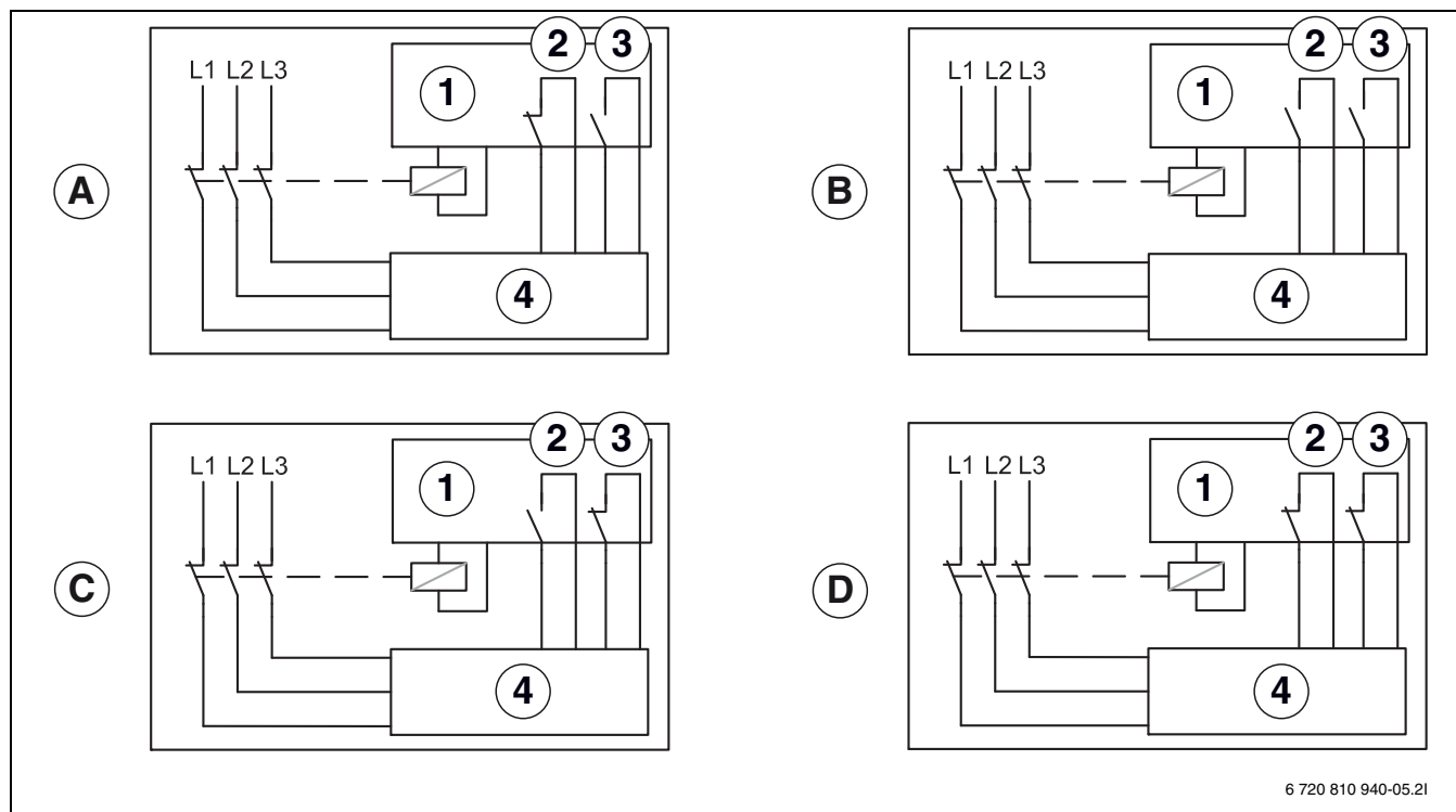
Bild 47 Anschlussplan für EVU-Sperre/SG
