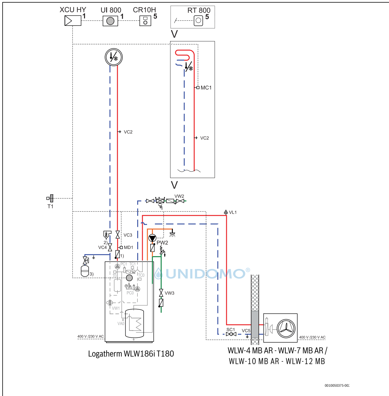
Bild 55 Tower Inneneinheit, Wärmepumpe (ODU) und ein ungemischter Heizkreis (für Deutschland, Österreich, Schweiz)
