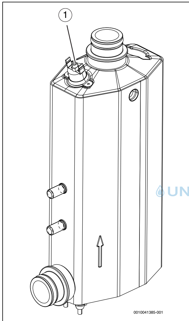
Bild 50 Elektrischer Zuheizer
