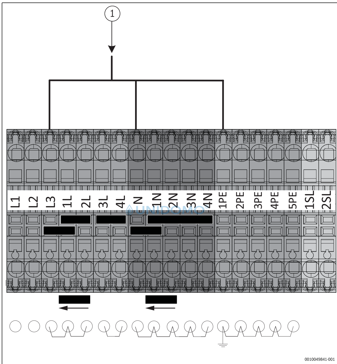
Bild 42 Elektrischer Anschluss, einphasig, nur 3 kW
