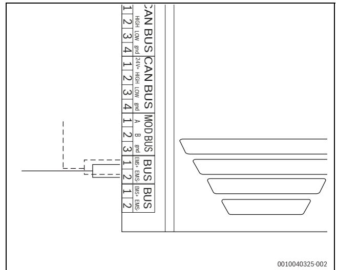
Bild 35 EMS-Anschluss
