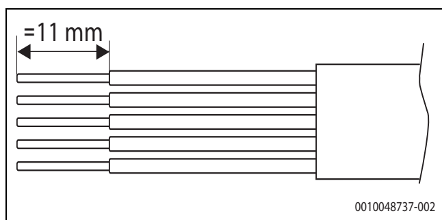
Bild 37 Abisolieren der Adern für den Netzanschluss
