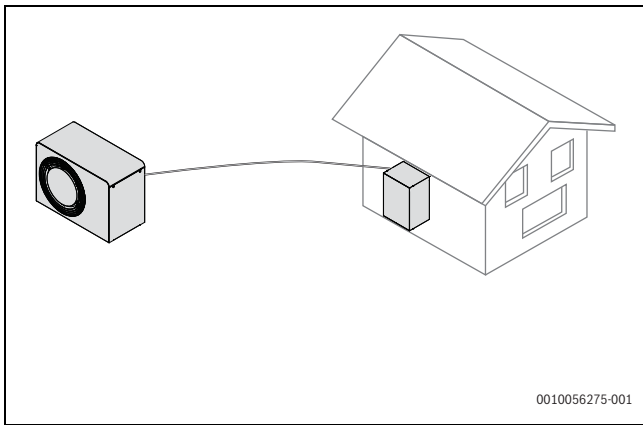
Bild 34 CAN-BUS-Verbindung zwischen Innen- und Außeneinheit
