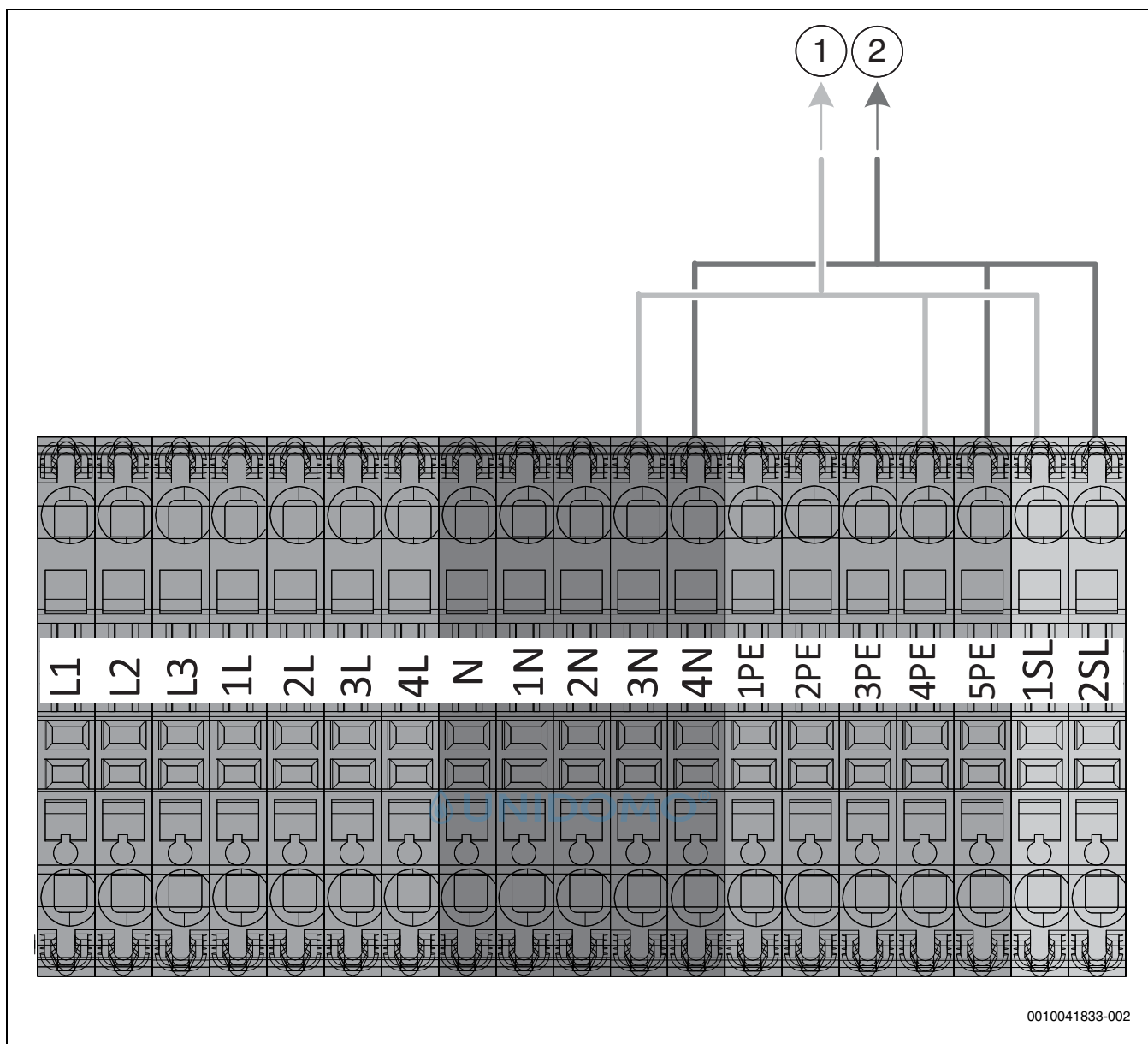
Bild 44 Elektrische Anschlüsse für Zubehör
