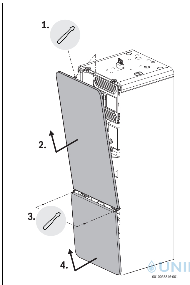
Bild 13 Vorderwand
