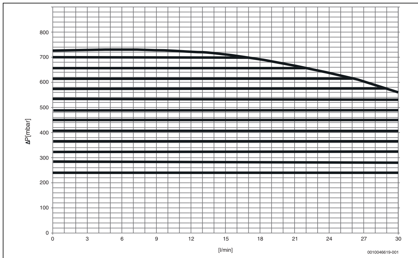
Bild 56 Pumpenkennzahlen für PC1
