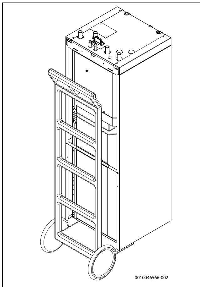
Bild 11 Transportwagen mit Gerät
