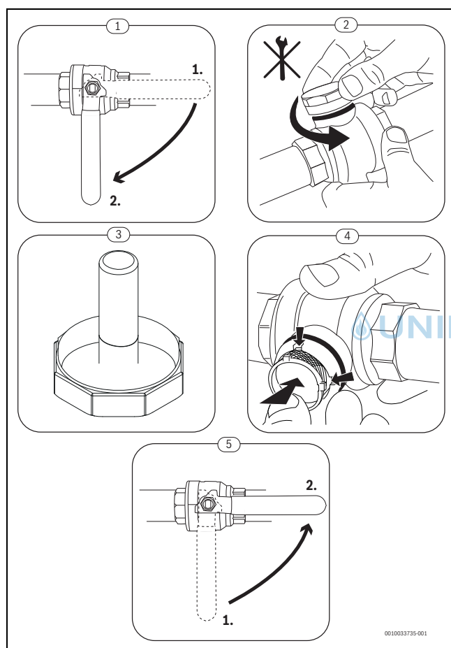
Bild 51 Reinigen des Partikelfilters
