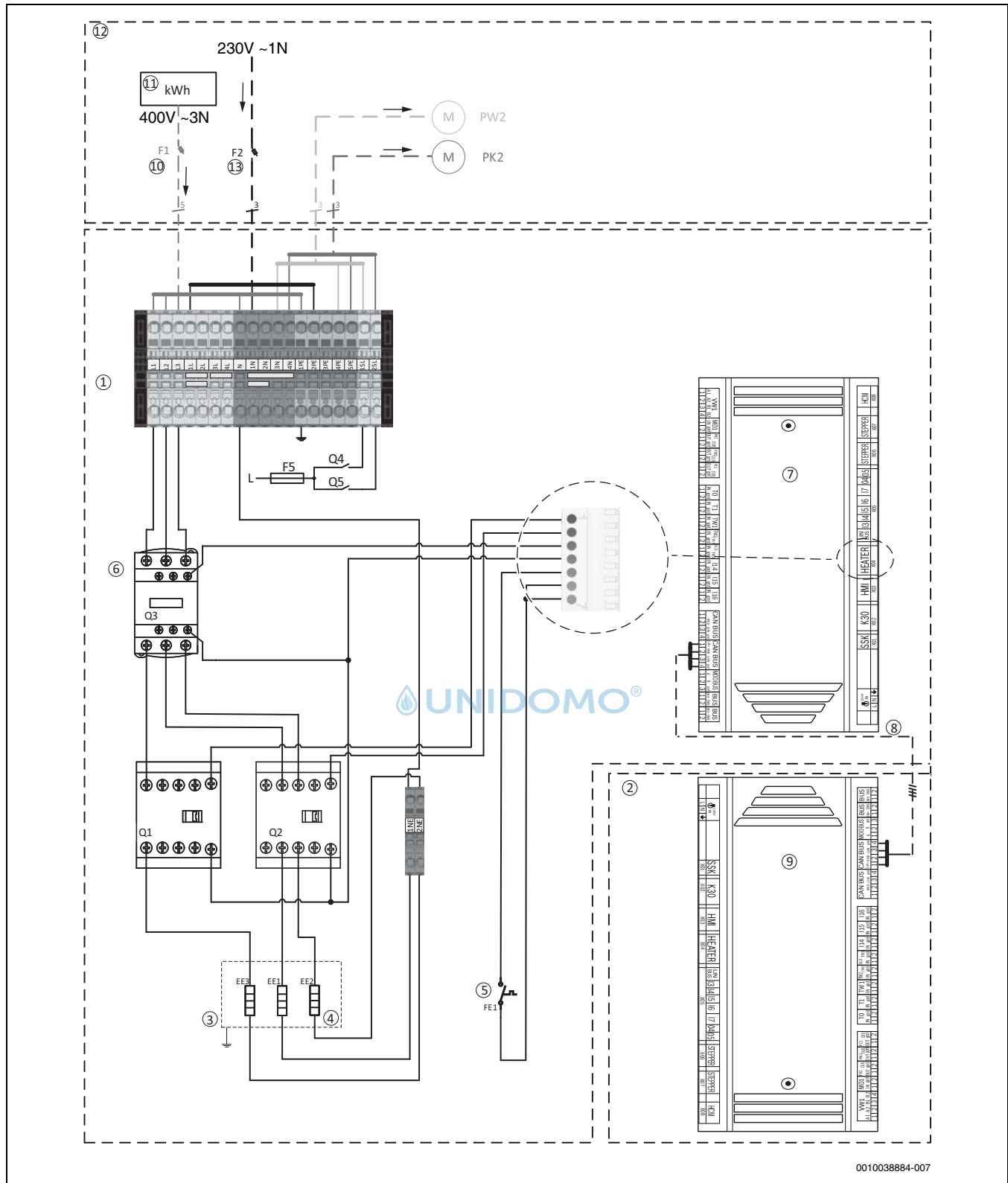
Bild 58 Spannungsversorgung Inneneinheit
