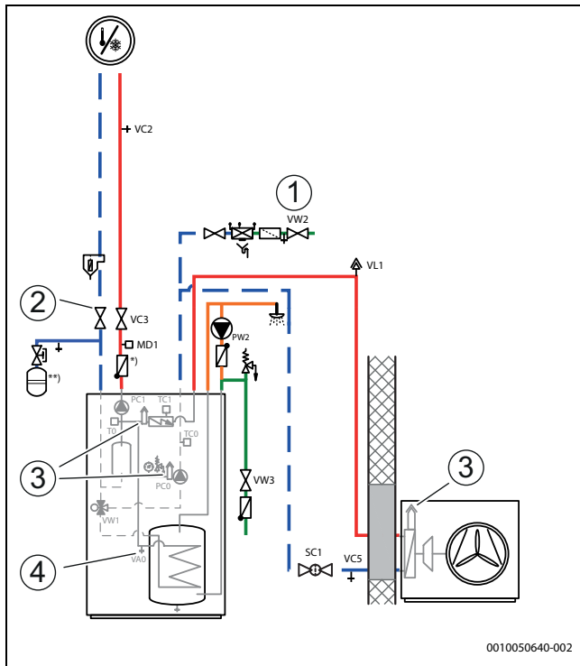
Bild 31 Inneneinheit, Wärmepumpe und Heizungsanlage (für Deutschland, Österreich, Schweiz)
