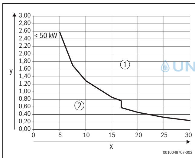
Bild 7 Wärmeerzeuger < 50 kW - 100 kW
