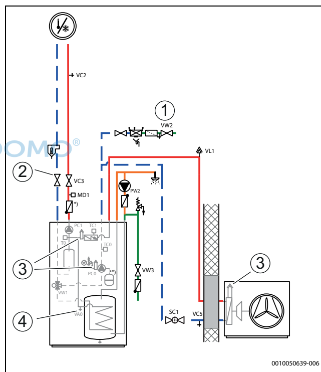
Bild 30 Inneneinheit, Wärmepumpe und Heizungsanlage (nur für Polen)
