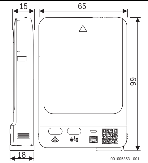
Bild 6 Abmessungen in mm
