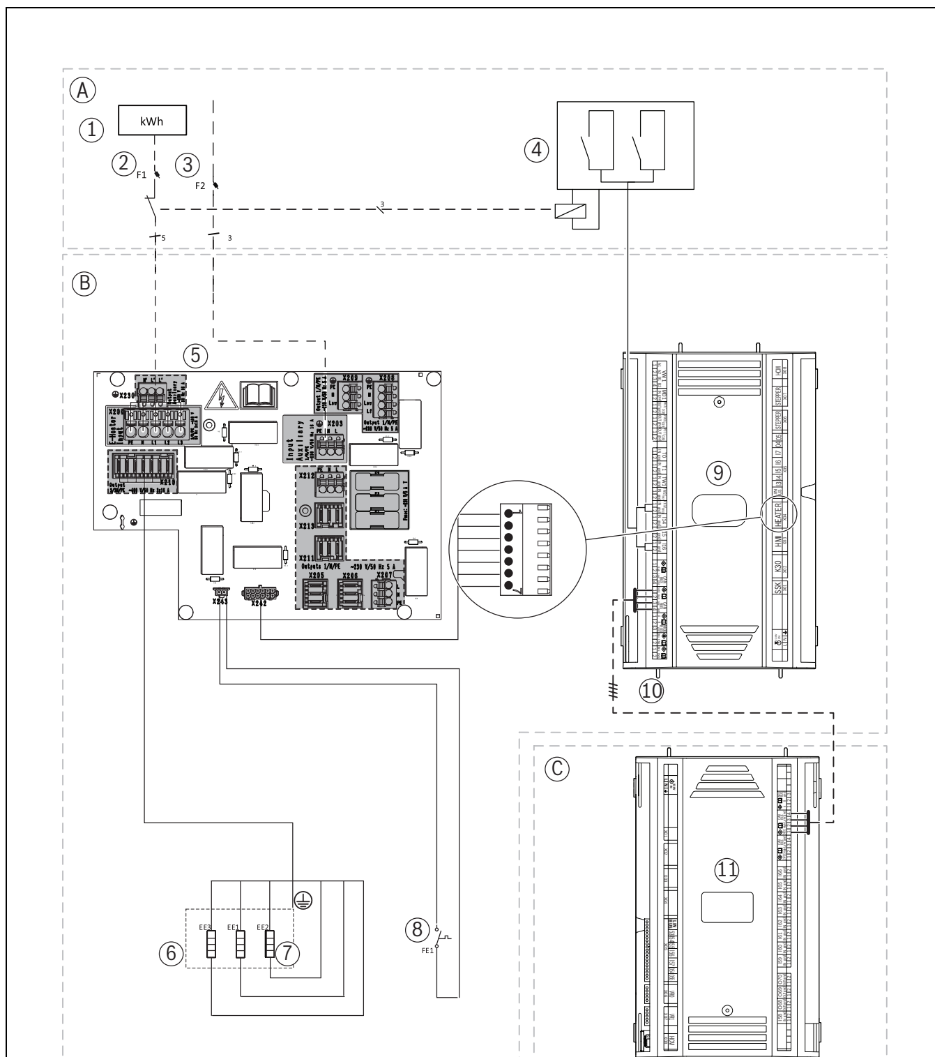
Bild 54 Spannungsversorgung Inneneinheit
