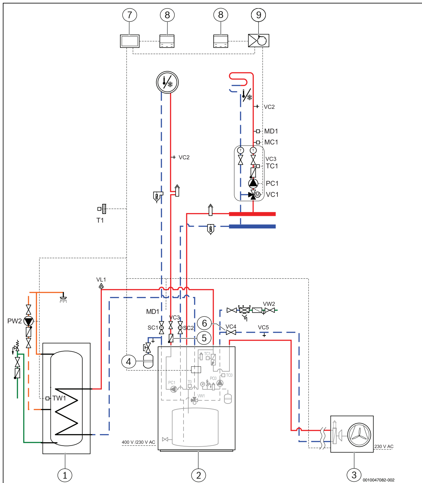
Bild 58 Anlagenlösung mit Außeneinheit, Inneneinheit mit integriertem Zuheizer und Pufferspeicher, einem ungemischten und einem gemischten Heizkreis
