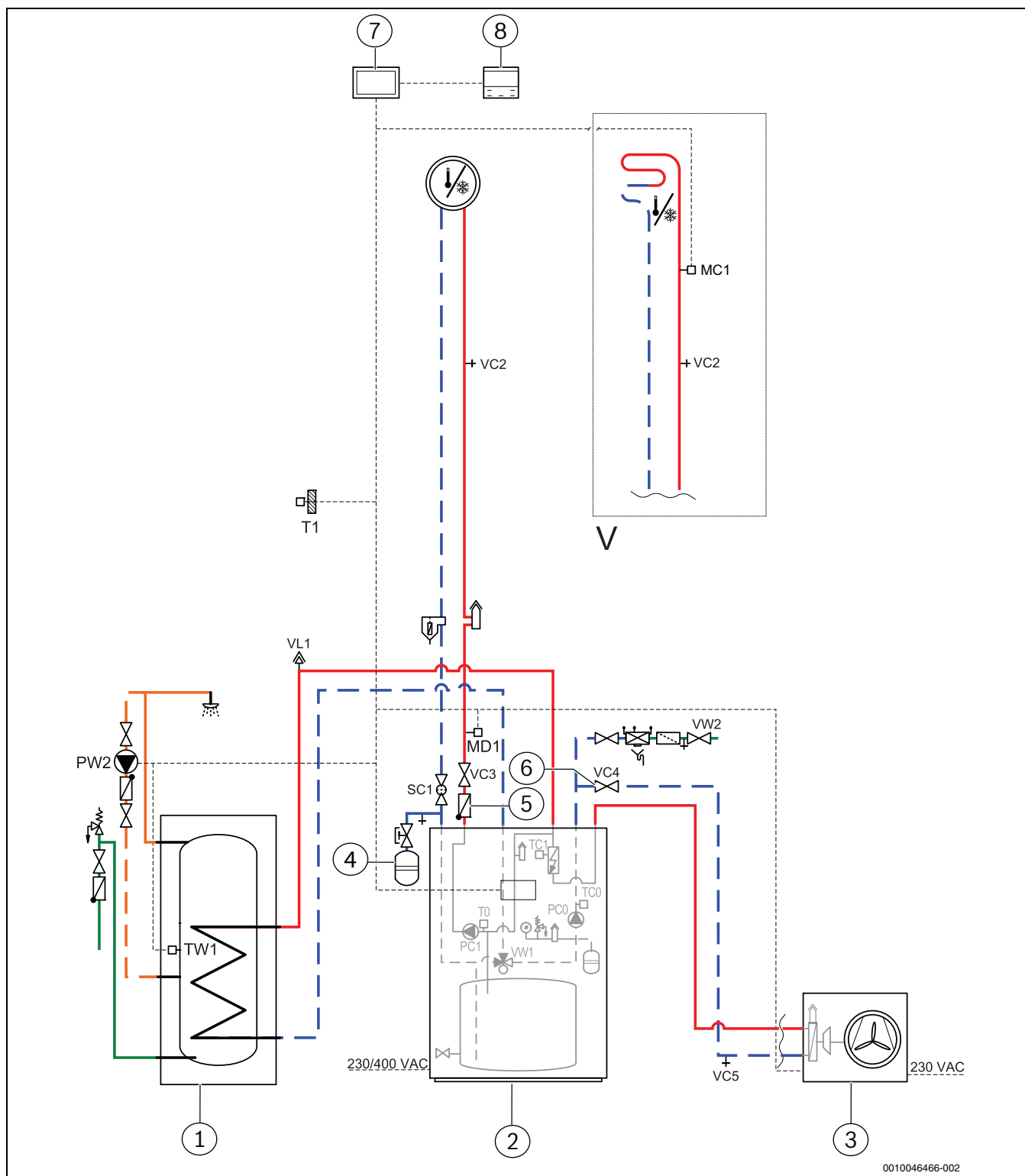
Bild 57 Anlagenlösung mit Außeneinheit, Inneneinheit mit integriertem Zuheiz- und Pufferspeicher und einem ungemischten Heizkreis
